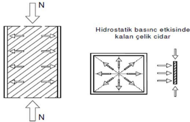
Şekil 3.3 : Eksenel Basınç Yüğü Altında Kalan CFT Elemanın Çelik Cidarına Etkiyen Kuvvetler.
