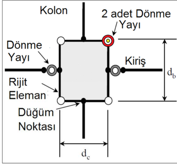
Şekil 4.10 : Gupta ve Krawinkler Tarafından Önerilen Panel Bölgesi Modeli.
