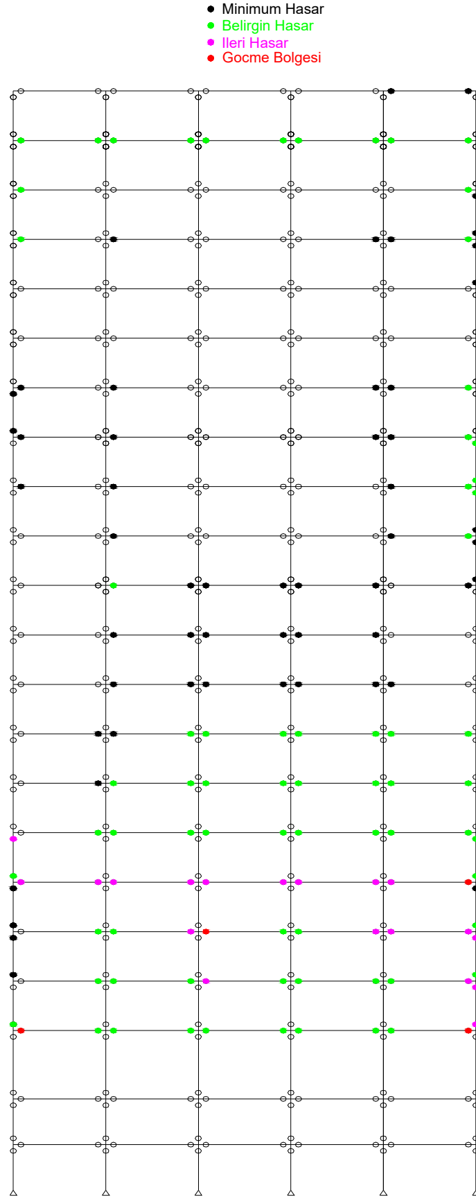
Şekil 5.13 : 7 Aksı Kesit Hasar Seviyeleri.
