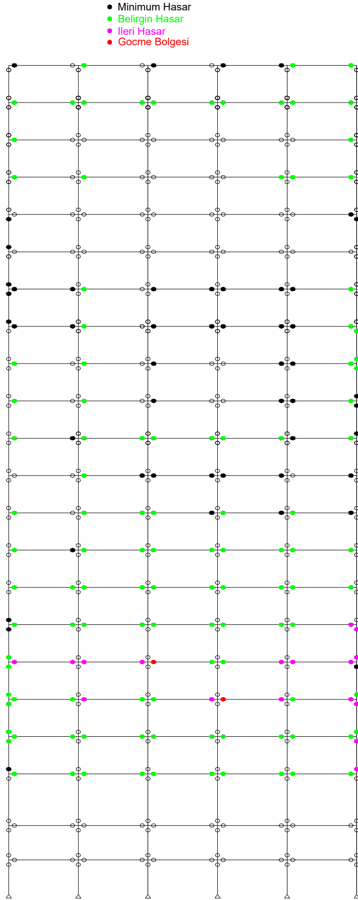
Şekil 5.8 : 7 Aksı Kesit Hasar Seviyeleri.
