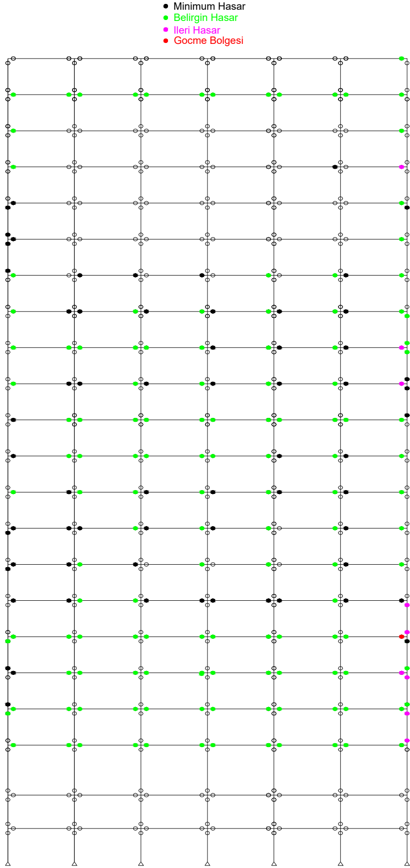
Şekil 5.9 : A Aksı Kesit Hasar Seviyeleri.
