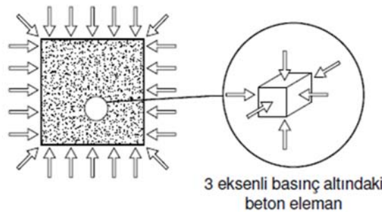
Şekil 3.4 : Eksenel Basınç Yüğü Altında Kalan CFT Elemanın Çelik Cidarına Etkiyen 3 Eksenli Kuvvetler.
