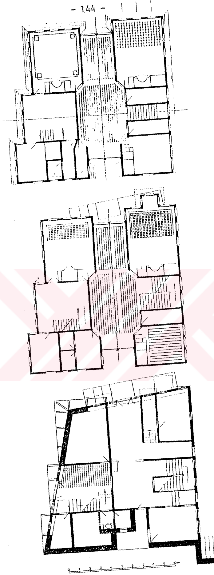
Şekil 5.6. Üsküdar, Selimiye Kavak Bayırı'ndaki Ev, Zemin Kat, I. Kat ve II. Kat Plânları.
