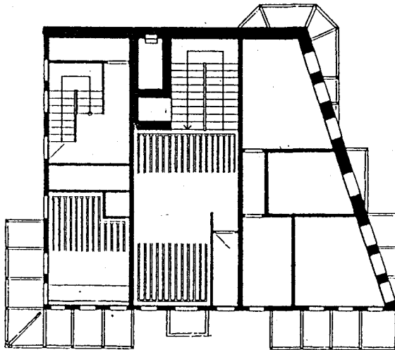
Şekil 5.5. Cihangir Cami Yanındaki Ev, Giriş Cephesi ve Kat Plânları Restitüsyonu.
