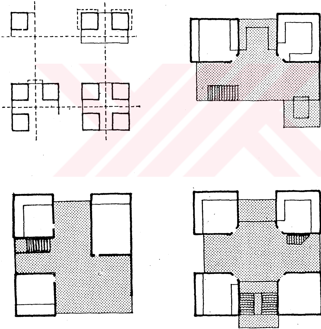
Şekil 1.2.2. Doğan Kuban'ın "Türk Evi Plânlamasındaki İşlevsel Birim ve Çoğalımı" Şeması.
