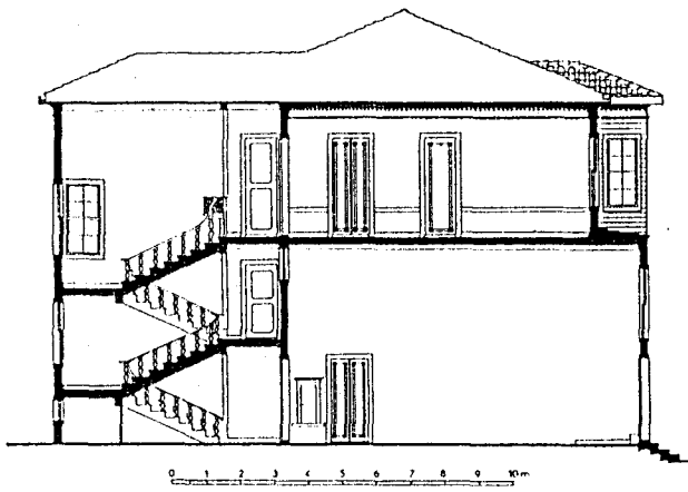
Şekil 5.1. . İstanbul Agâh Efendi Konağı, Zemin ve I.Kat Planları, Kesit ve Cephe Restitüsyonları
