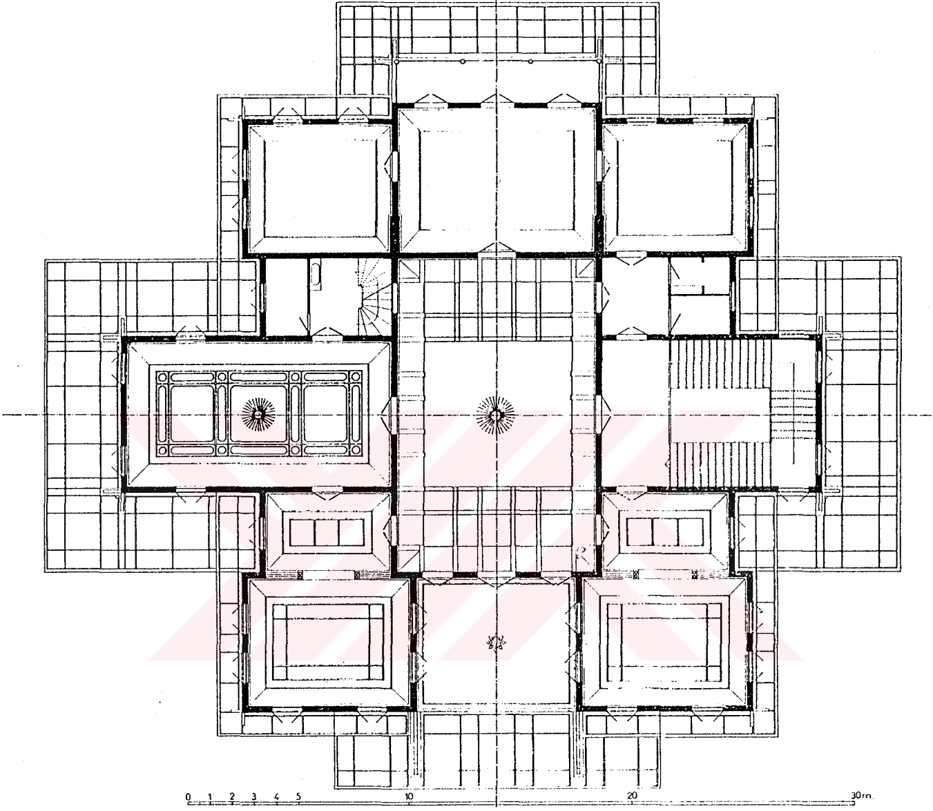
Şekil 5.4. Bağlarbaşı Mecid Efendi Konağı, I.Kat Restitüsyon Planı
