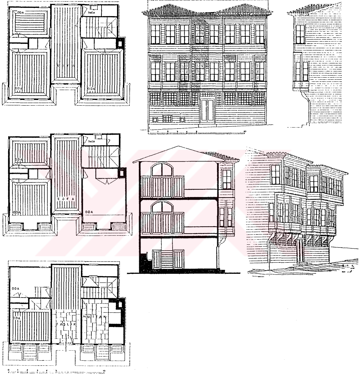
Şekil 5.2. Bağlarbaşı Selamsız'da Bir Konak, Kat Planları, Kesit ve Cephe Restitüsyonları
