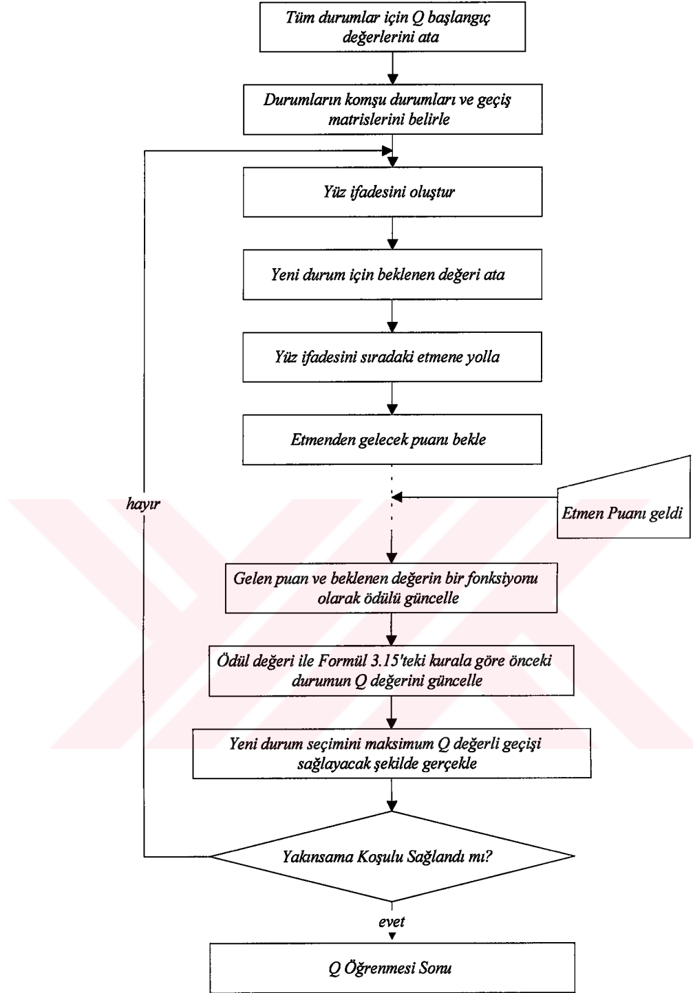
Şekil 7.13 Öğrenme Süreci Yürütme Adımları
