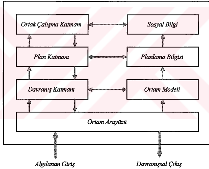
řekil 2.6 Interrap Mimarisi
