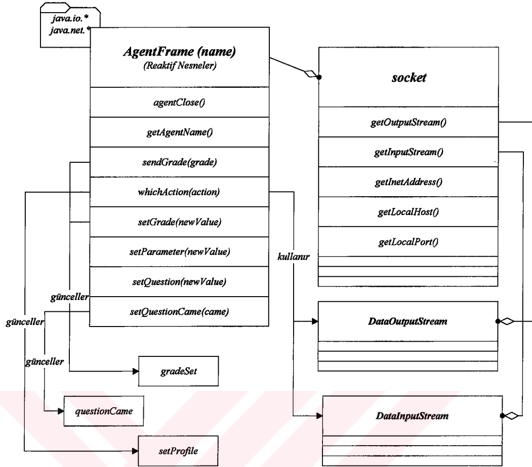
Şekil 8.7 AgentFrame Sınıf Hiyerarşisi
