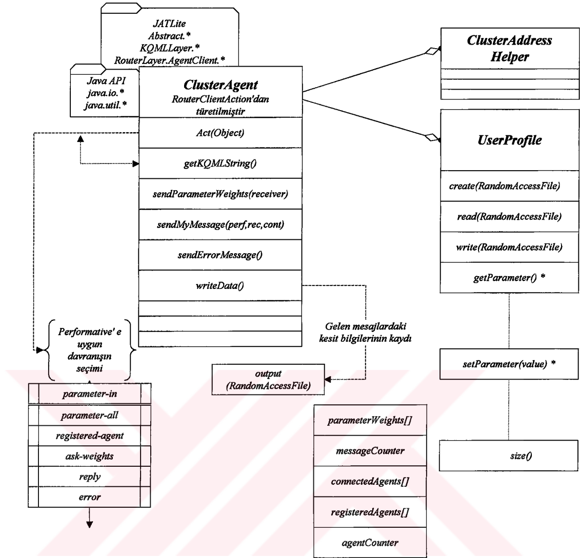
Şekil 8.10 ClusterAgent Sınıf Hiyerarşisi
