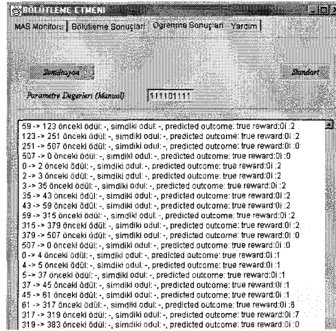
Şekil 9.8 “Öğrenme Sonuçları” Menüsü (Bölütleme Etmeni)
