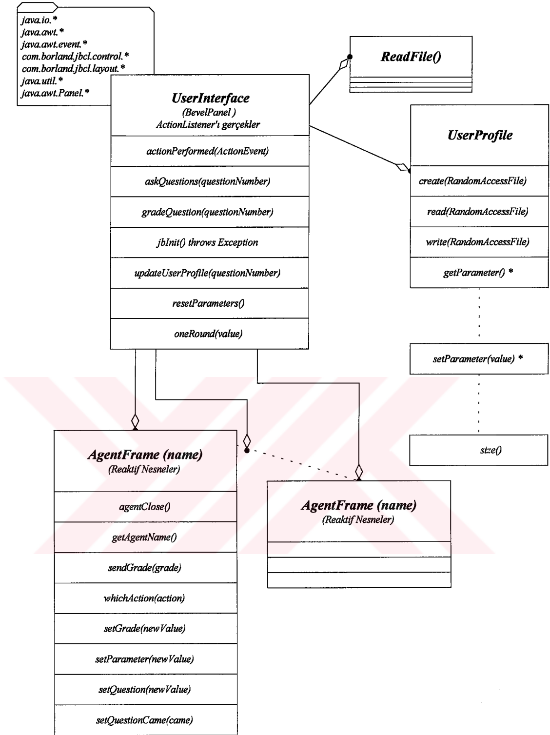
 ekil 8.6 UserInterface Sınıf Hiyerar isi
