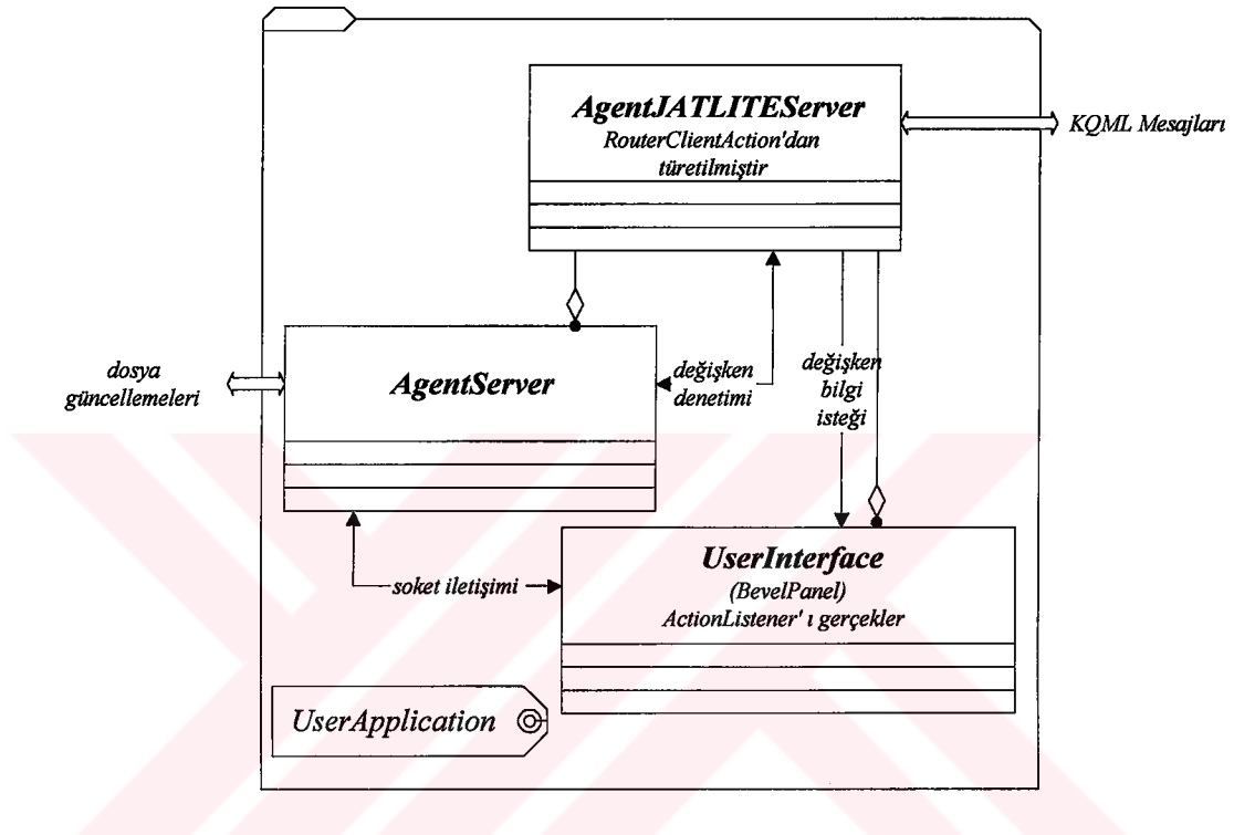
Şekil 8.2 UserApplication Sınıfı ve Alt Bileşenleri
