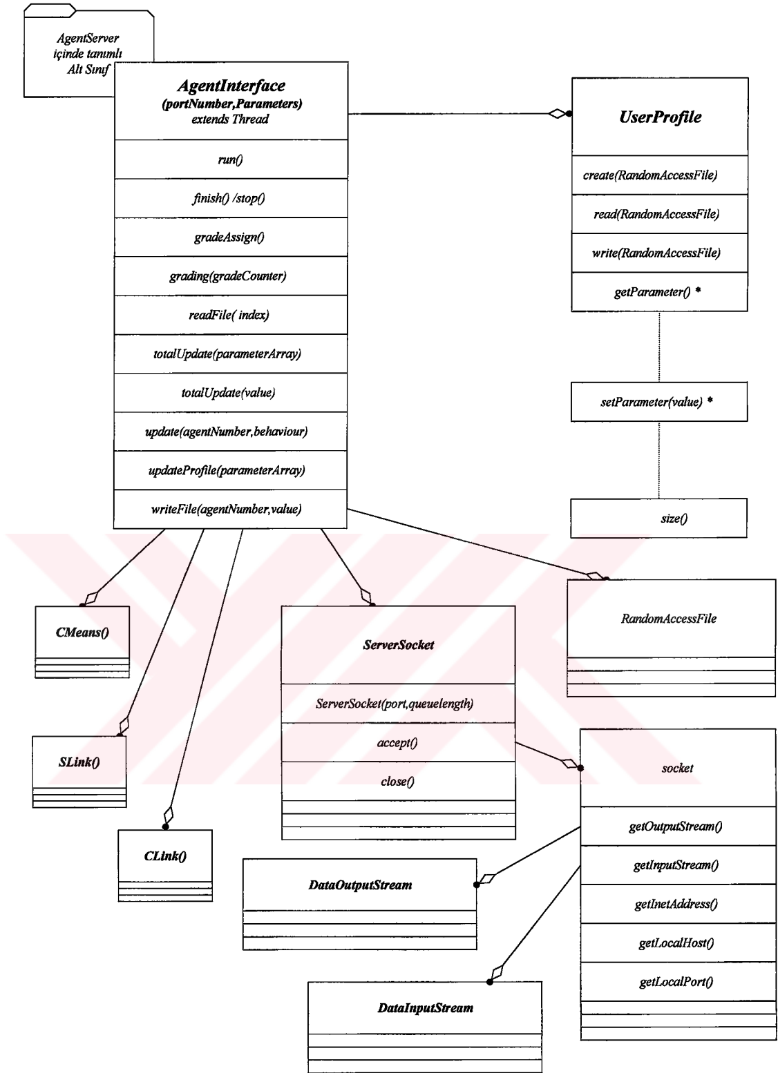
Şekil 8.5 AgentInterface Sınıf Hiyerarşisi
