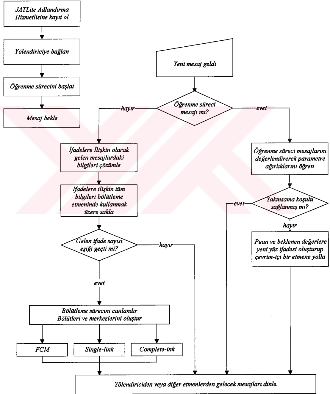
Şekil 7.12 Bölütleme Etmeni Yaşam Çevrimi
