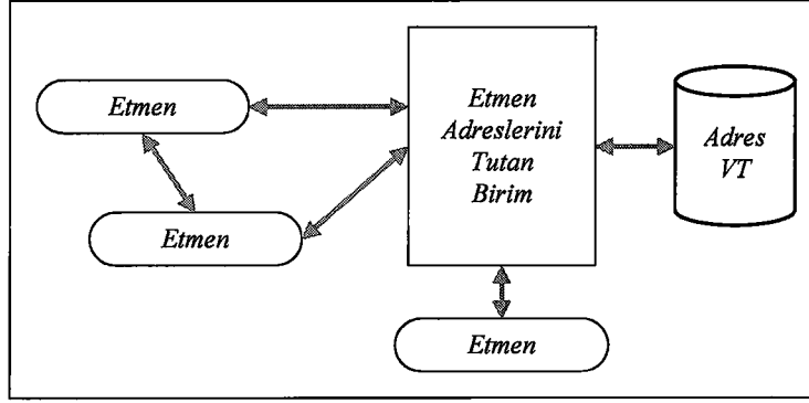
Şekil 2.3 Doğrudan İletişim
