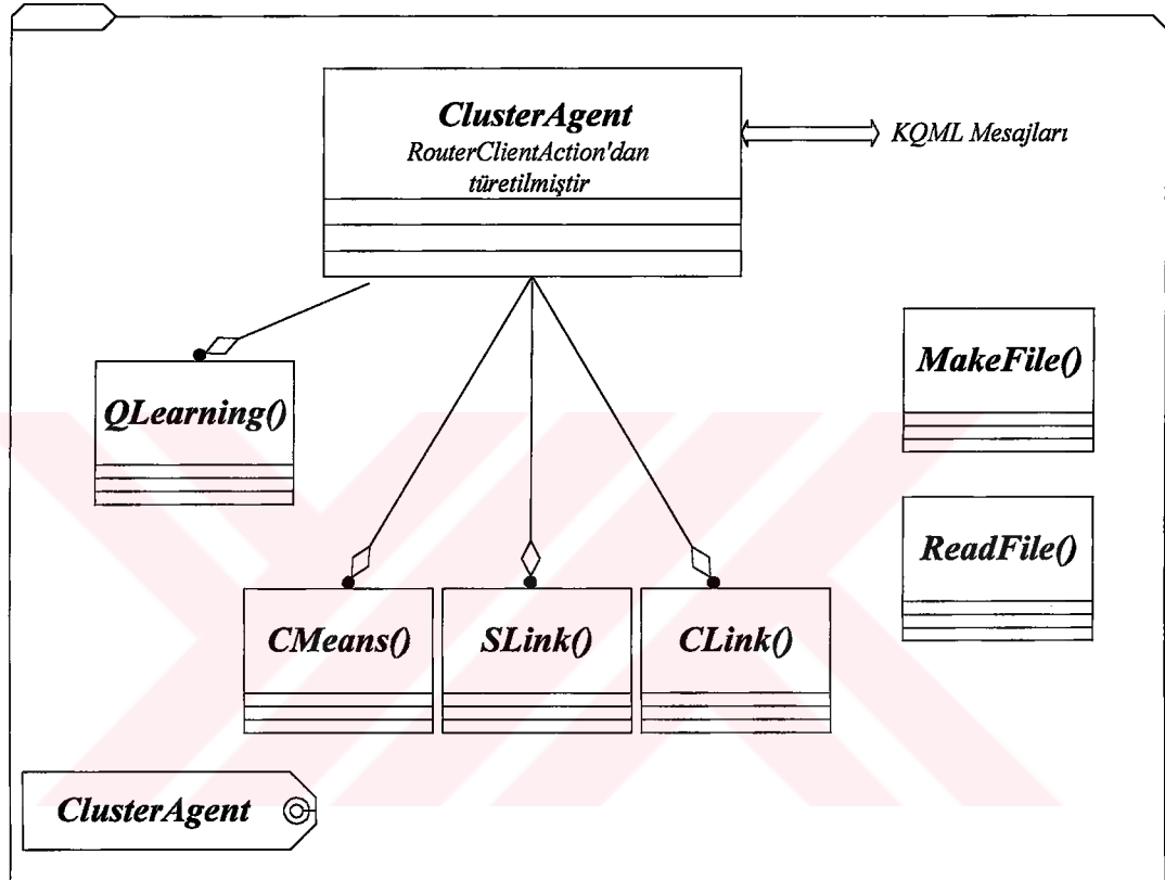
Şekil 8.9 ClusterAgent Sınıfı
