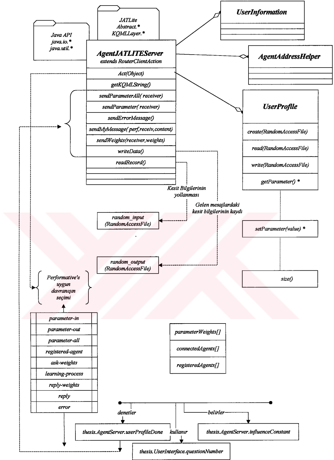
Şekil 8.3 AgentJATLITEServer Sınıf Hiyerarşisi
