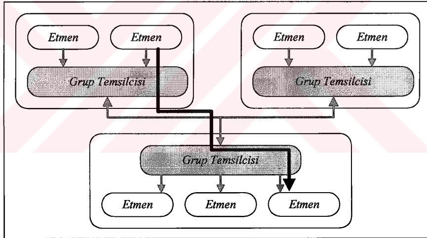
Şekil 2.4 Birleşik Sistemlerde İletişim
