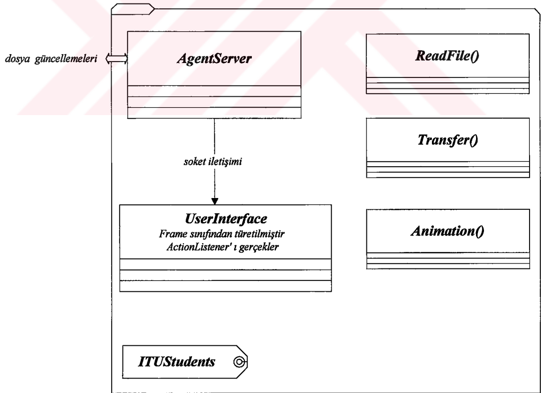
Şekil 8.8 ITUStudents Sınıfı
