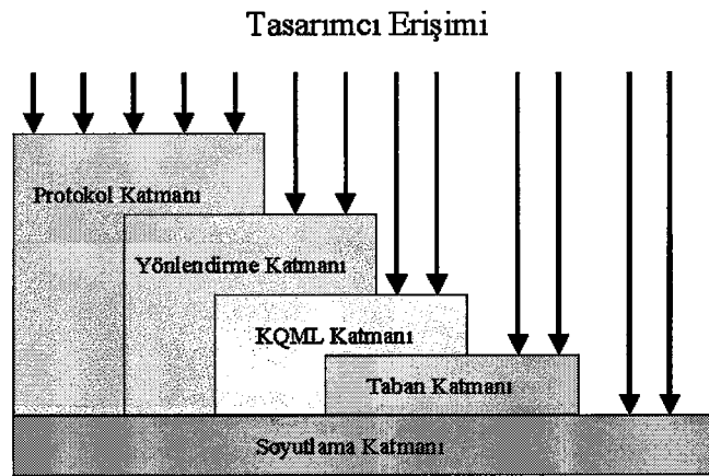
Şekil 2.7 JATLite Katmanları
