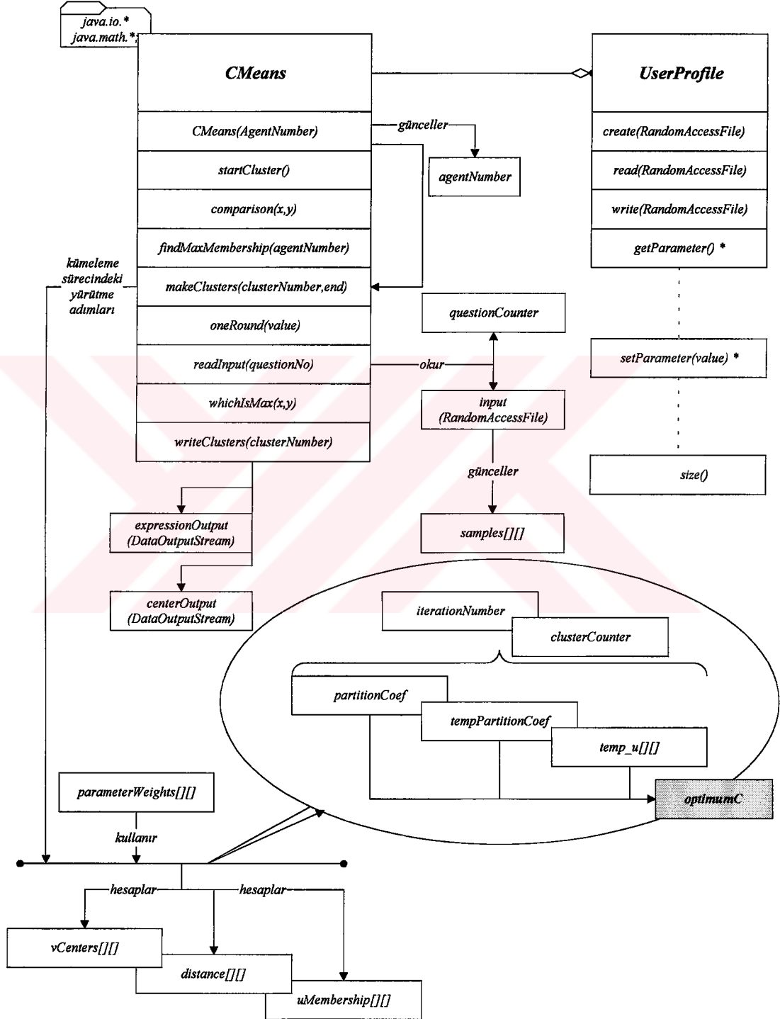
Şekil 8.12 CMeans Sınıf Hiyerarşisi
