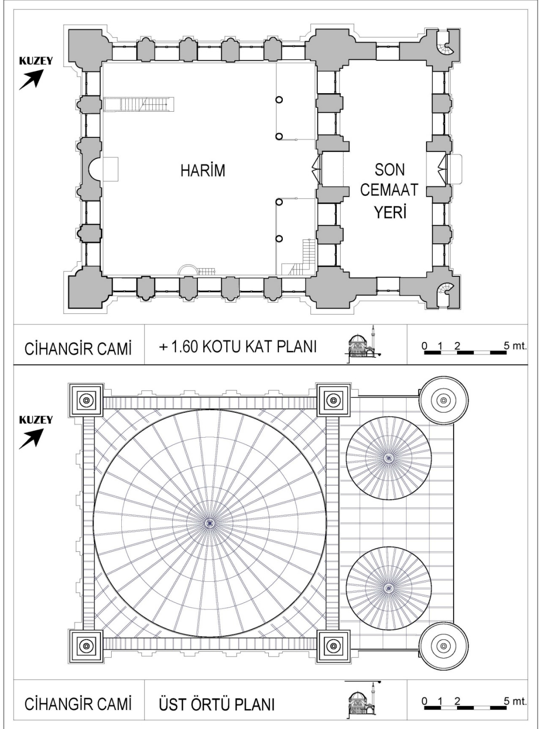
Şekil 4.3: Cihangir Camisi üstte plan, altta üst örtü planı, 2015
