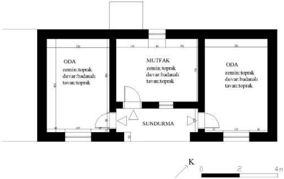
Şek.C2.8A/2. [59.7.1/1] no'lu evin planı
