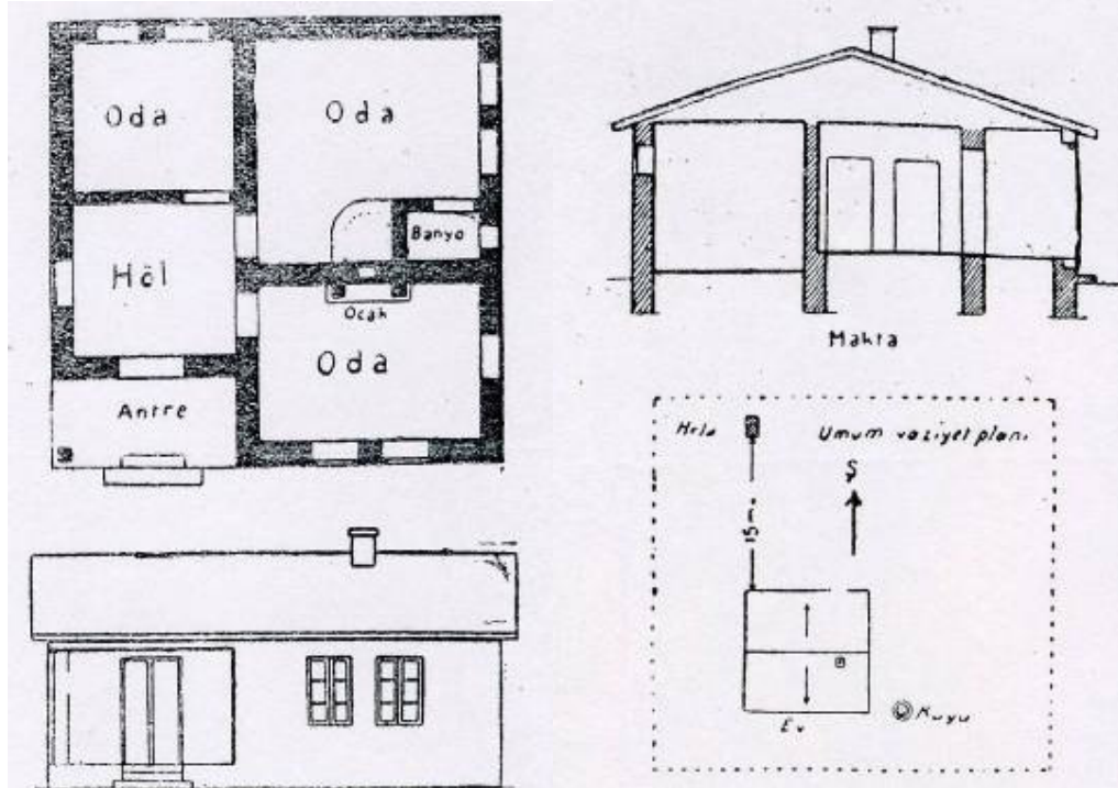
Şek.B9/25. Sıhhi köy evi projesi (Anonim, 1941)
