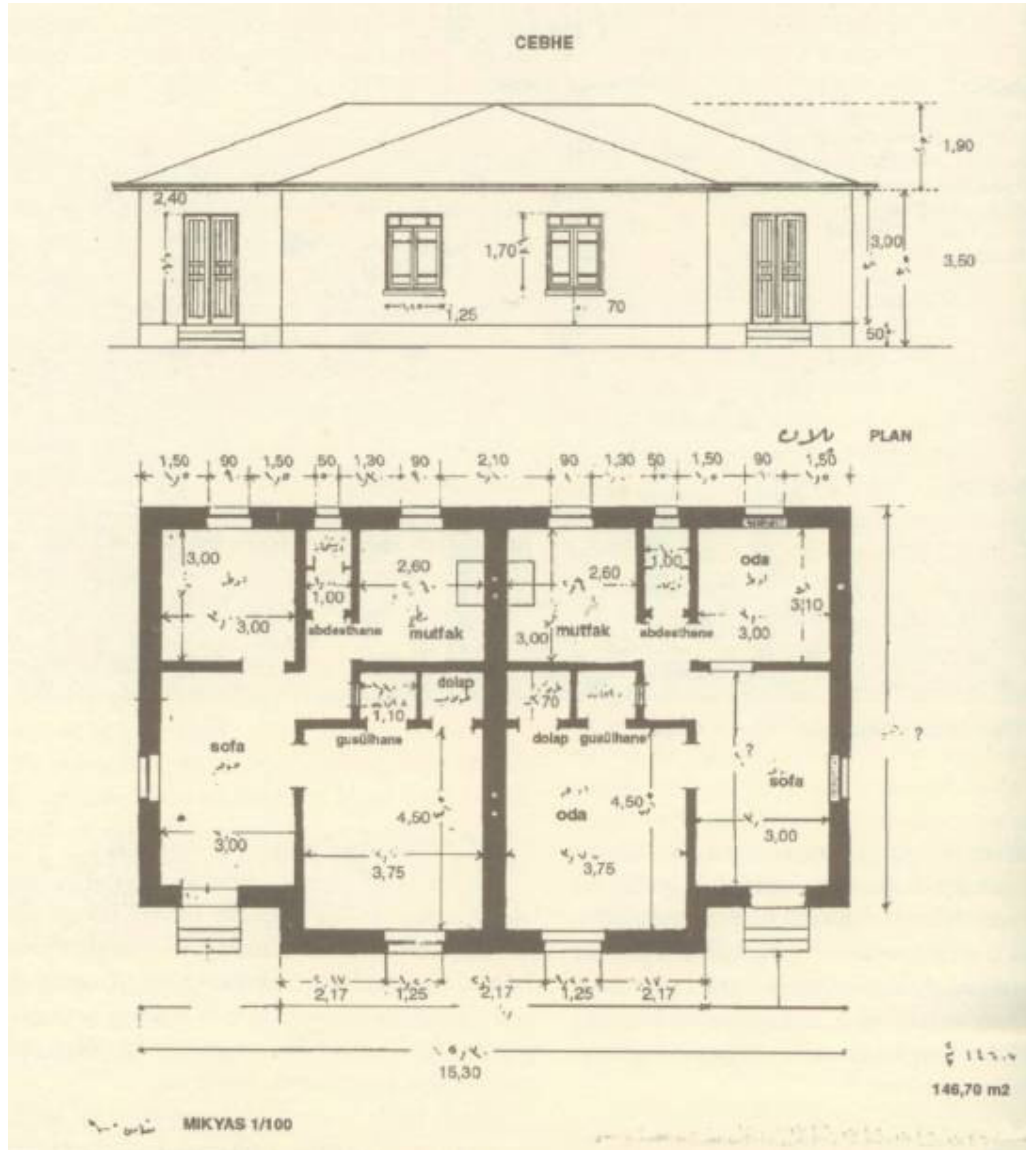
Şek.B9/31. Manisa Çobanisa Köyü konut projesi (Cengizkan, 2004a:44)
