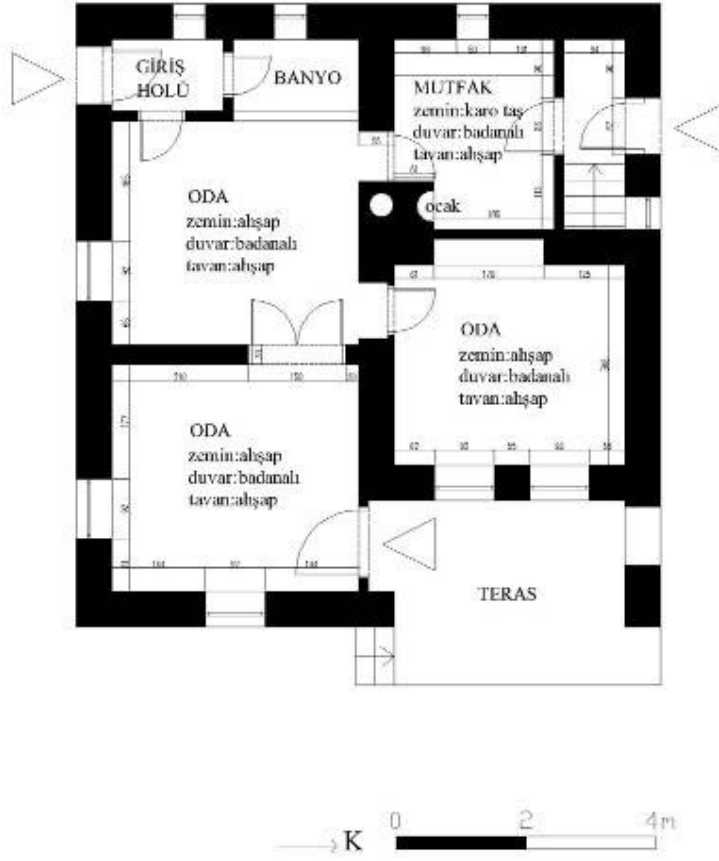
Şek.C2.5A/15. [39.1.5/6] no'lu öğretmen lojmanı planı
