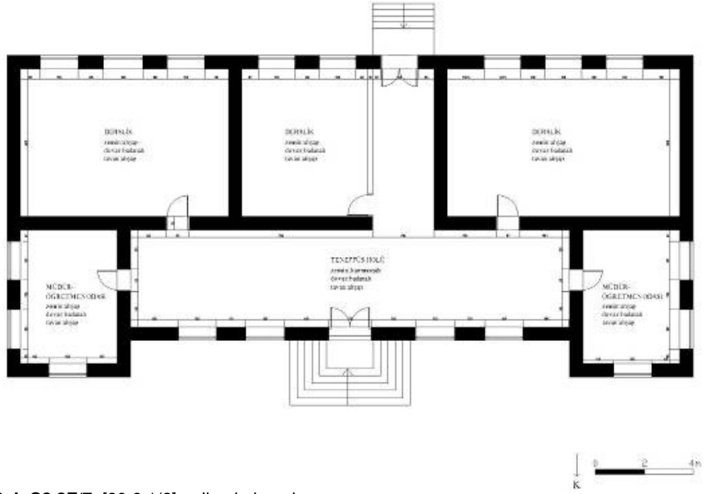
Şek.C2.3F/7. [39.8.1/2] no'lu okulun planı
