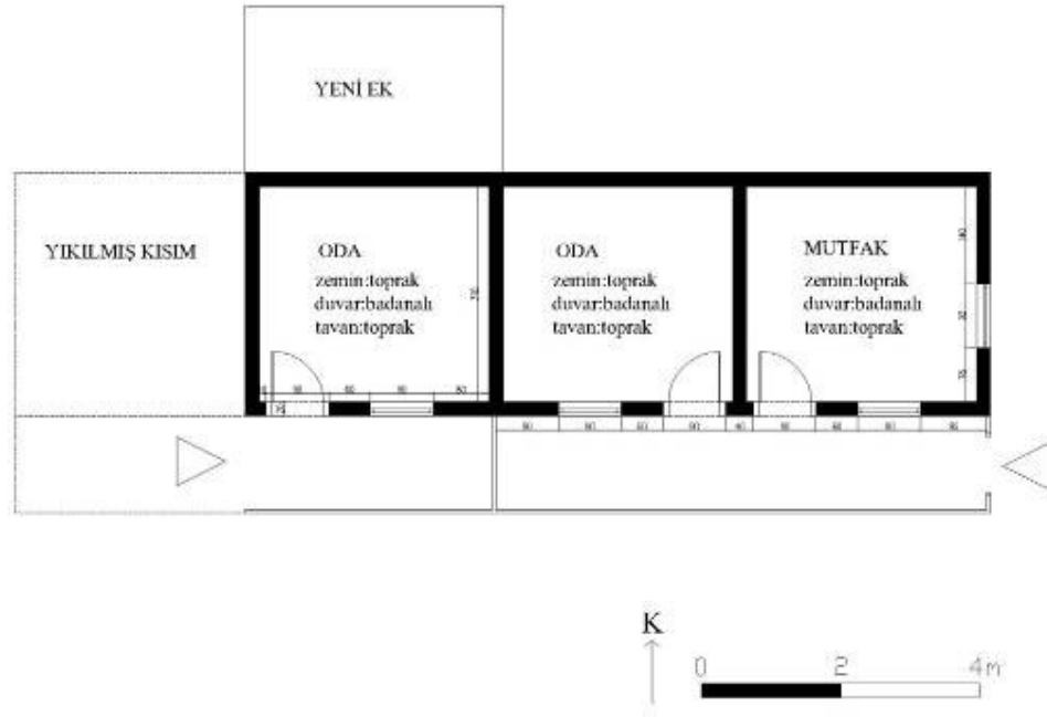
Şek.C2.4C/2. [39.5.2/1] no'lu ikiz evin planı
