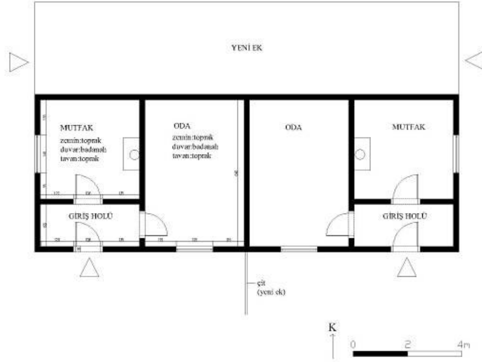
Şek.C2.4C/4. [39.5.2/2] no'lu ikiz evin planı
