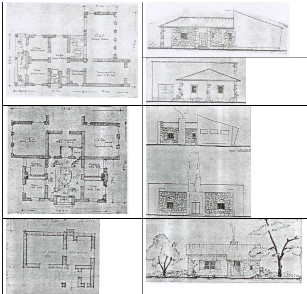
Şek.B1/6. Behçet Ünsal tarafından tasarlanan köy evi projeleri (Ünsal, 1940)
