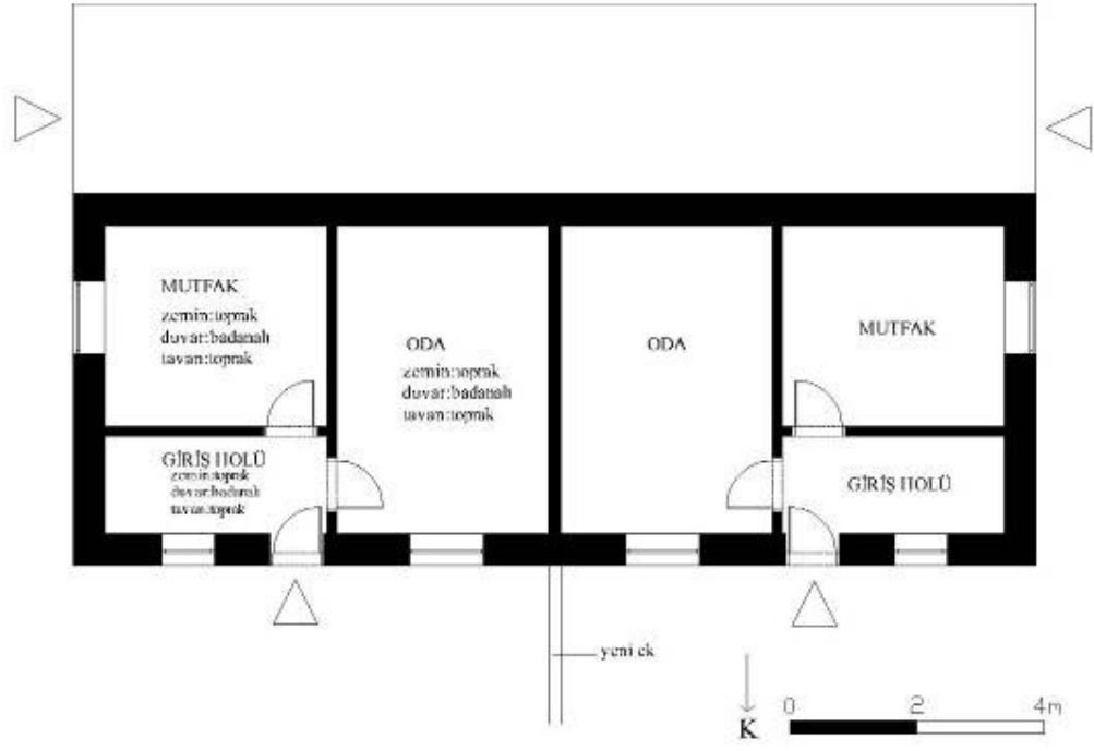
Şek.C2.3D/20. [39.7/4] no'lu evin planı
