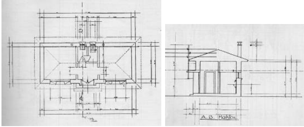
Şek.B9/1. Köy konağı plan ve kesiti (İKKP, 1939:21-22)
