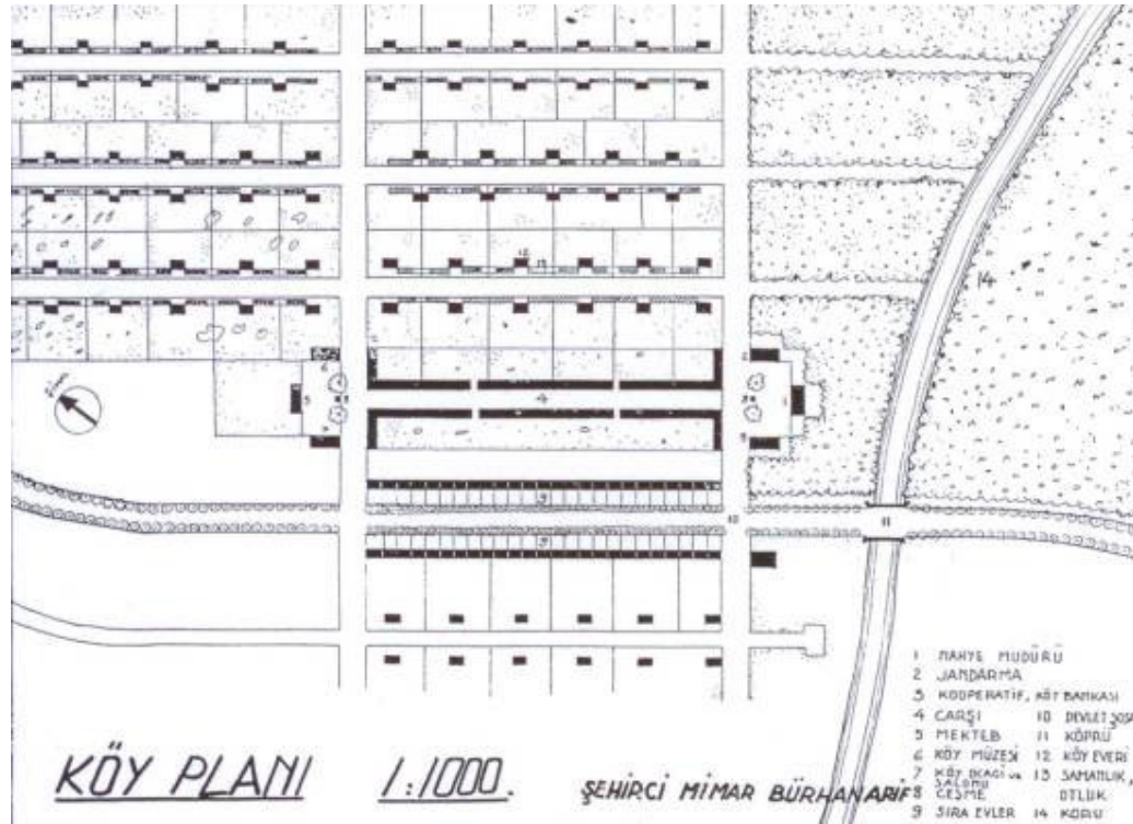
Şek.B1/2. Burhan Arif'in tasarladığı köy projesi (Burhan Arif [Ongun], 1935:320)
