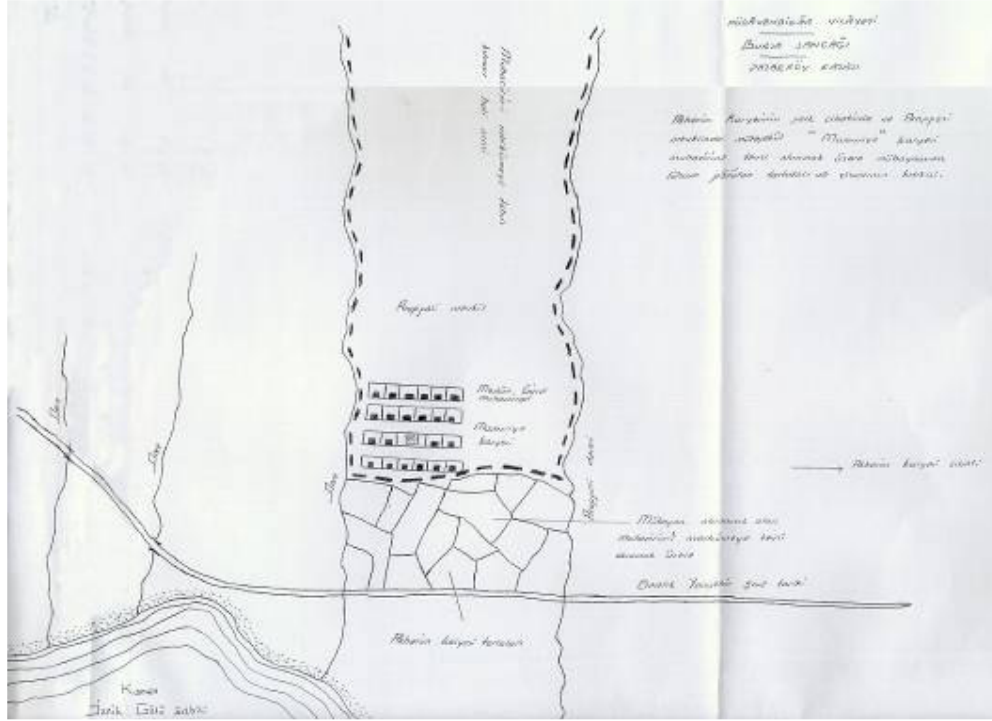
Şek.A4/14. 1900 yılında Giritli göçmenlerin kurduğu Mamure (Gölyaka) Köyü'nün BOA'nde bulunan 1901 tarihli yerleşme planı (Yadigar, 1980:[76])
