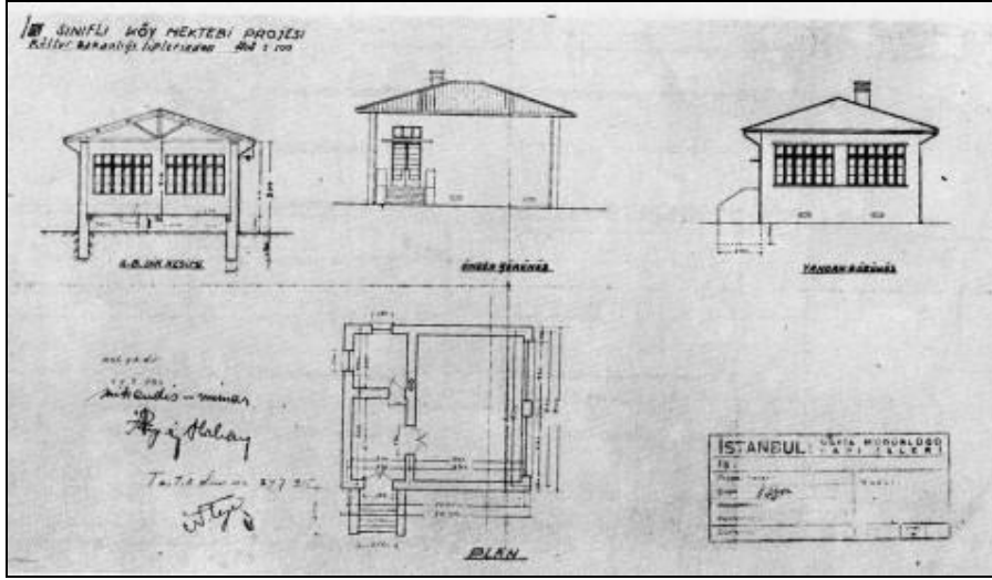
Şek.B9/2. Bir sınıflı köy okulu projesi (İKKP, 1939:54)
