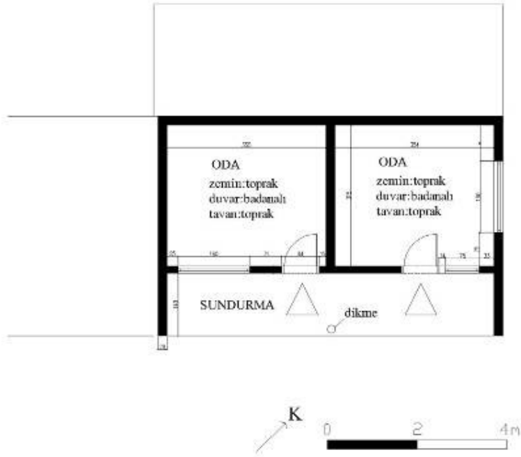
Şek.C2.8B/2. [59.7.2/1] no'lu evin planı
