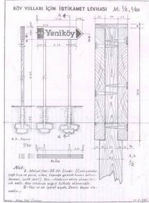
Şek.B9/27. Köy yolu levhası (Anonim, 1944:5)
