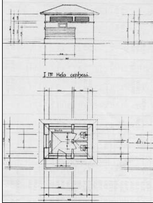
Şek.B9/13. Köy helası projesi (İKKP, 1939:39-40)
