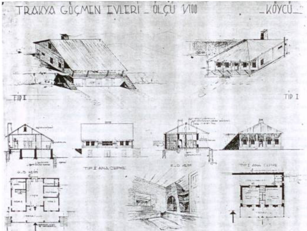
Şek.B1/8. Abdullah Ziya'nın "Halkevi Trakya Göçmen Evleri Proje Yarışması"nda birinci olan projesi (Abdullah Ziya [Kozanoğlu], 1935a:205)
