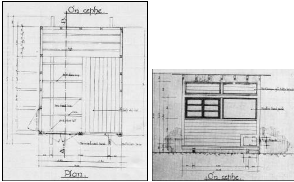
Şek.B9/8. Kütüphane projesi (İKKP, 1939:46, 49)
