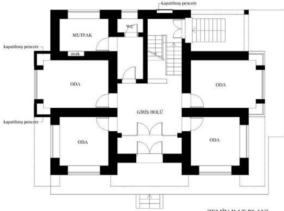
ZEMİN KAT PLANI
