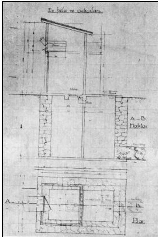
Şek.B9/14. Köy evi helası projesi (İKKP, 1939:42)
