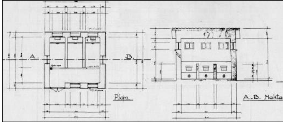
Şek.B9/7. Ahır projesi (İKKP, 1939:51)
