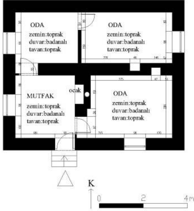
Şek.C2.3D/5. [39.7/1] no'lu evin planı
