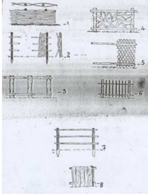
Şek.B9/26. Trakya için önerilerilen çit tipleri (TKK, 1941:[211])
