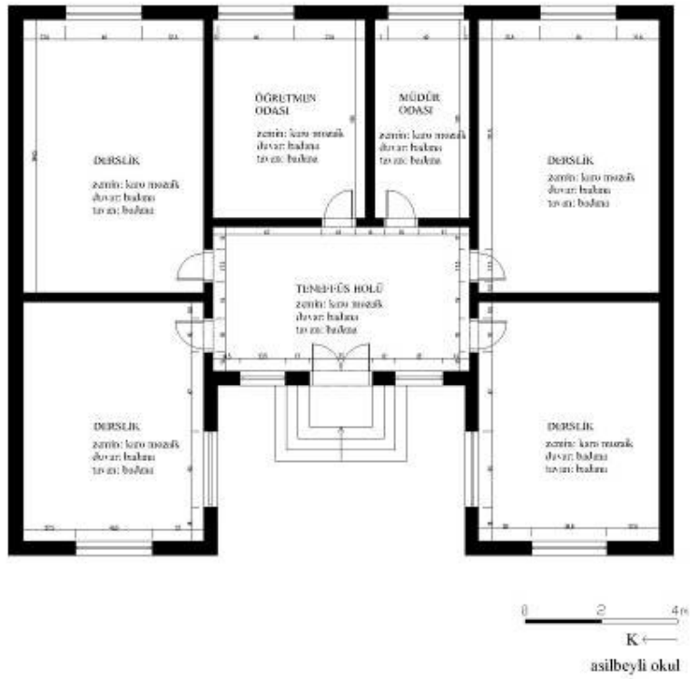
Şek.C2.4A/2. [39.1.4/1] no'lu Asilbeyli Köyü Okulu planı
