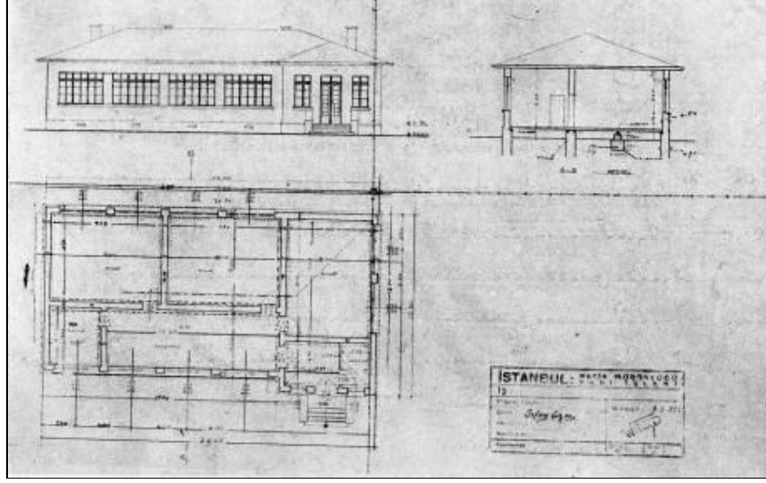
Şek.B9/4. Üç sınıflı köy okulu projesi (İKKP, 1939:56)
