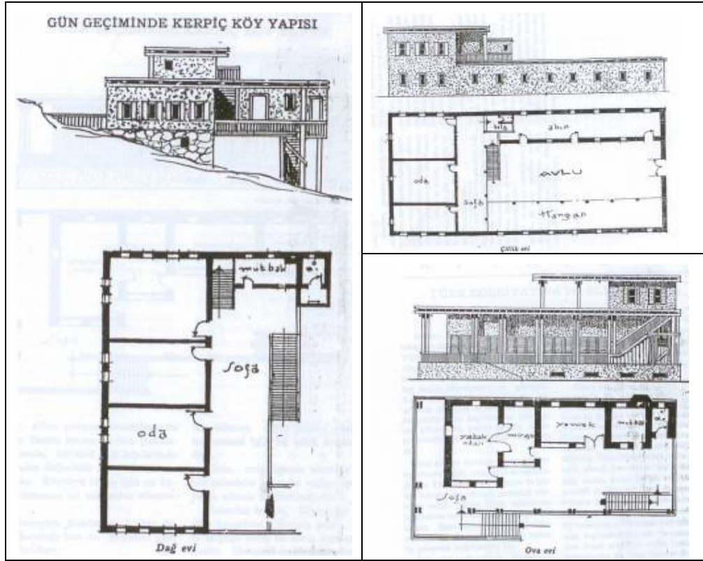
Şek.B1/7. Abdullah Ziya tarafından tasarlanan köy evi projeleri (Abdullah Ziya [Kozanoğlu], 1934:67-69)
