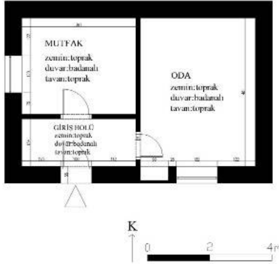
Şek. C2.3C/3. [39.7.1/1] no'lu evin planı
