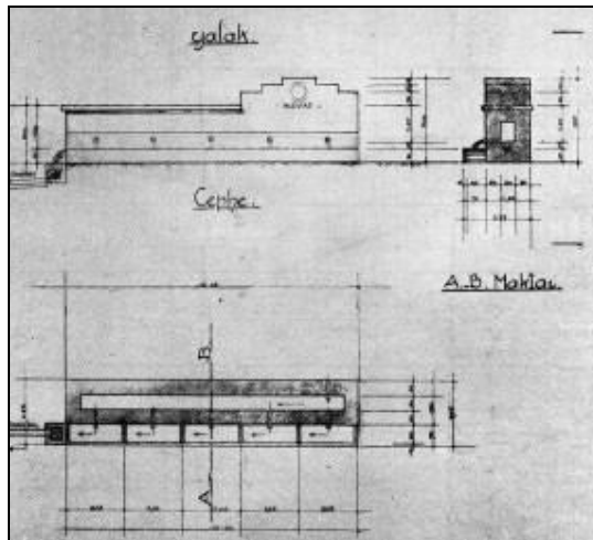
Şek.B9/12. Köy çeşmesi projesi (İKKP, 1939:33)
