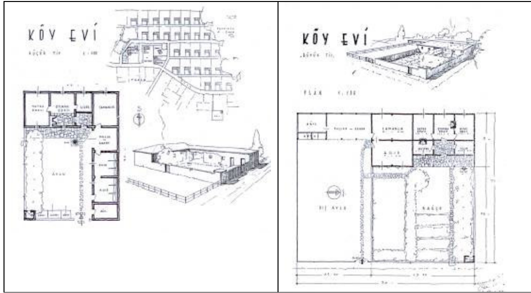
Şek.B1/5. Abidin Mertaş'ın tasarladığı köy projesi (Mertaş, 1940)
