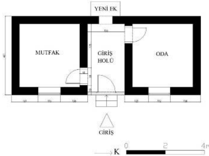
Şek.C2.6B/2. [39.6.1/1] no'lu yapının planı
