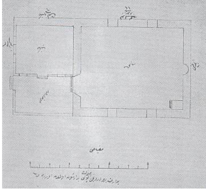
    A4/4. Kabaag    K    cami ve okulunun BOA'nde bulunan 1866 tarihli planı (Kocacık, 1979:1)
