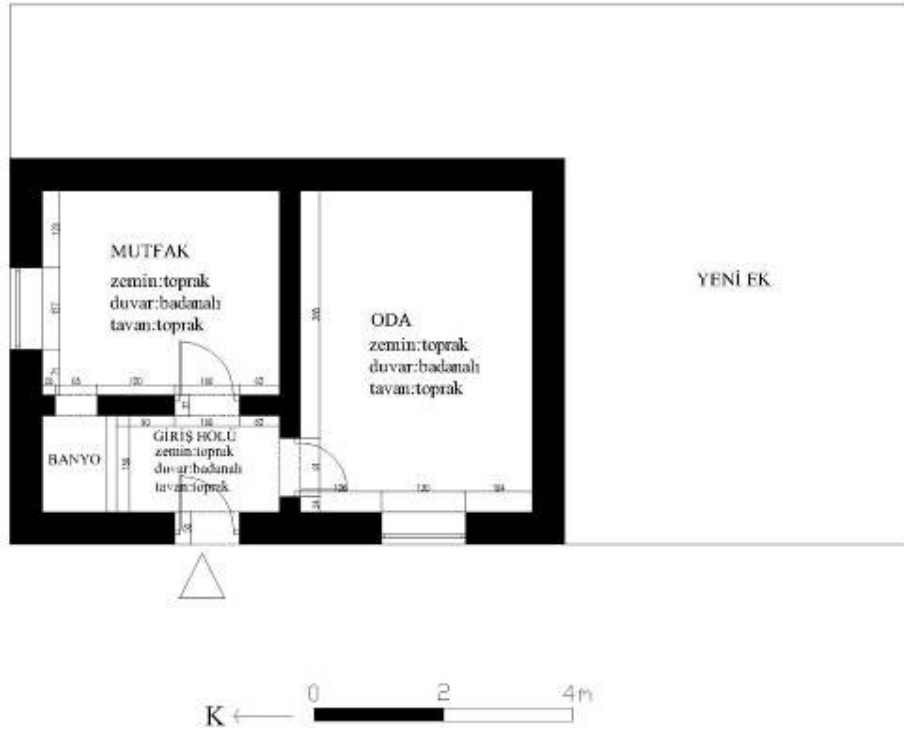
Şek.C2.5A/3. [39.1.5/1] no'lu evin planı
