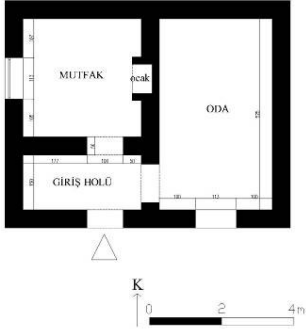
Şek.C2.3D/8. [39.7/2] no'lu evin planı
