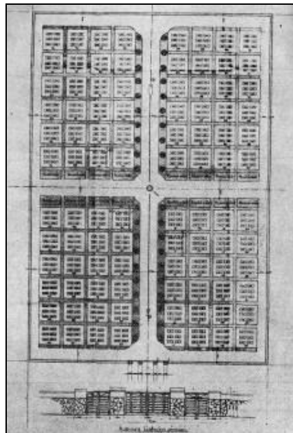
Şek.B9/17. Köy mezarlığı projesi (İKKP, 1939:31)
