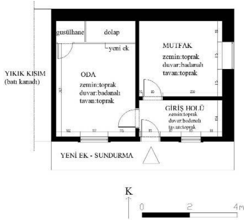
Şek.C2.3D/18. [39.7/3] no'lu evin planı
