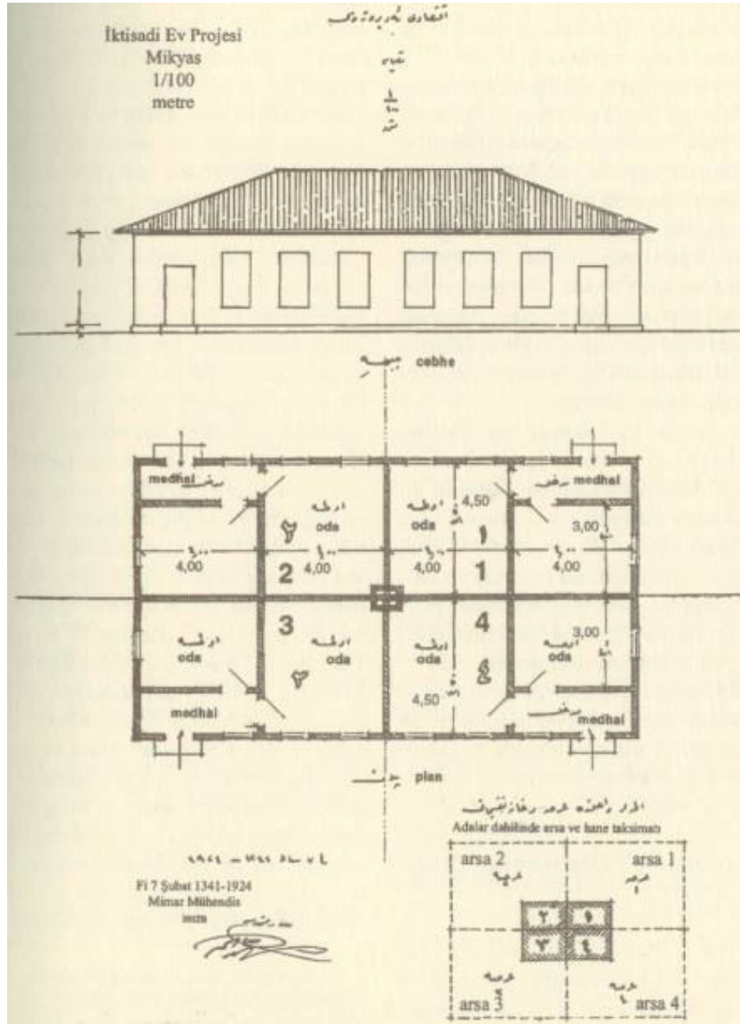
Şek.B9/32. İktisadi hane projesi (Cengizkan, 2004a:45)
