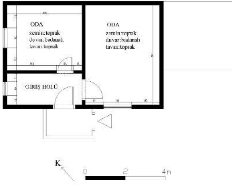
Şek.C2.8C/2. [59.7.3/1] no'lu evin planı
