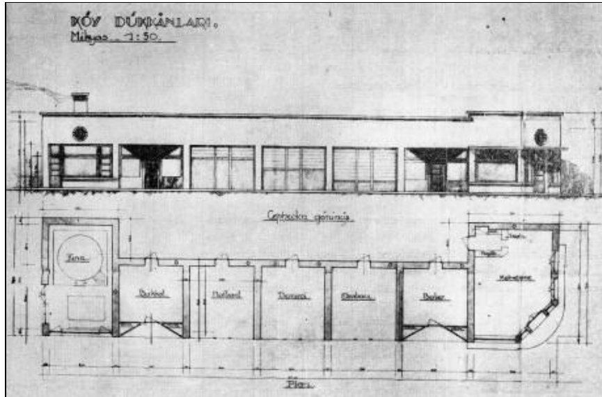
Şek.B9/6. Köy dükkanları projesi (İKKP, 1939:44)
