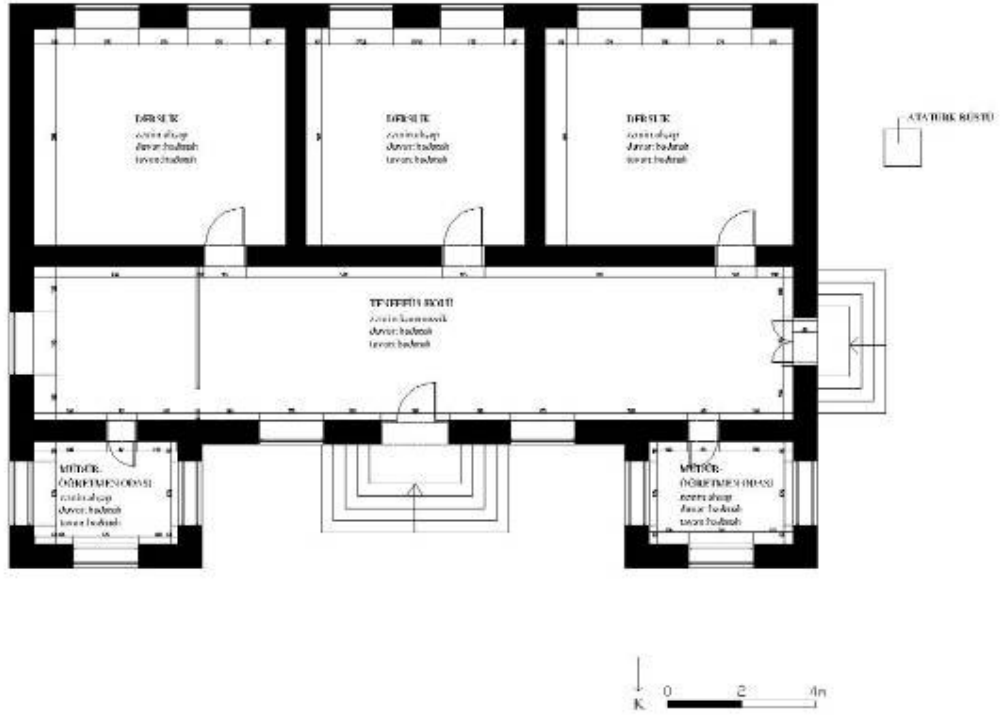
Şek.C2.5A/10. [39.1.5/5] no'lu okulun planı
