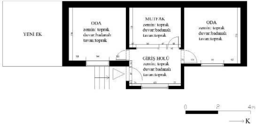
Şek.C2.3F/2. [39.8.1/1] no'lu evin planı
