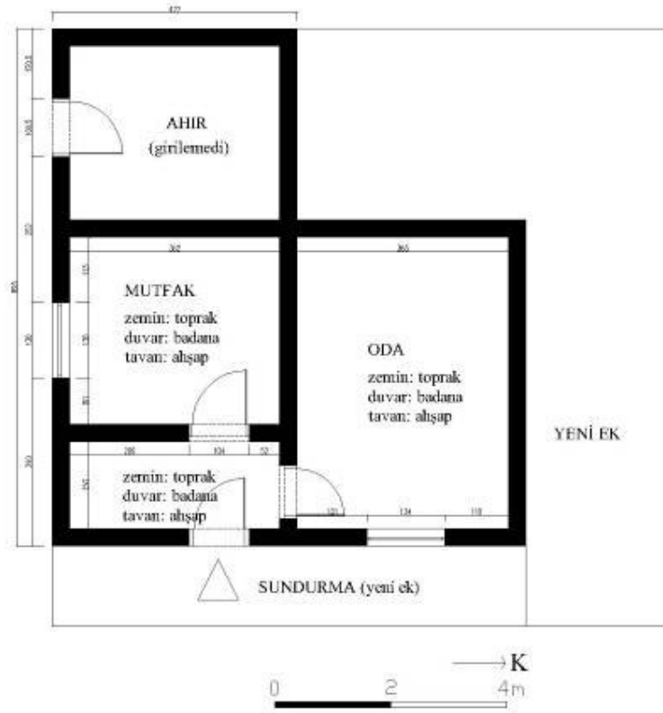
Şek. C3A/4. Arizbaba Köyü'nde belgelenen [39.1.9/37] no'lu evin planı
