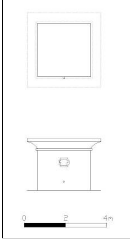
Şek.C2.5B/7. [39.1.6/2] no'lu çeşmenin planı Şek.C2.5B/8. [39.1.6/2] no'lu çeşme ve park
