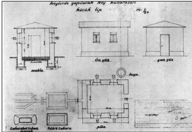
Şek.B9/11. Küçük köy kanarası projesi (İKKP, 1939:29)
