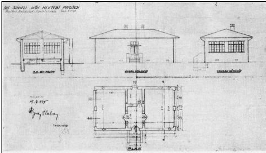
Şek.B9/3. İki sınıflı köy okulu projesi (İKKP, 1939:55)
