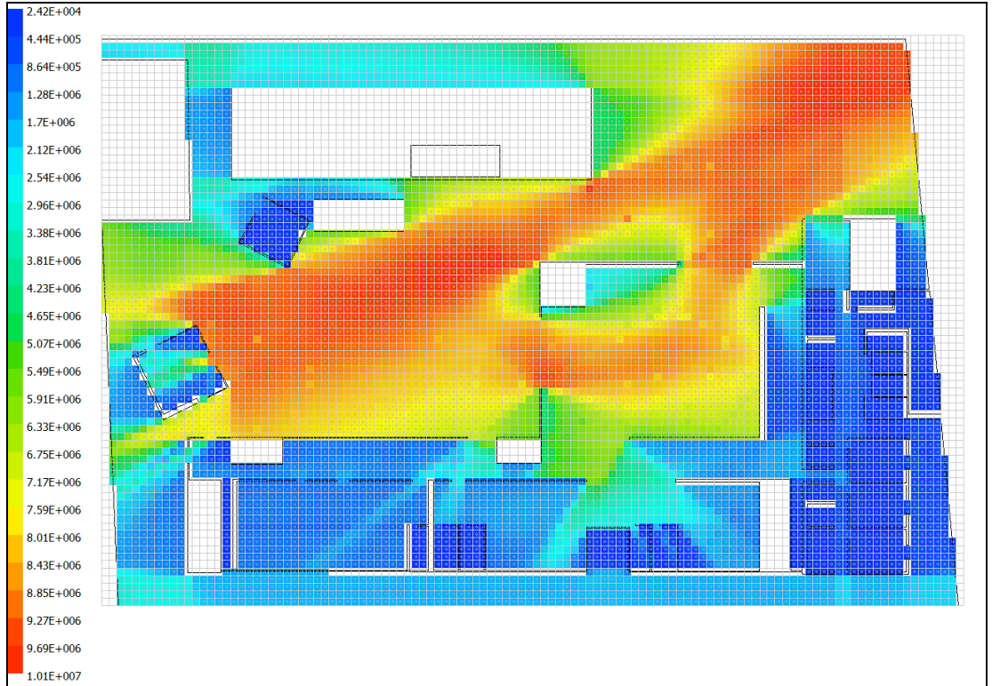
Şekil 5.36 : Eskişehir Belediyesi, Zemin Katı Ortalama Eşgörüş Alanı Değerlerinin Dağılımı.
