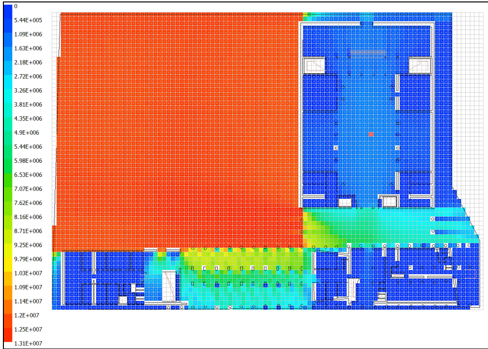
Şekil 5.9 : İstanbul Belediye Sarayı, Zemin Katı Ortalama Bütünleşme Değerlerinin Dağılımı.
