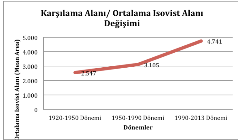
Şekil 5.50 : Giriş/Karşılama Alanı-Ortalama Eşgörüş Alanı (Area)-1920-2013 Değişim Grafiği.
