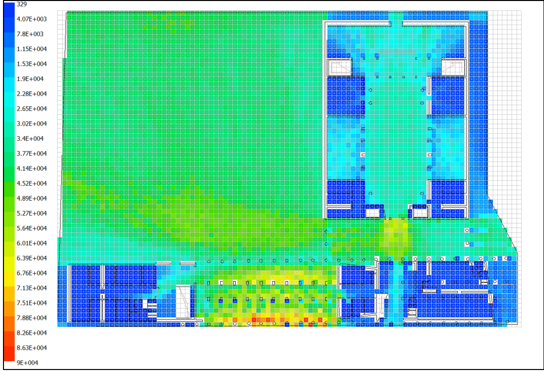
Şekil 5.10 : İstanbul Belediye Sarayı, Zemin Katı Ortalama Eşgörü Çevresi Değerlerinin Dağılımı.
