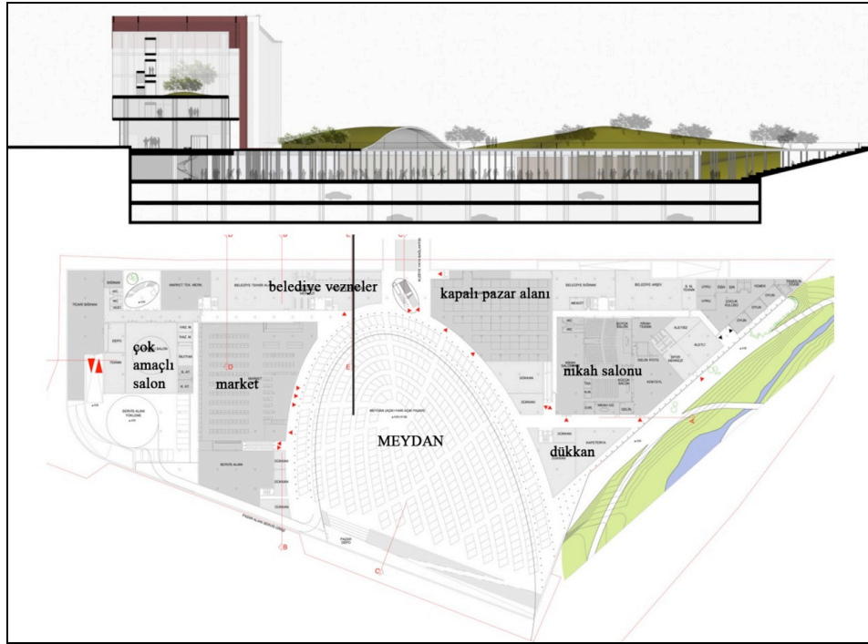
Şekil 3.35 : Manisa Belediyesi Hizmet Binası ve Çevresi Ulusal Mimari Proje Yarışması 1.Ödül Zemin Kat Planı ve Kesiti (URL 9)
