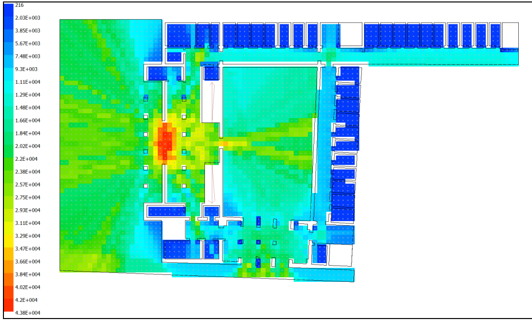
Şekil 5.5 : Adana Belediye Sarayı, Ortalama Eşgörüş Çevresi Değerlerinin Dağılımı.
