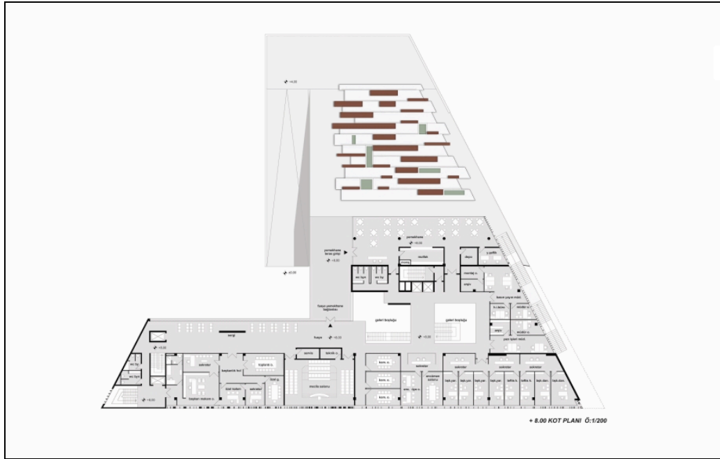
Şekil 3.32 : Kadirli Belediyesi Hizmet Binası ve Kültür Merkezi Yarışması 1.Ödül +8.00 Kotu Planı (URL 8).
