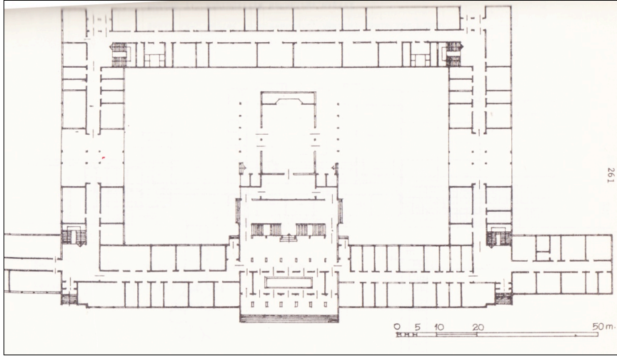
Şekil 3.6 : Devlet Demiryolları Merkez Binası Zemin Kat Planı (Aslanoğlu, 1980).
