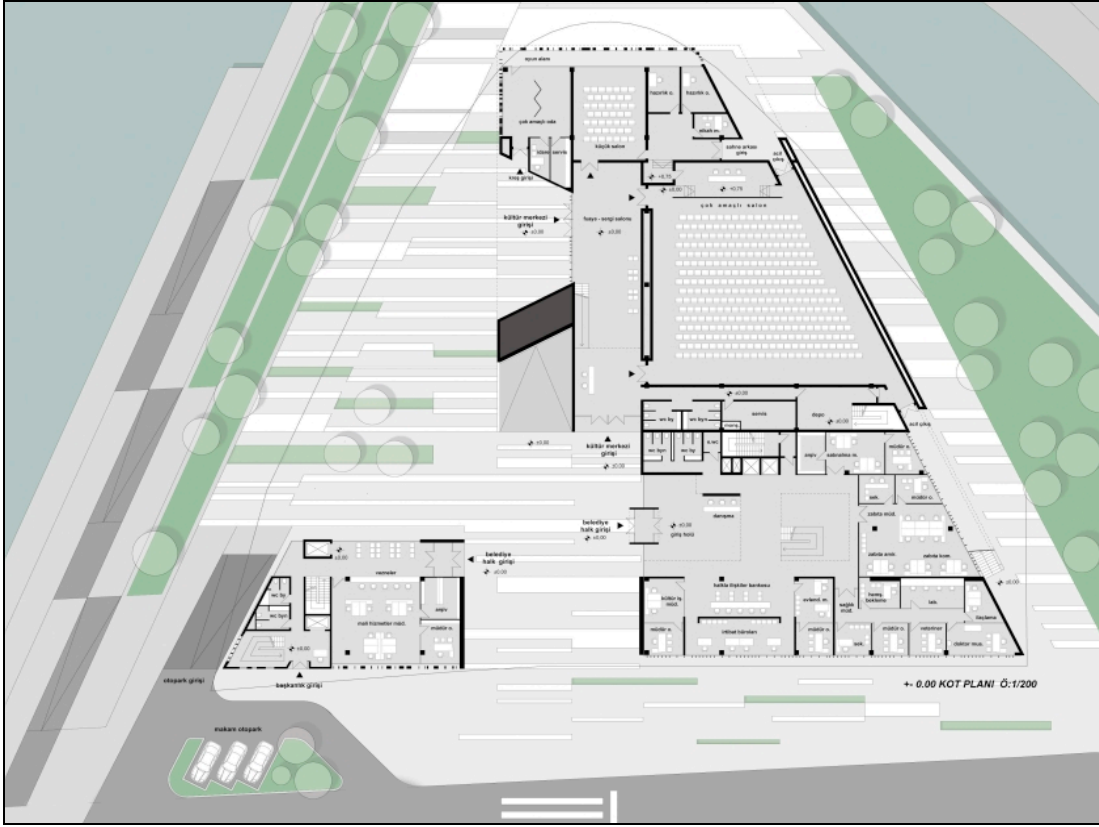
Şekil 3.30 : Kadirli Belediyesi Hizmet Binası ve Kültür Merkezi Yarışması 1.Ödül Zemin Kat Planı (URL 8).
