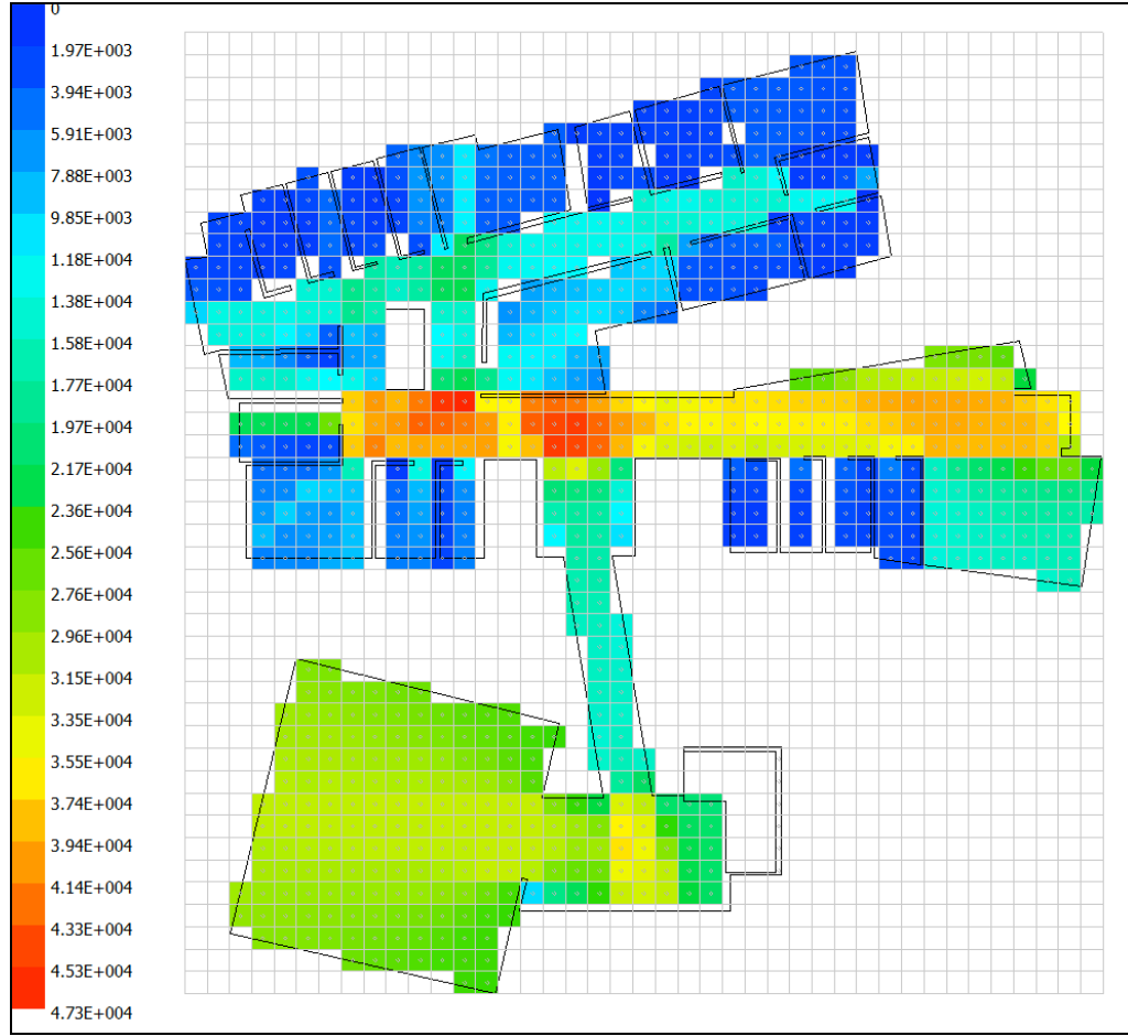
Şekil 5.31 : Trabzon Belediyesi, Meclis Katı Ortalama Bütünleşme Değerlerinin Dağılımı.
