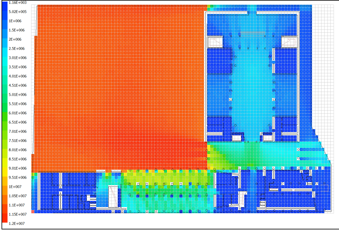
Şekil 5.12 : İstanbul Belediye Sarayı, Zemin Katı Ortalama Eşgörüş Alanı Değerlerinin Dağılımı.
