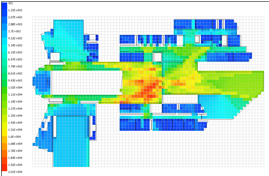
Şekil 5.22 : Gaziantep Belediyesi, Zemin Katı Ortalama Eşgörü Çevresi Değerlerinin Dağılımı.
