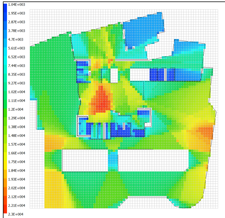
Şekil 5.28 : Trabzon Belediyesi, Zemin Katı Ortalama Eşgörüş Çevresi Değerlerinin Dağılımı.
