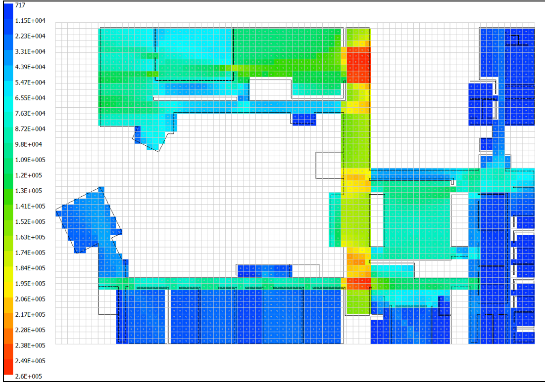
Şekil 5.37 : Eskişehir Belediyesi, Meclis ve Başkanlık Katı Ortalama Bütünleşme Değerlerinin Dağılımı.
