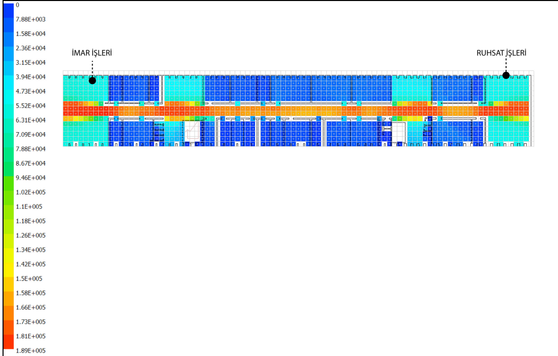
Şekil 5.13 : İstanbul Belediye Sarayı, İmar İşleri Katı Ortalama Bütünleşme Değerlerinin Dağılımı.
