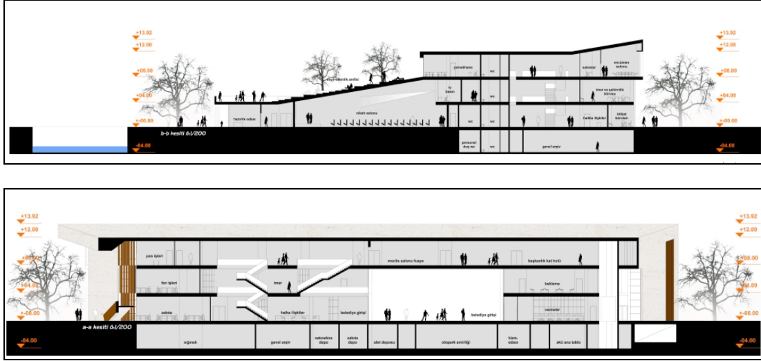
Şekil 3.33 : Kadirli Belediyesi Hizmet Binası ve Kültür Merkezi Yarışması 1.Ödül En ve Boy Kesitleri (URL 8).
