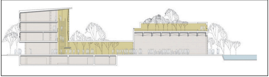
Şekil 3.42 : Uşak Belediyesi Hizmet Binası Kesiti (URL 11).
