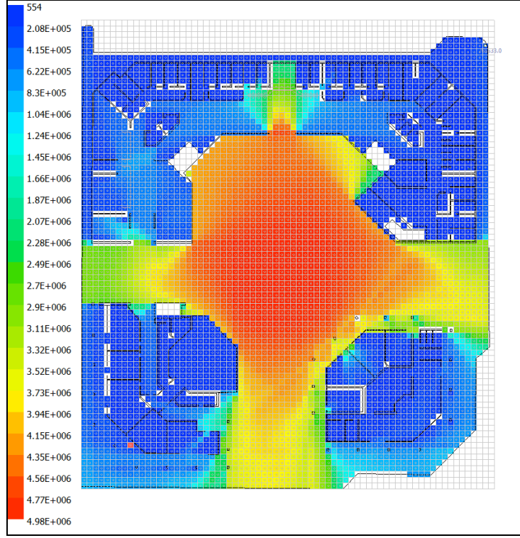
Şekil 5.16 : Samsun Belediyesi, Zemin Katı Ortalama Bütünleşme Değerlerinin Dağılımı.
