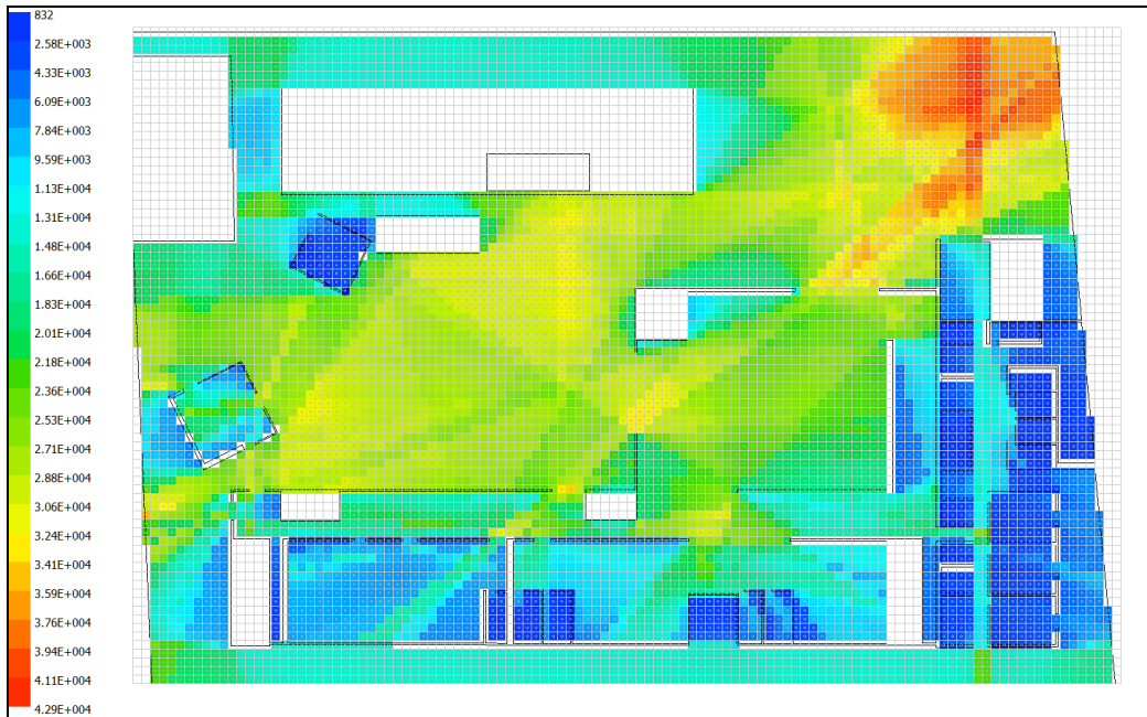
Şekil 5.34 : Eskişehir Belediyesi, Zemin Katı Ortalama Eşgörüş Çevresi Değerlerinin Dağılımı.
