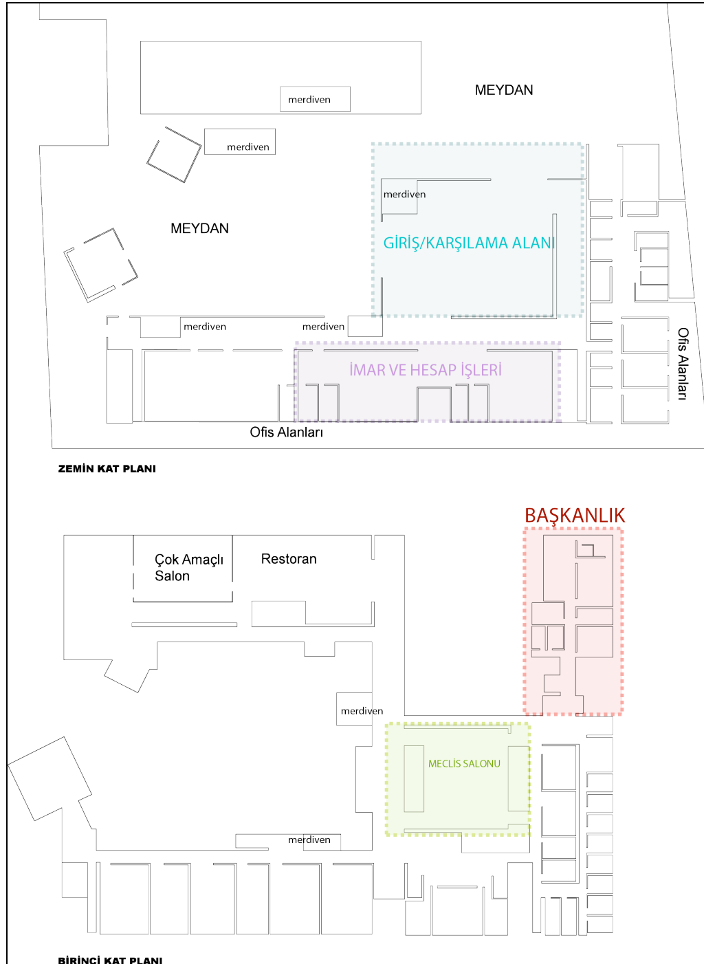
Şekil 5.32 : Eskişehir Belediyesi Zemin Kat ve Birinci Kat Plan Şeması ve Analiz Bölgeleri.
