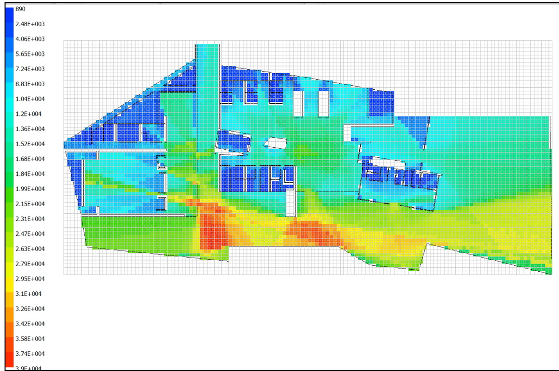
Şekil 5.40 : Çukurova Belediyesi, Zemin Katı Ortalama Eşgörüş Çevresi Değerlerinin Dağılımı.
