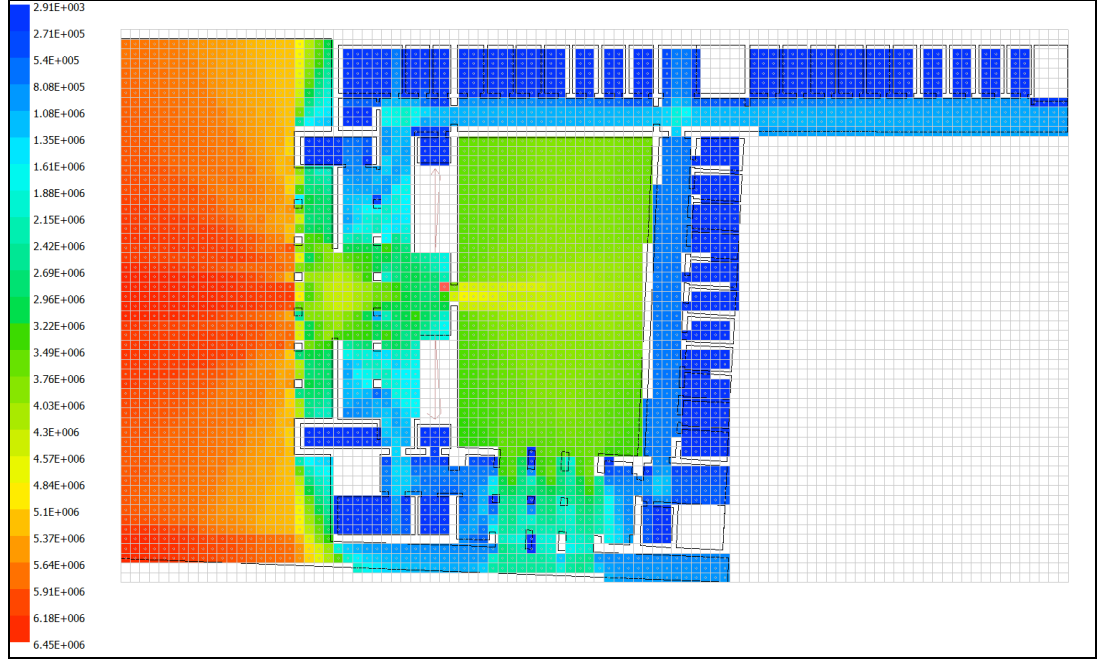
Şekil 5.7 : Adana Belediye Sarayı, Ortalama Eşgörüş Alanı Değerlerinin Dağılımı.
