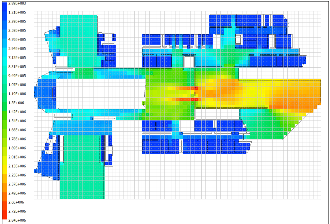
Şekil 5.24 : Gaziantep Belediyesi, Zemin Katı Ortalama Eşgörüş Alanı Değerlerinin Dağılımı.
