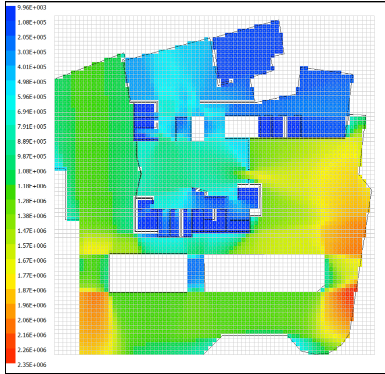
Şekil 5.27 : Trabzon Belediyesi, Zemin Katı Ortalama Bütünleşme Değerlerinin Dağılımı.
