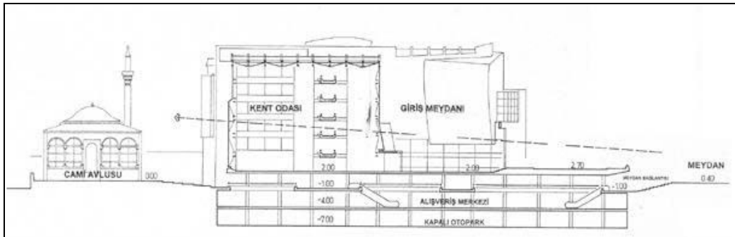
Şekil 3.20 : Trabzon Belediyesi Hizmet Binası Yarışma Projesi (Kesit) (URL-4).
