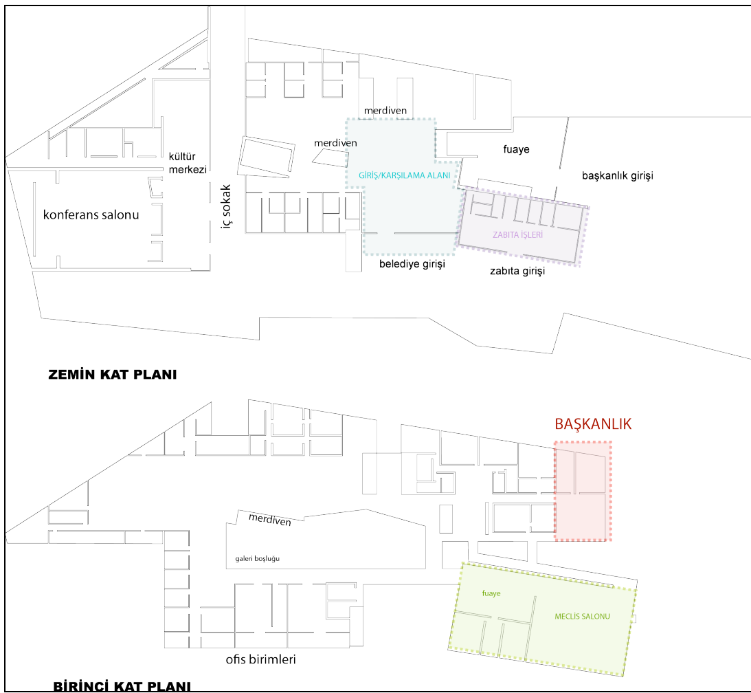
Şekil 5.38 : Çukurova Belediyesi Zemin Kat ve Birinci Kat Plan Şeması ve Analiz Bölgeleri.
