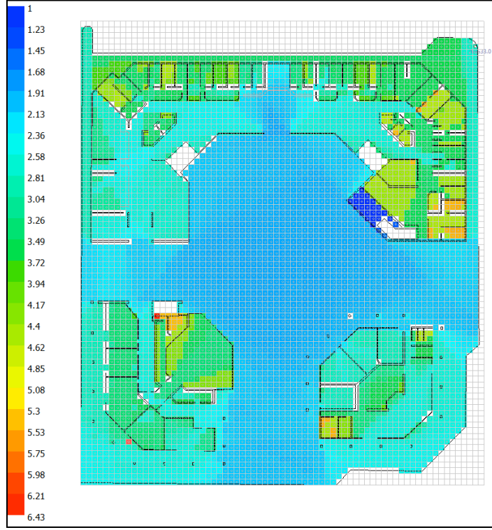
Şekil 5.18 : Samsun Belediyesi, Zemin Katı Ortalama Derinlik Değerlerinin Dağılımı.
