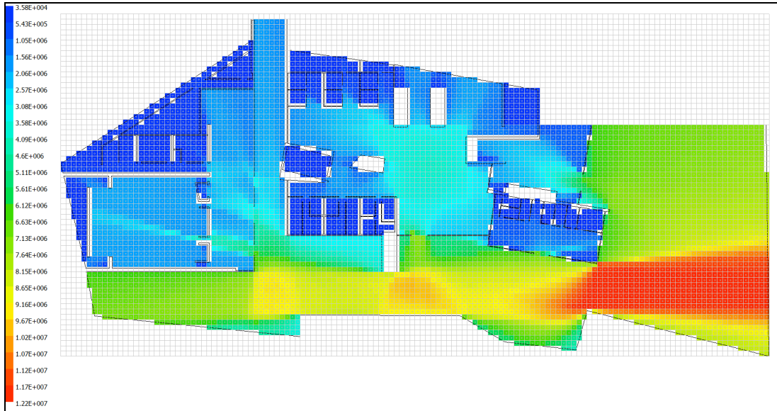
Şekil 5.42 : Çukurova Belediyesi, Zemin Katı Ortalama Eşgörüş Alanı Değerlerinin Dağılımı.
