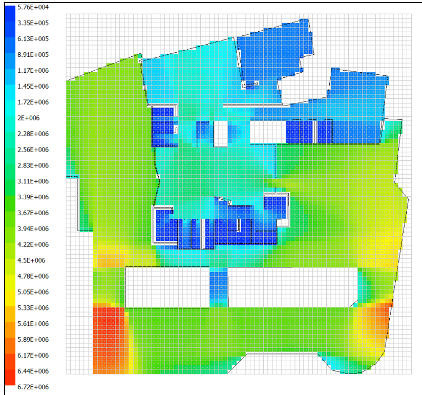
Şekil 5.30 : Trabzon Belediyesi, Zemin Katı Ortalama Eşgörüş Alanı Değerlerinin Dağılımı.
