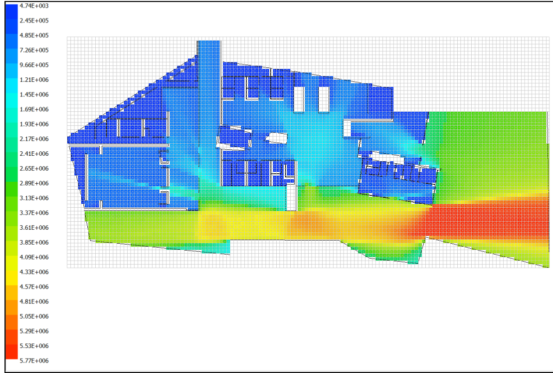
Şekil 5.39 : Çukurova Belediyesi, Zemin Katı Ortalama Bütünleşme Değerlerinin Dağılımı.
