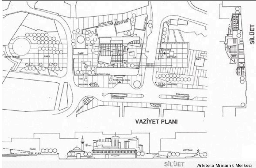
Şekil 3.19 : Trabzon Belediyesi Hizmet Binası Yarışma Projesi Vaziyet Planı (URL 4).
