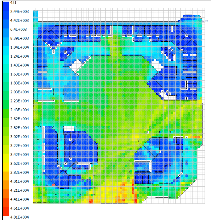
Şekil 5.17 : Samsun Belediyesi, Zemin Katı Ortalama Eşgörü Çevresi Değerlerinin Dağılımı.
