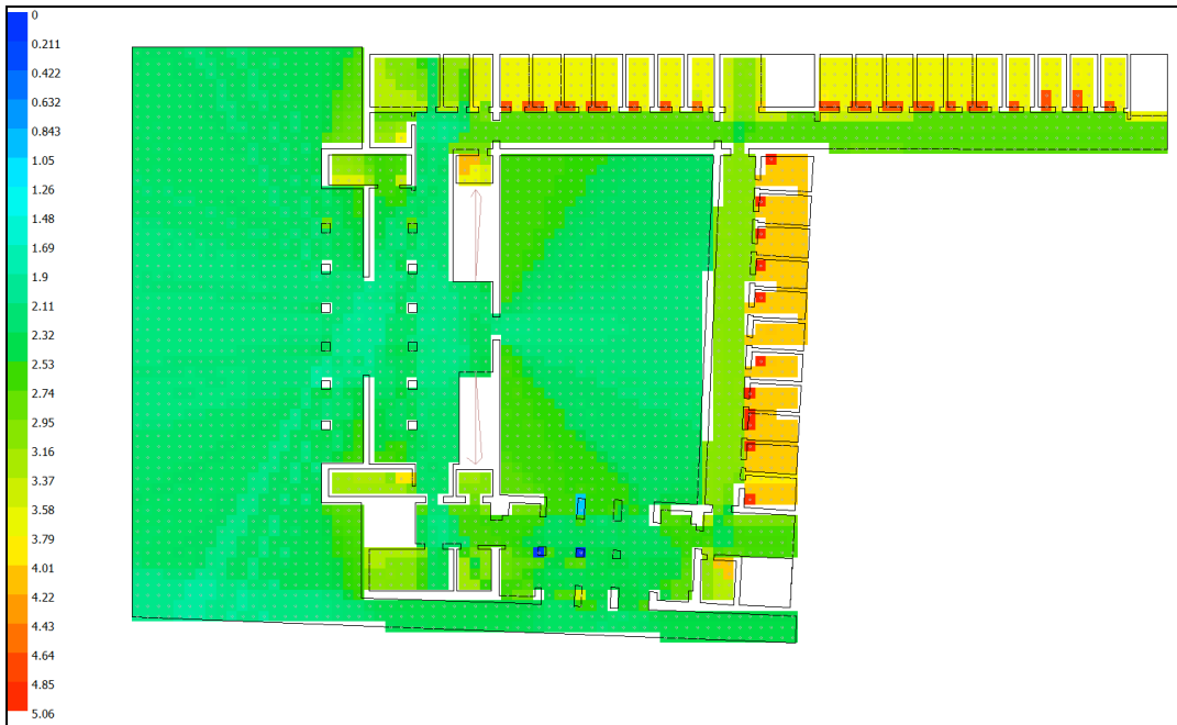
Şekil 5.6 : Adana Belediye Sarayı, Ortalama Derinlik Değerlerinin Dağılımı.
