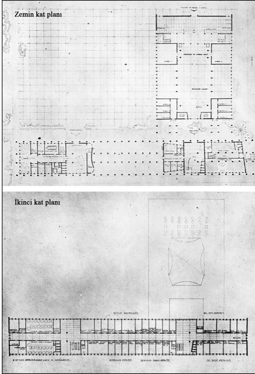
Şekil 3.13 : İstanbul Belediye Sarayı, Kat Planları (Arkitekt,1953, 05-06, s.161).
