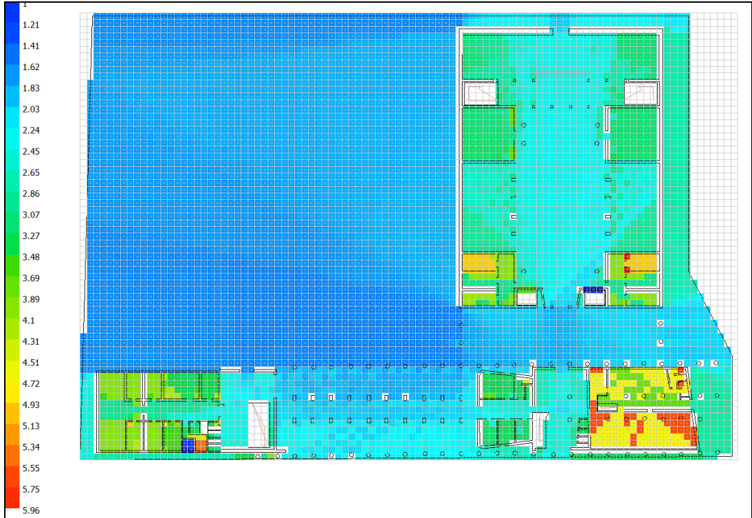
Şekil 5.11 : İstanbul Belediye Sarayı, Zemin Katı Ortalama Derinlik Değerlerinin Dağılımı.
