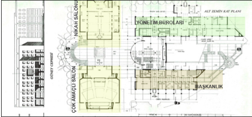
Şekil 3.18 : Gaziantep Belediyesi Hizmet Binası, Hasan Özbay, Tamer Başbuğ tasarımı. Çizim, binanın alt zemin kat planını göstermektedir. Çizim, binanın iç mekanlarının ve dış cephesinin ayrılmış olduğunu göstermektedir.
