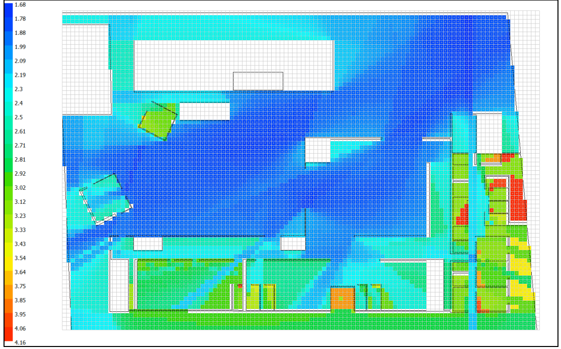
Şekil 5.35 : Eskişehir Belediyesi, Zemin Katı Ortalama Derinlik Değerlerinin Dağılımı.
