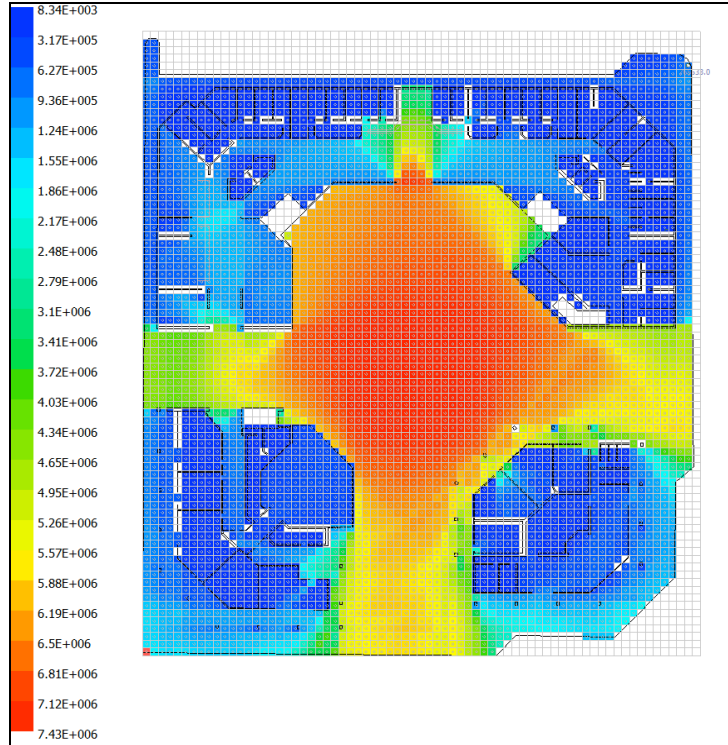
Şekil 5.19 : Samsun Belediyesi, Zemin Katı Ortalama Eşgörüş Alanı Değerlerinin Dağılımı.
