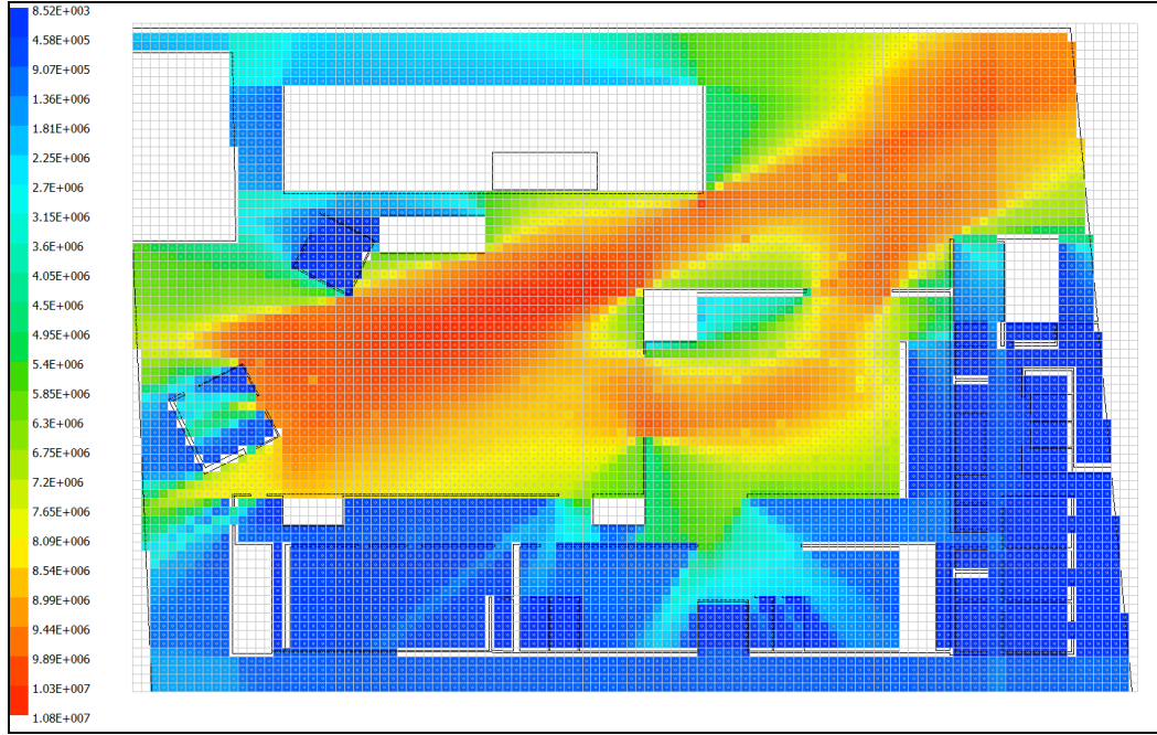
Şekil 5.33 : Eskişehir Belediyesi, Zemin Katı Ortalama Bütünleşme Değerlerinin Dağılımı.
