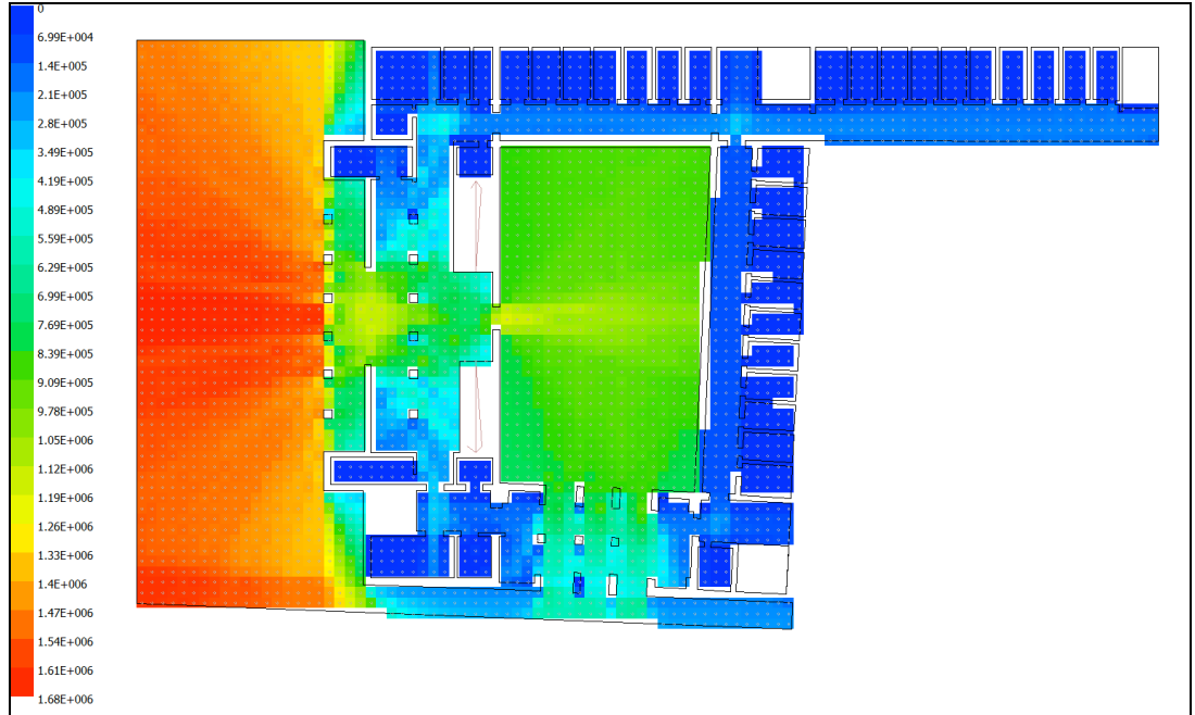
Şekil 5.4 : Adana Belediye Sarayı, Ortalama Bütünleşme Değerlerinin Dağılımı.
