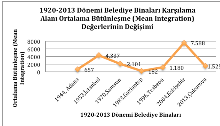
Şekil 5.55 : 1920-2013 Dönemi Belediye Binaları Karşılama Alanı Ortalama Bütünleşme Değerlerinin Değişimi.
