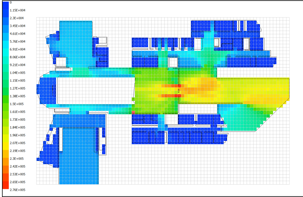
Şekil 5.21 : Gaziantep Belediyesi, Zemin Katı Ortalama Bütünleşme Değerlerinin Dağılımı.
