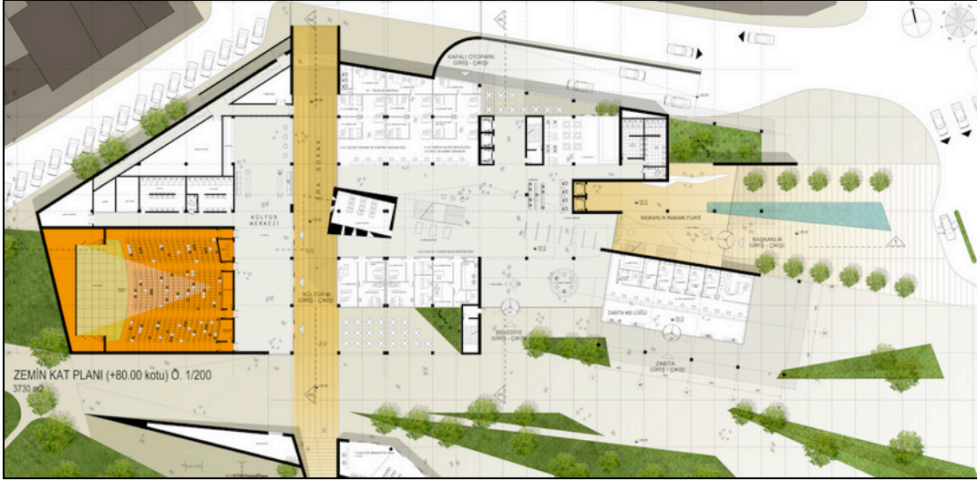
Şekil 3.38 : Adana Çukurova İlçe Belediyesi Hizmet Binası ve Kültür Merkezi, Zemin Kat Planı (URL 10).
