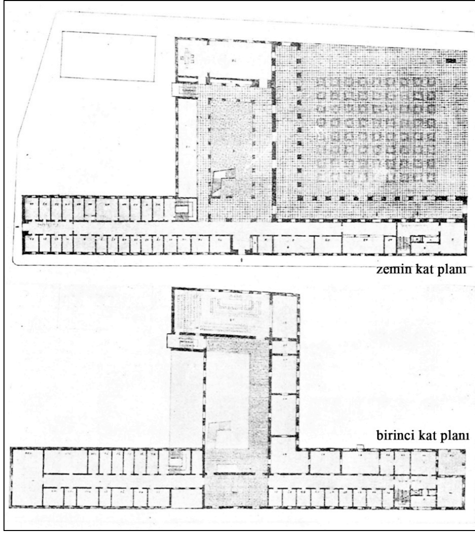
Şekil 3.8 : Adana Adana Belediye Sarayı Yarışması, 1944, Sedat Hakkı Eldem, Samim Oktay ve Demirtaş Kamçıl'ın Önerisi, Birinci ve Zemin Kat Planları (Arkitekt 14, no. 11-12, 1944).
