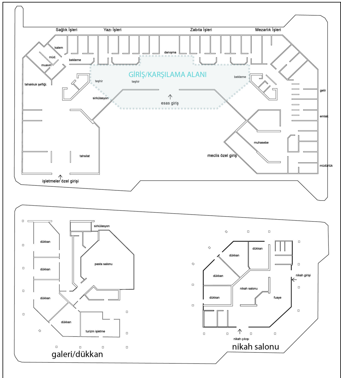
Şekil 5.14 : Samsun Belediyesi Zemin Kat Plan Şeması ve Analiz Bölgeleri.
