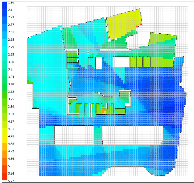
Şekil 5.29 : Trabzon Belediyesi, Zemin Katı Ortalama Derinlik Değerlerinin Dağılımı.
