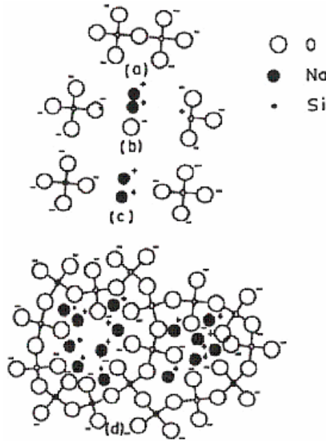
Şekil 2.3: \text{SiO}_2 ile \text{Na}_2\text{O} Arasındaki Reaksiyon ve Bu Reaksiyon Sonucu Oluşan Camın Yapısı, (a) \text{SiO}_2 yapısı, (b) \text{Na}_2\text{O} ' in Yapıya Girmesi, (c) \text{Na}_2\text{O} ' in Oksijen Bağını Koparması, (d) \text{Na}^+ İyonlarının Hollere Yerleşmesi [5]
