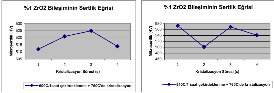
Şekil 7.22: 600°C ve 610°C’de Çekirdeklendirme, 760°C’de Kristalizasyon Isıl İşlemi Uygulanan M7A3 (%1 ZrO 2 ) Grubu Numunelerin Zamana Bağlı Sertlik Değerleri.
