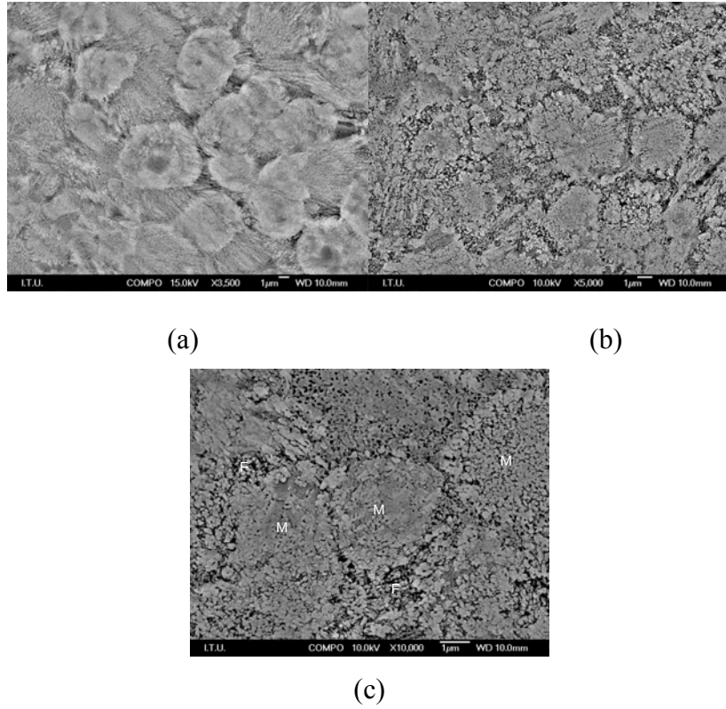
Şekil 7.16: ZrO_2 içermeyen Numuneye (M7A3) 600^\circ C 'de 1 saat Çekirdeklendirme, 755^\circ C 'de 4 saat Kristalizasyon Isıtma İşlemi Uygulanan Durumdaki Mikroyapı. (a) x3500 büyütme, (b) x5000 büyütme (c) x10000 M: K-Mikası F: Florapatit
