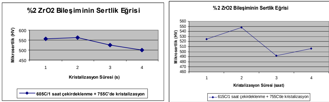
Şekil 7.23: 605°C ve 615°C’de Çekirdeklendirme, 755°C’de Kristalizasyon Isıl İşlemi Uygulanan M7A3 (%2 ZrO 2 ) Grubu Numunelerin Zamana Bağlı Sertlik Değerleri
