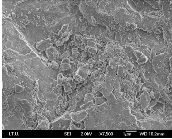
Şekil 7.25: ZrO_2 İçermeyen Numunenin Yapay Vücut Sıvısı İçerisinde 1 Gün Bekletildikten Sonraki Yüzey Görüntüsü
