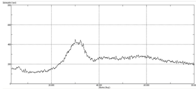
Şekil 7.6: M7A3 (%0 ZrO 2 ) Bileşimine Ait XRD Diyagramı 600°C/1s
