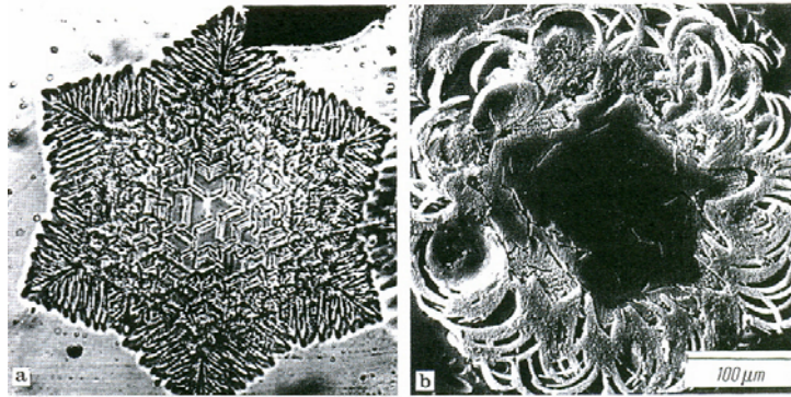
Şekil 4.17: (a) Teknik Camdaki Korderit Kristal Hatası (b) Bükülmüş Phlogopite Mika Kristallerindeki Kordierit Kristalleri [18]
