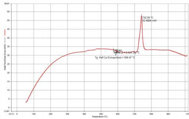
Şekil 7.5: M7A3 (%8 ZrO 2 ) Bileşimine Ait DTA Eğrisi
