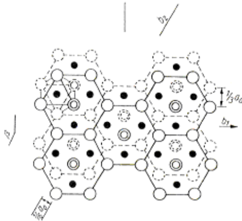
Şekil 4.11: Phlogopite Yapısındaki (001) Düzleminin Şematik Gösterimi [18]
