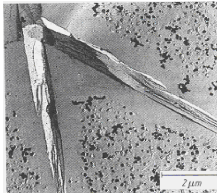
Şekil 4.7: Şekil 4.6’da Verilen Cama 980°C’de Isıl İşlem Uygulanmasıyla Elde Edilen Büyük Sodyum Phlogopite Kristalleri [18]
