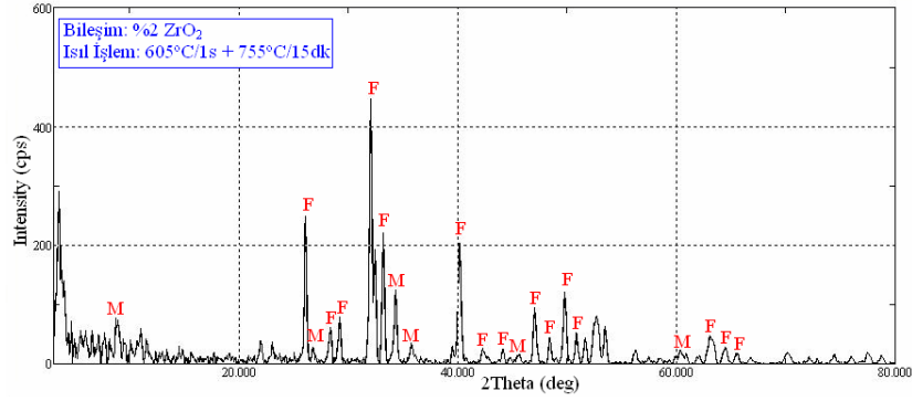
Şekil 7.11: M7A3 (%2 ZrO 2 ) Bileşimine Ait XRD Diyagramı 605°C/1s+755°C/15dk M: K-Mika, F: Florapatit
