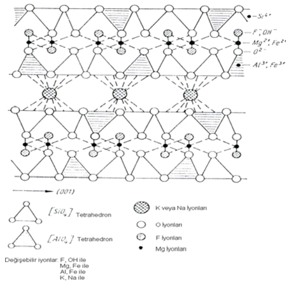
Şekil 4.9: Phlogopite Yapısının Şematik Gösterimi [18]
