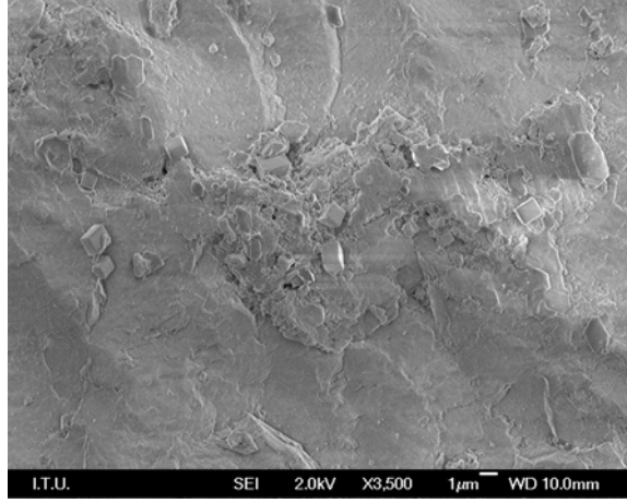
Şekil 7.24: ZrO_2 İçermeyen Numunenin Yapay Vücut Sıvısı İçerisinde 1 Saat Bekletildikten Sonraki Yüzey Görüntüsü
