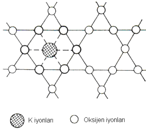
Şekil 4.10: Phlogopite Yapısının Küçük Bir Parçasının Şematik Gösterimi [18]
