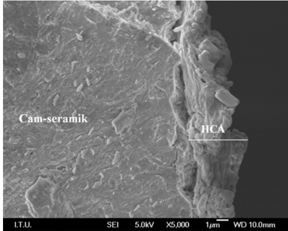
Şekil 7.29: ZrO 2 İçermeyen Numunenin Yapay Vücut Sıvısı İçerisinde 4 Hafta Bekletildikten Sonraki Kesit Görüntüsü
