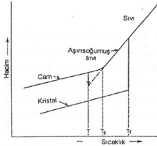
Şekil 2.1: Camsı, Sıvı ve Katı Haller Arasındaki İlişki [2]
