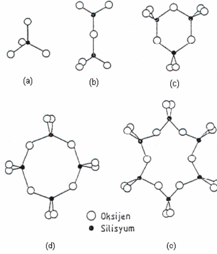
Şekil 2.2: Silikat Yapıları İçin Çeşitli Anyon Grupları (a) \text{SiO}_4^{4-} , (b) \text{Si}_2\text{O}_7^{6-} , (c) \text{Si}_3\text{O}_9^{6-} (d) \text{Si}_4\text{O}_{12}^{8-} , (e) \text{Si}_6\text{O}_{18}^{12-} [3]
