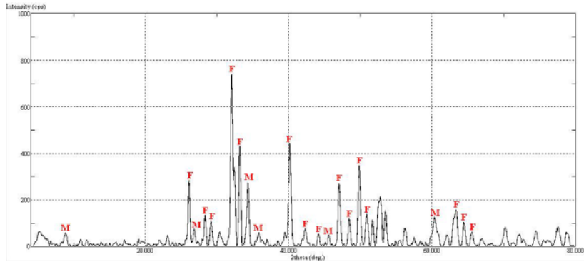
Şekil 7.15: M7A3 (%8 ZrO 2 ) Bileşimine Ait XRD Diyagramı 600°C/1s + 750°C/1s
