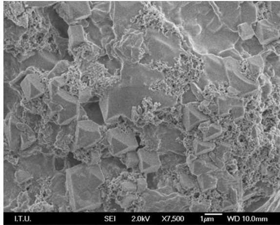
Şekil 7.27: Ağırlıkça %1 ZrO_2 İçeren Numunenin Yapay Vücut Sıvısı İçerisinde 2 Hafta Bekletildikten Sonraki Yüzey Görüntüsü
