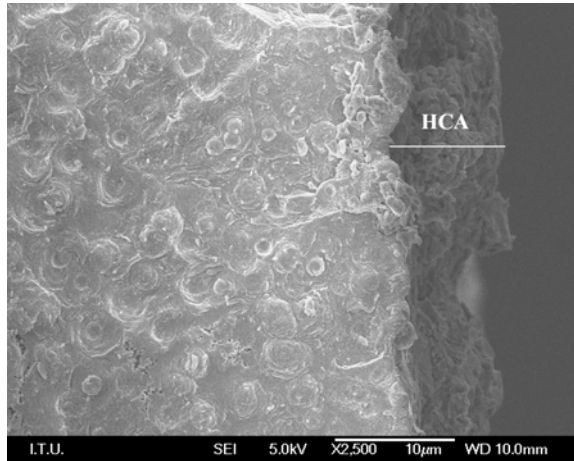
Şekil 7.31: Ağırlıkça %2 ZrO_2 İçeren Numunenin Yapay Vücut Sıvısı İçerisinde 4 Hafta Bekletildikten Sonraki Kesit Görüntüsü
