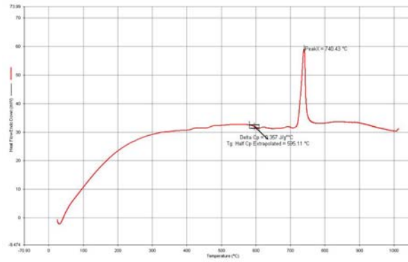
Şekil 7.4: M7A3 (%4 ZrO 2 ) Bileşimine Ait DTA Eğrisi
