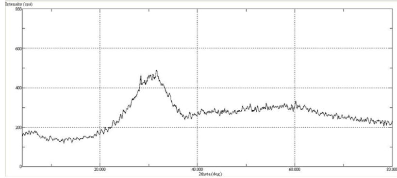
Şekil 7.14: M7A3 (%8 ZrO 2 ) Bileşimine Ait XRD Diyagramı 600°C/1s
