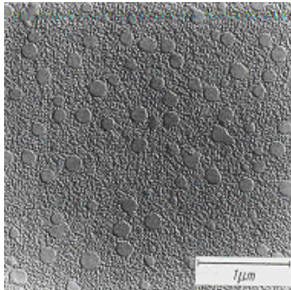
Şekil 4.3: Şekil 4.2'deki MAS Sistemindeki Camın %11,2 Mol Oksijen İyonunun Flor İyonuyla Yer Değiştirmesi Sonucunda Oluşan Mikroyapı Görüntüsü [18]
