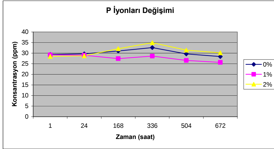
Şekil 7.34: Numunelere Ait Çözeltilerdeki Fosfor İyonlarının Değişimi
