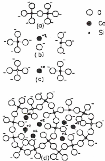
Şekil 2.4: SiO 2 ile CaO Arasındaki Reaksiyon ve Bu Reaksiyon ile Oluşan Camın Yapısı [4]. (a) SiO 2 Yapısı, (b) CaO' in Yapıya Girmesi, (c) CaO' in Oksijen Bağını Koparması, (d) Ca 2+ İyonlarının Hollere Yerleşmesi [5]
