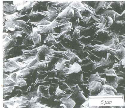
Şekil 4.4: F ve %5,2 Mol Na_2O İlave Edilmiş MgO-Al_2O_3-SiO_2 Bileşimindeki Camın Mikroyapı Görüntüsü [18]
