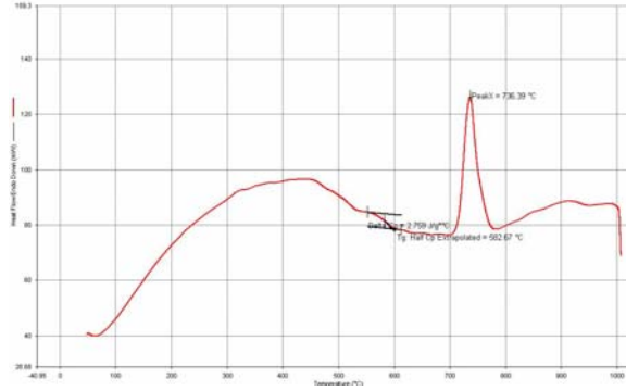
Şekil 7.2: M7A3 (%1 ZrO 2 ) Bileşimine Ait DTA Eğrisi
