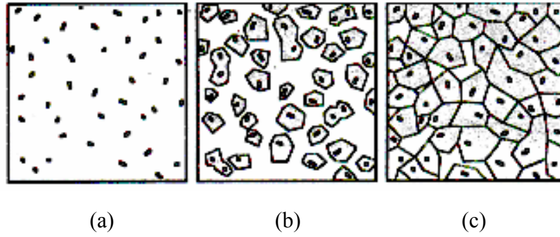
Şekil 3.1: Camdan Cam-Seramik Oluşumu (a) Çekirdek Oluşumu, (b) Kristal Oluşumu, (c) Cam-Seramik Mikroyapısı [7].
