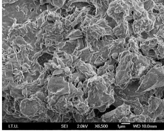
Şekil 7.26: ZrO_2 İçermeyen Numunenin Yapay Vücut Sıvısı İçerisinde 1 Hafta Bekletildikten Sonraki Yüzey Görüntüsü
