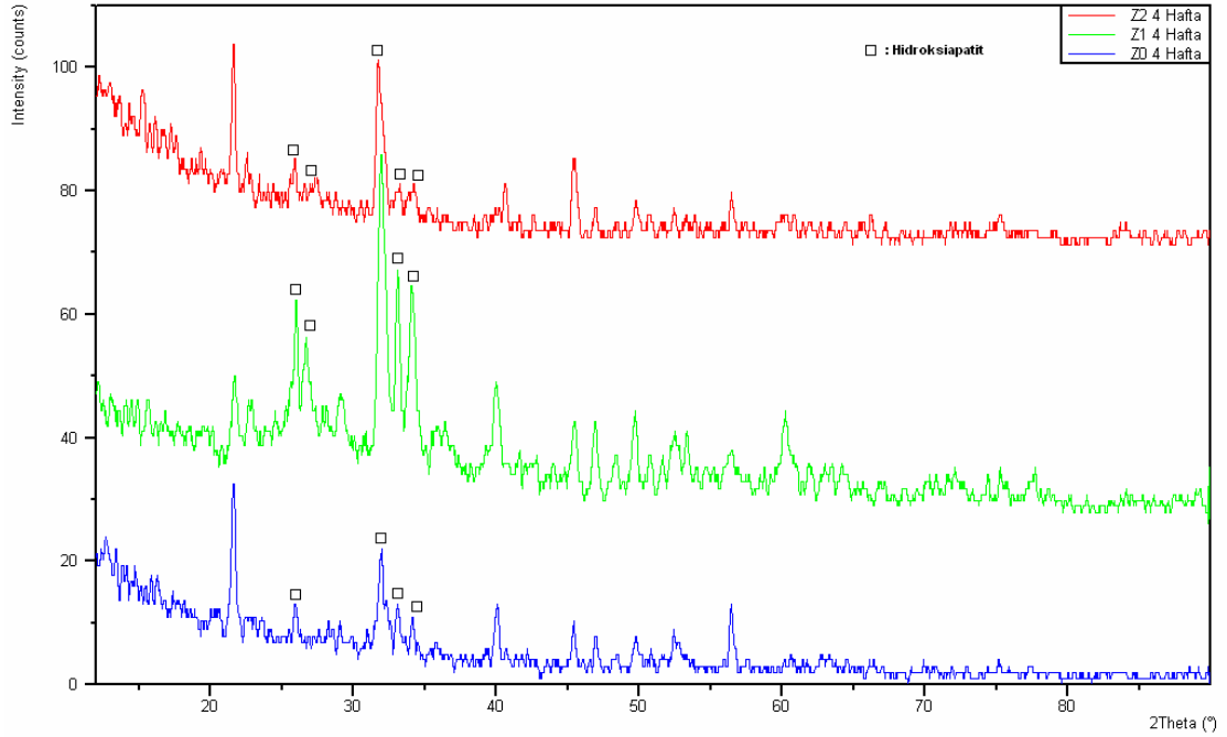
Şekil 7.32: 4 Hafta SBF İçinde Bekletilmiş M7A3 (%0 ZrO 2 , %1 ZrO 2 %2 ZrO 2 ) Bileşimine Sahip Numunelerin TF-XRD Analizi Sonuçları
