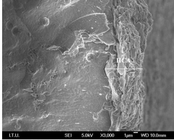
Şekil 7.30: Ağırlıkça %1 ZrO_2 İçeren Numunenin Yapay Vücut Sıvısı İçerisinde 4 Hafta Bekletildikten Sonraki Kesit Görüntüsü
