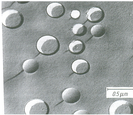
Şekil 4.19: Yüksek Miktarda CaO/P 2 O 5 Eklenmiş Ana Camın Hızlı Soğutulmasından Sonraki Karışmaz Yapı [7]
