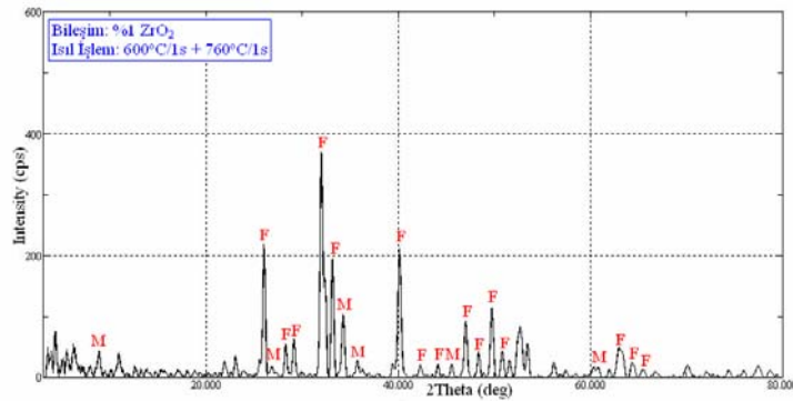
Şekil 7.9: M7A3 (%1 ZrO 2 ) Bileşimine Ait XRD Diyagramı 600°C/1s + 760°C/1s M: K-Mika F: Florapatit
