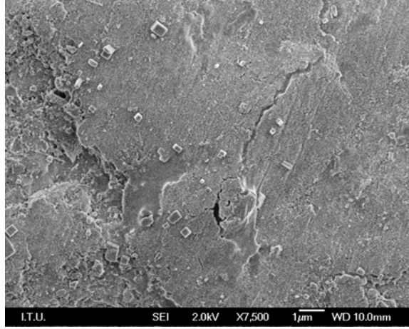
Şekil 7.28: Ağırlıkça %2 ZrO 2 İçeren Numunenin Yapay Vücut Sıvısı İçerisinde 2 Hafta Bekletildikten Sonraki Yüzey Görüntüsü
