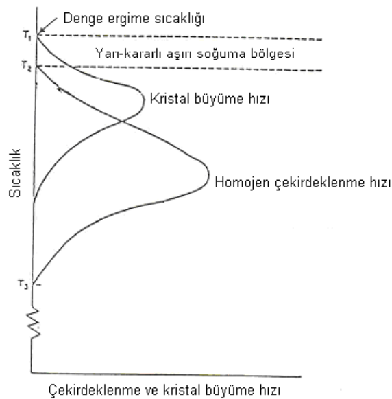
Şekil 3.3: Viskoz Bir Sıvı İçin Homojen Çekirdeklenme ve Büyüme Hızları [10]
