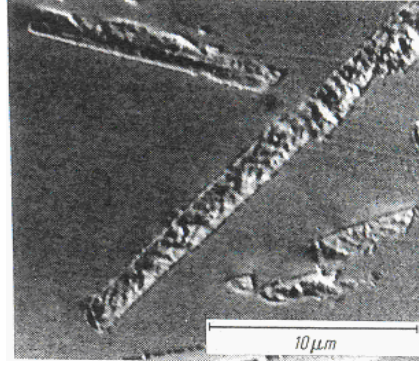
Şekil 4.12: Uzun Süre Isıl İşlem Görmüş Camdaki Na-phlogopite Kristalleri [18]
