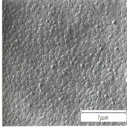
Şekil 4.2: MAS Sistemindeki Camdan MgO ve Al 2 O 3 'ce Zenginleştirilmiş Droplet Fazın Çökmesi [18]
