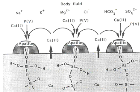
Şekil 5.1: CaO-SiO 2 İçeren Bir Cam-Seramikte Yüzeyde Apatit Oluşumunun Şematik Gösterimi [24]
