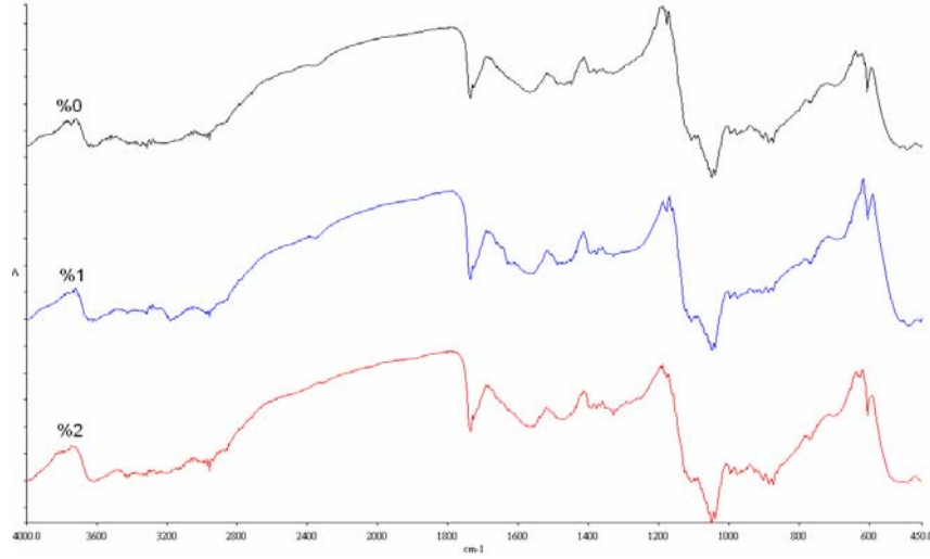
Şekil 7.33: Yapay Vücut Sıvısı İçerisinde 4 Hafta Bekletilmiş ZrO_2 İçermeyen, Ağırlıkça %1 ve %2 Oranlarında ZrO_2 İçeren Numunelerin FTIR Analizi Sonuçları
