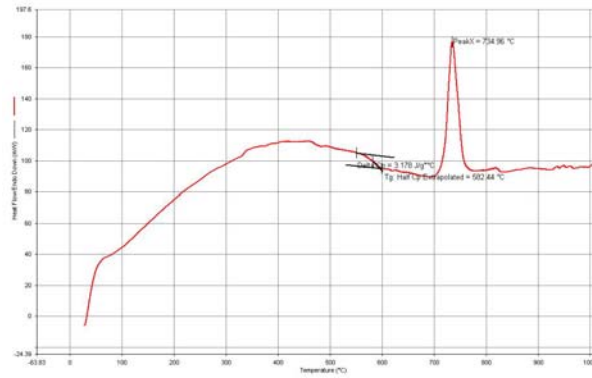
Şekil 7.3: M7A3 (%2 ZrO 2 ) Bileşimine Ait DTA Eğrisi
