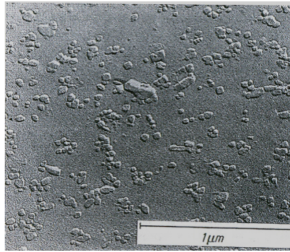
Şekil 4.6: Şekil 4.5’de Verilen Camın Tekrar Isıtılarak 780°C’de Sellaite ( \text{MgF}_2 ) ve Norbergite ( 2\text{MgO} \cdot \text{SiO}_2 \cdot \text{MgF}_2 )’nin Kristalizasyonu [18]
