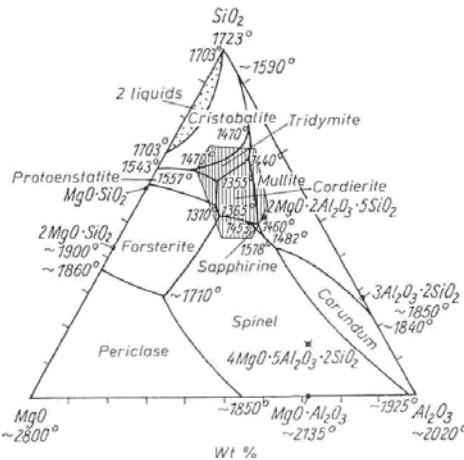
Şekil 4.1: \text{MgO-Al}_2\text{O}_3\text{-SiO}_2 Sisteminde Ait Faz Diyagramı [18]
