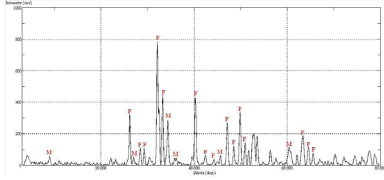
Şekil 7.13: M7A3 (%4 ZrO 2 ) Bileşimine Ait XRD Diyagramı 600°C/1s + 750°C/1s M: K-Mika F: Florapatit
