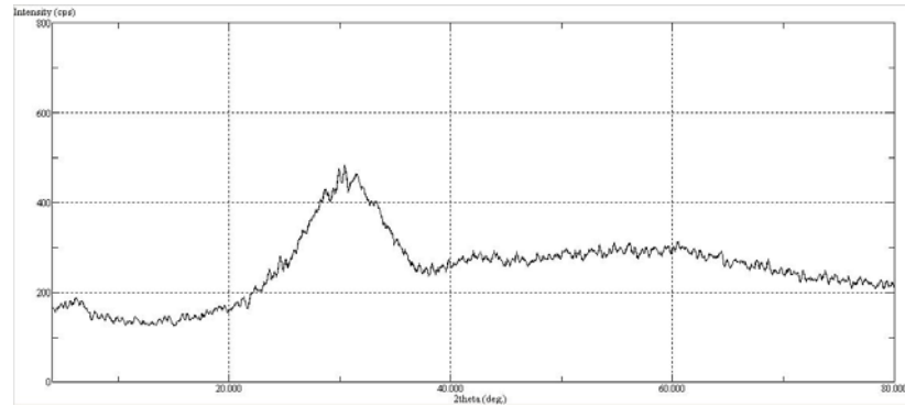
Şekil 7.12: M7A3 (%4 ZrO 2 ) Bileşimine Ait XRD Diyagramı 600°C/1s
