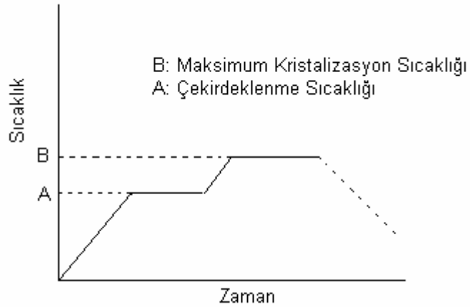
Şekil 3.5: Cam Seramiklerin Isıl İşlemi [12]
