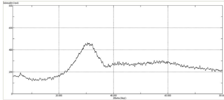
Şekil 7.8: M7A3 (%1 ZrO 2 ) Bileşimine Ait XRD Diyagramı 600°C/1s
