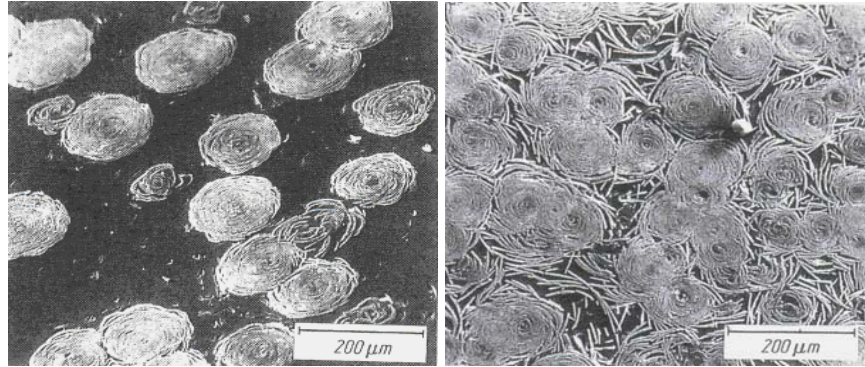
Şekil 4.13-4.14: Phlogopite Kristallerinin Küresel Lamelli Düzeni [18]
