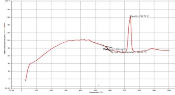
Şekil 7.1: M7A3 (%0 ZrO 2 ) Bileşimine Ait DTA Eğrisi
