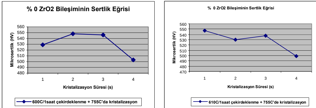
Şekil 7.21: 600°C ve 610°C’de Çekirdeklendirme, 755°C’de Kristalizasyon Isıl İşlemi Uygulanan M7A3 (%0 ZrO 2 ) Grubu Numunelerin Zamana Bağlı Sertlik Değerleri.
