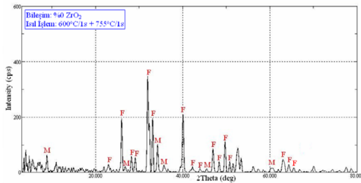
Şekil 7.7: M7A3 (%0 ZrO 2 ) Bileşimine Ait XRD Diyagramı 600°C/1s + 755°C/1s M: K-Mika F: Florapatit
