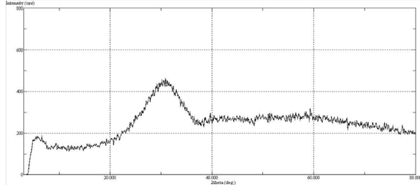
Şekil 7.10: M7A3 (%2 ZrO 2 ) Bileşimine Ait XRD Diyagramı 605°C/1s
