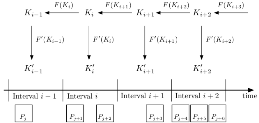
Şekil 4.5 : \mu Tesla protokolü şeması.
