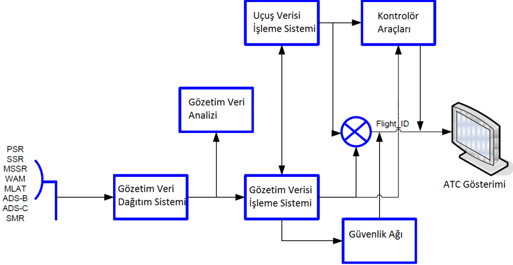
Şekil 1.8 : ATC gözetim sistemi
