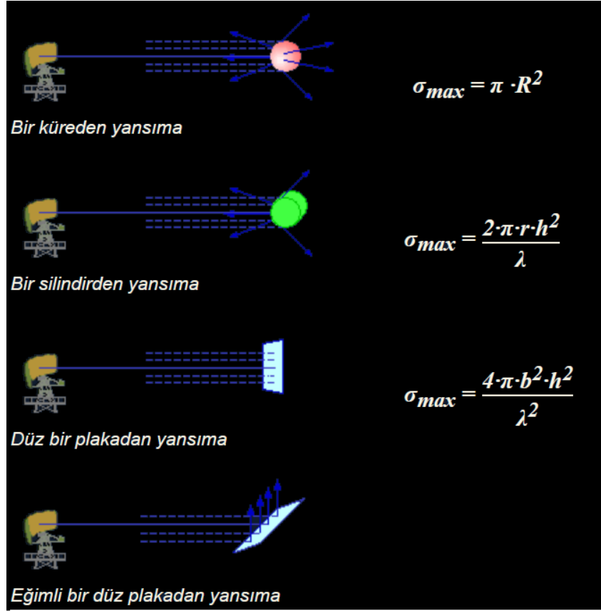
Şekil 1.5 : Radar yansıma çeşitleri.
