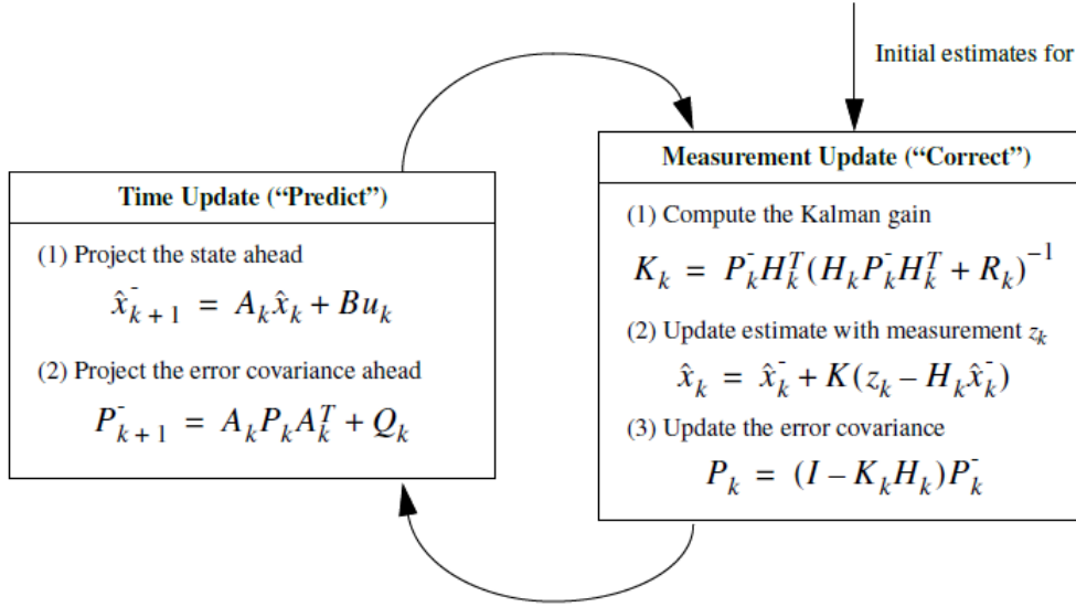
Şekil 4.15 : Kalman Filtre Şeması.
