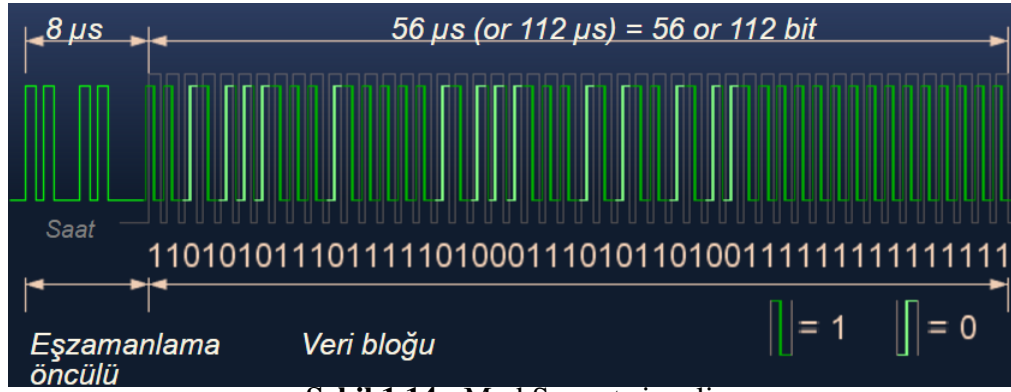
Şekil 1.14 : Mod S yanıt sinyali.
