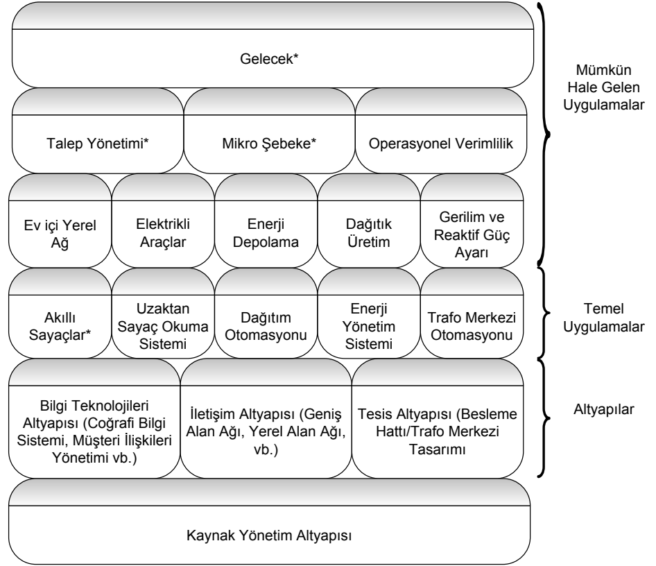
Şekil 2.1: Akıllı Şebeke'nin genel alt başlıkları [20]
