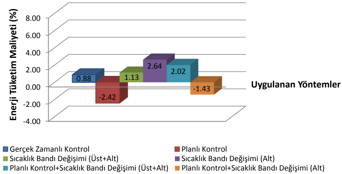
Şekil 7.10: A sınıfı buzdolabının yıllık elektrik faturasındaki değişim yüzdesi
