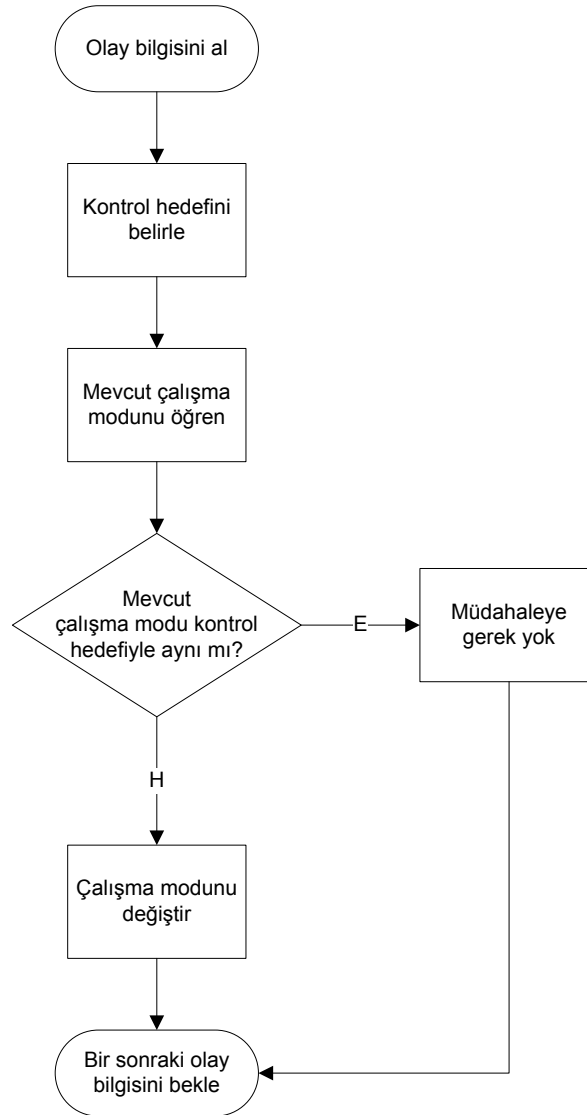
Şekil 7.2 : Gerçek Zamanlı Kontrol yönteminin çalışma mantığı
