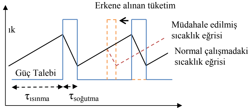
Şekil 4.2 : Bir soğutucu için erken tüketim örneği
