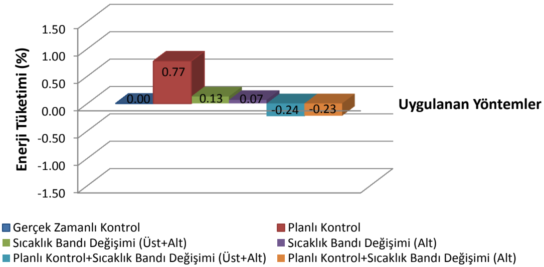
Şekil 7.9 : G sınıfı buzdolabının yıllık tüketimindeki değişim yüzdesi
