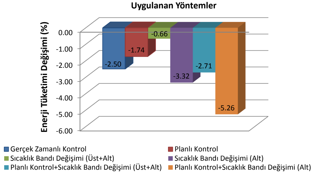
Şekil 7.4 : A sınıfı buzdolabı için şebekeden çekilen enerjideki değişim yüzdesi
