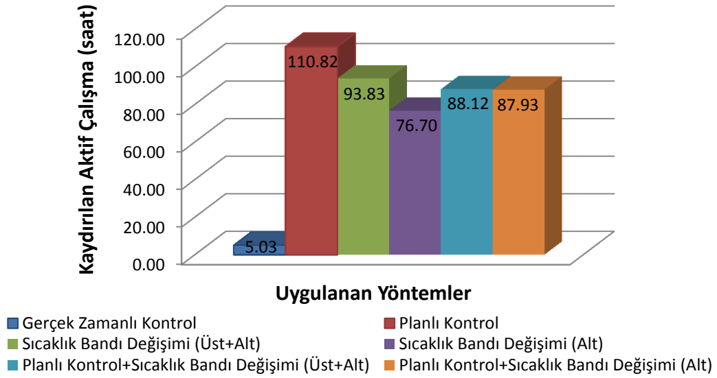
Şekil 7.7 : G sınıfı buzdolabı için yeterli üretim zamanlarına kaydırılan çalışma
