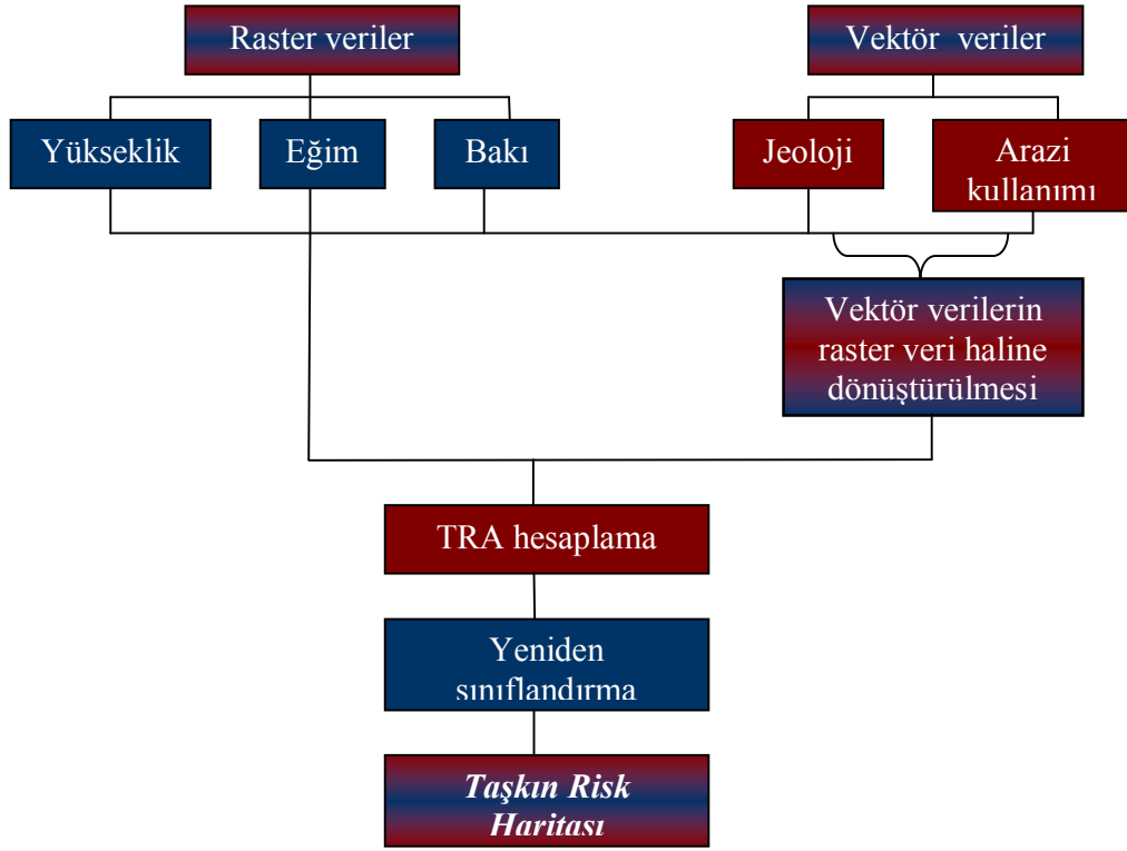
Şekil 3.1 : TRA yazılımı AHP yöntemi akış şeması.
