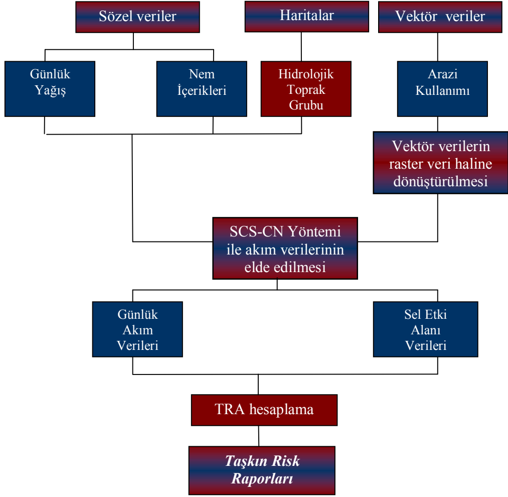
Şekil 3.2 : TRA yazılımı InfoDif yöntemi akış şeması.
