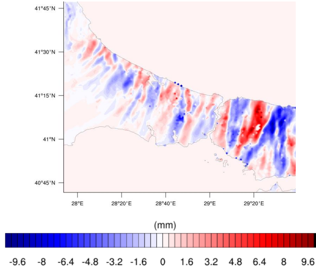
Şekil 3.48 : 02.02.2012 00 UTC fiziksel kar kalınlığı fark haritası.
