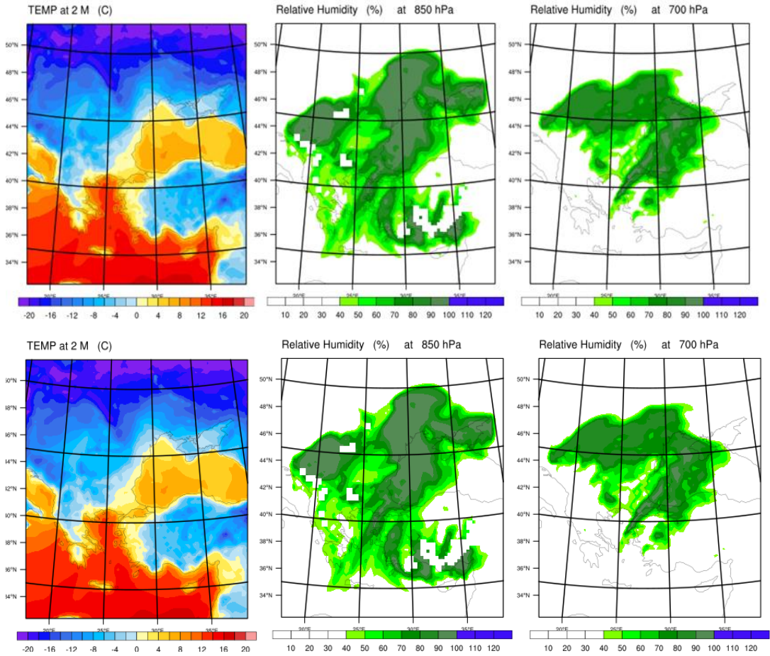
Şekil 3.11 : 24.01.2000 06 UTC'ye ait gerçek altlık ile hazırlanan haritalar 2m sıcaklık (üstte solda), 850 mb nem (üstte ortada), 700mb nem (üstta sağda) 24.01.2000 06 UTC'ye ait düzenlenmiş altlık ile hazırlanan haritalar 2m sıcaklık (altta solda), 850 mb nem (altta ortada), 700mb nem (altta sağda).
