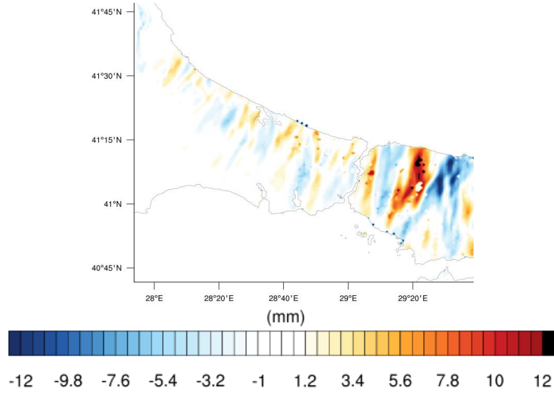
Şekil 3.49 : 02.02.2012 00 UTC kar su eşleniği fark haritası.
