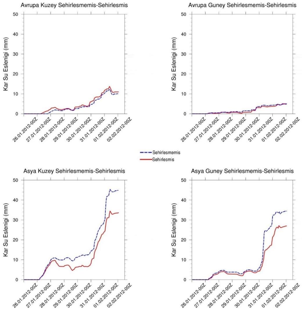
Şekil 3.45 : 2012 yılı Avrupa Kuzey (üste solda), Avrupa Güney (üstte sağda), Asya Kuzey (alta solda), Asya Güney (altta sağda) şehirleşmemiş-şehirleşmiş noktaları kar su eşleniği zaman serileri.
