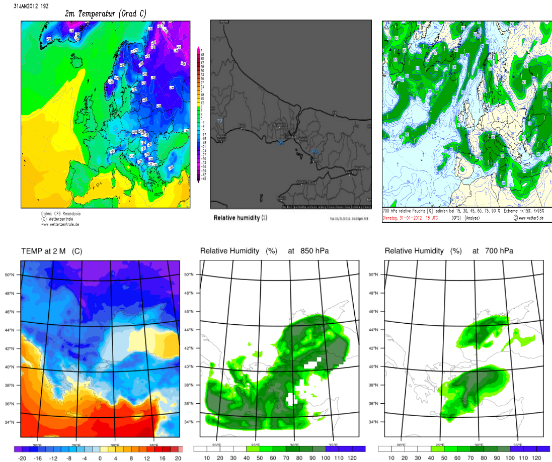
Şekil 3.38 : 31.01.2012 18 UTC gözlem haritaları, 2m sıcaklık (üstte solda), 850 mb nem (üstte ortada), 700 mb nem (üstte sağda) 31.01.2012 18 UTC model haritaları, 2m sıcaklık (altta solda), 850 mb nem (altta ortada), 700 mb nem (altta sağda).
