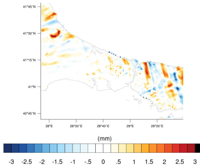
Şekil 3.21 : 25.01.2000 kar su eşleniği haritası fark haritası
