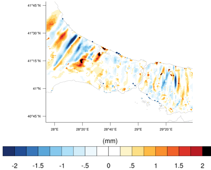
Şekil 3.34 : 24.01.2004 00 UTC kar su eşleniği fark haritası.
