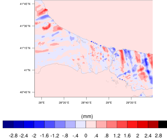
Şekil 3.20 : 25.01.2000 fiziksel kar kalınlığı fark haritası.
