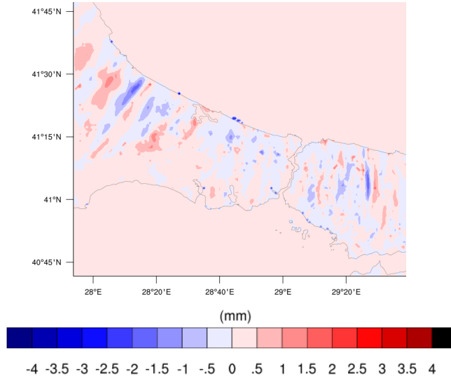
Şekil 3.33 : 24.01.2004 00 UTC fiziksel kar kalınlığı fark haritası.
