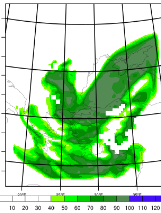
Şekil 3.8 : 25.01.2000 15 UTC gözlem haritaları, 2m sıcaklık (üstte solda), 850 mb nem-18 UTC (üstte ortada), 700 mb nem (üstte sağda), 25.01.2000 15 UTC model haritaları, 2m sıcaklık (altta solda), 850 mb nem (altta ortada), 700 mb nem (altta sağda).
