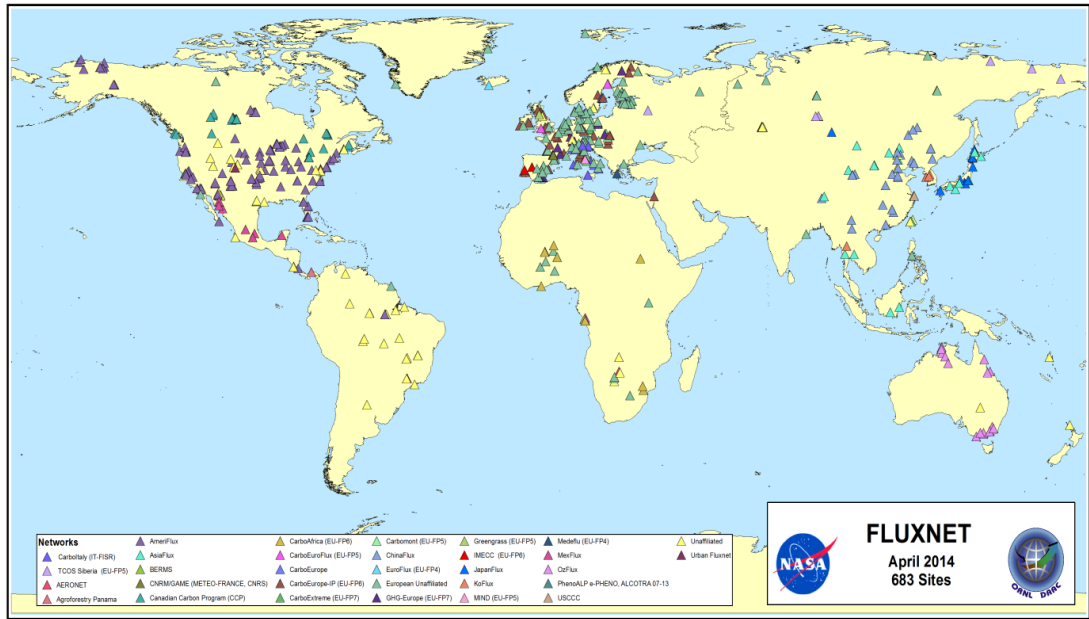
Şekil 1.2: Nisan 2014 itibariyle FLUXNET Ölçüm Ağı ( http://fluxnet.ornl.gov/sites/default/files/FluxnetNetwork4-2014.png ).
