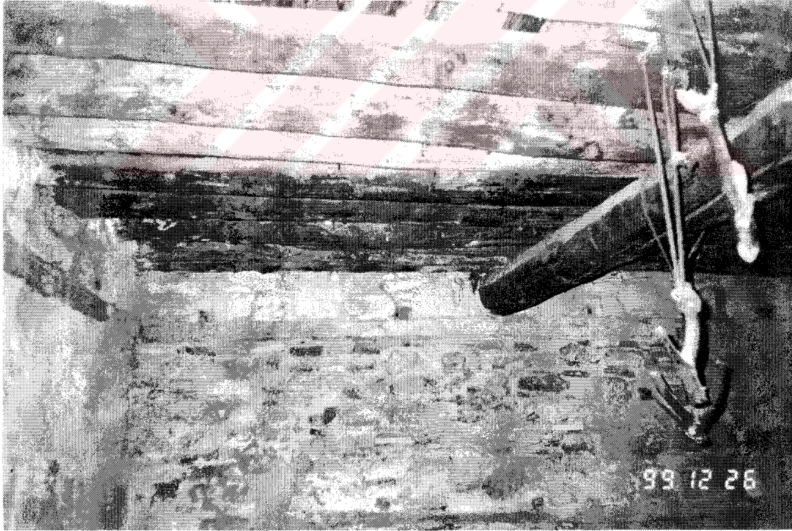
Şekil D64. Selamlık bölümü, soğuk depo (Z04) batı duvarı ve taşıyıcı sistemi (1999)
