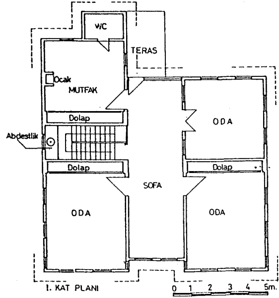
Şekil F142. Isparta, Gazi Kemal Mahallesi, Hacı Ethem Sokak, No:16'daki konutun birinci kat planı, abdestlik (Urfalıoğlu, 1995)
