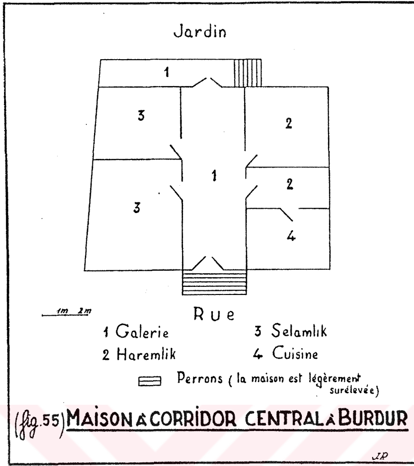
Şekil F1. Burdur’da merkezi koridorlu plan tipi (Planholl, 1958)
