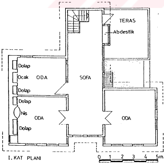
Şekil F143. Isparta, Gazi Kemal Mahallesi, Akarçeşme Sokak, No:3'deki konutun birinci kat planı, abdestlik (Urfalıoğlu, 1995)
