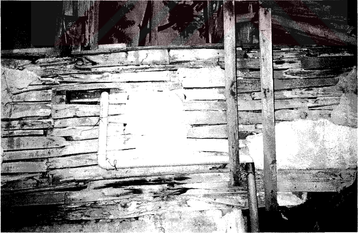
Şekil D186. Selamlık bölümü, P12-P13-P14 pencereleri altındaki ahşap strüktür (2000)
