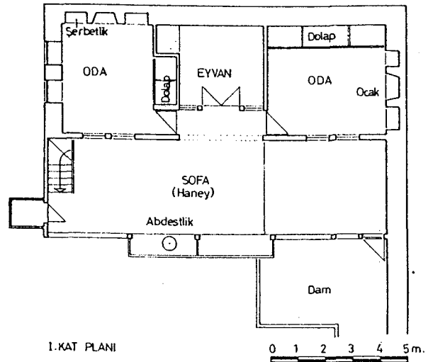
Şekil F144. Isparta, İskender Mahallesi, Şehit Fethi Bey Sokak, No:16'daki konutun birinci kat planı, abdestlik (Urfalıoğlu, 1995)
