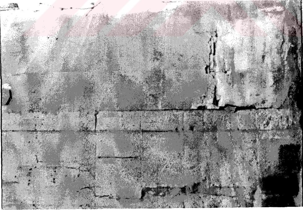
Şekil D181. Selamlık bölümü, avlu girişi taş yüzeyde çimentolu onarımlar ve duvar yüzeyinde şişme
