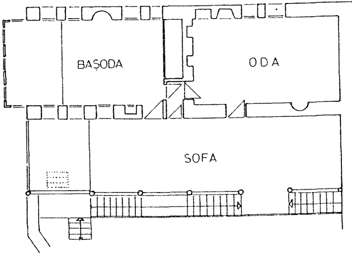
Şekil F6. Bakibey Konağı (Kocaoda) birinci kat planı (Urfalıoğlu, 1995)
