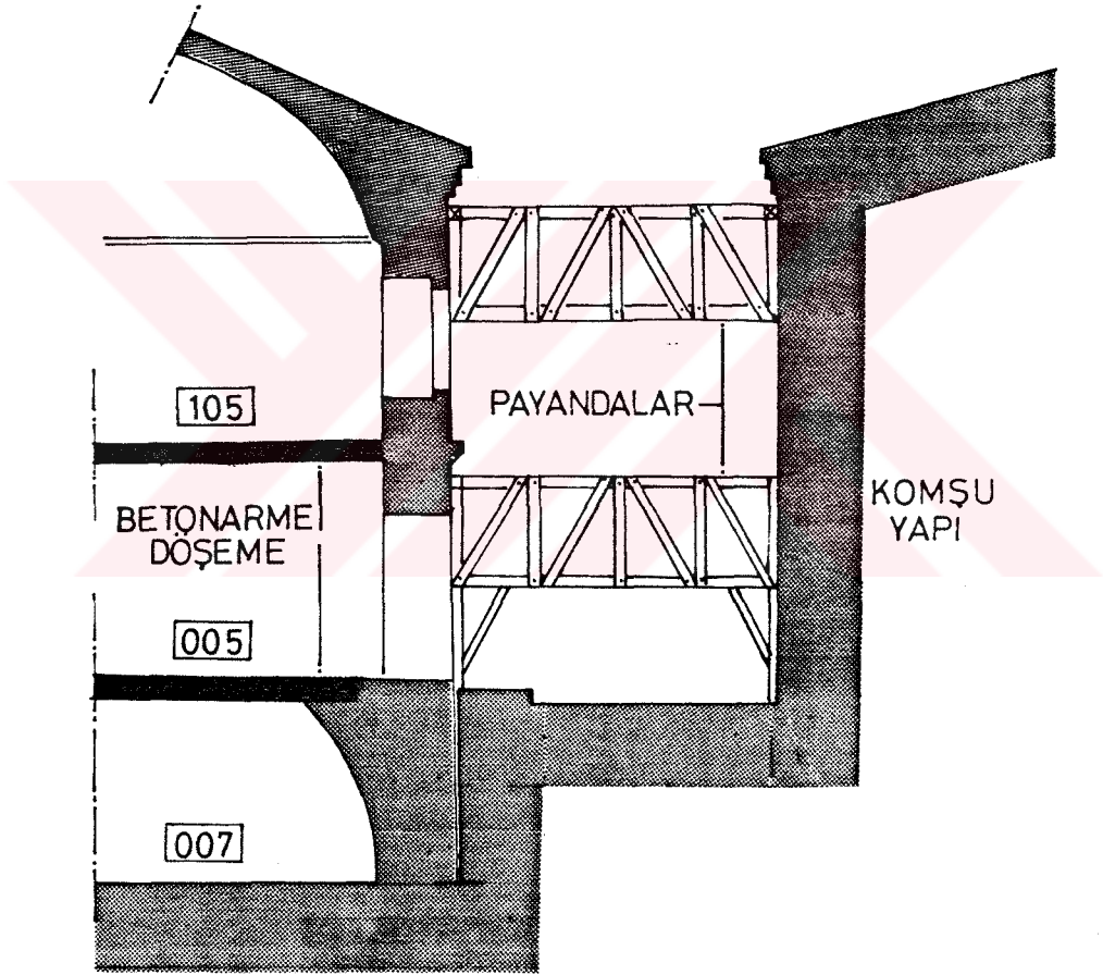
b) Perşembe Pazarı Caddesi Cephesinin Desteklenmesi, Kesit 1/100
