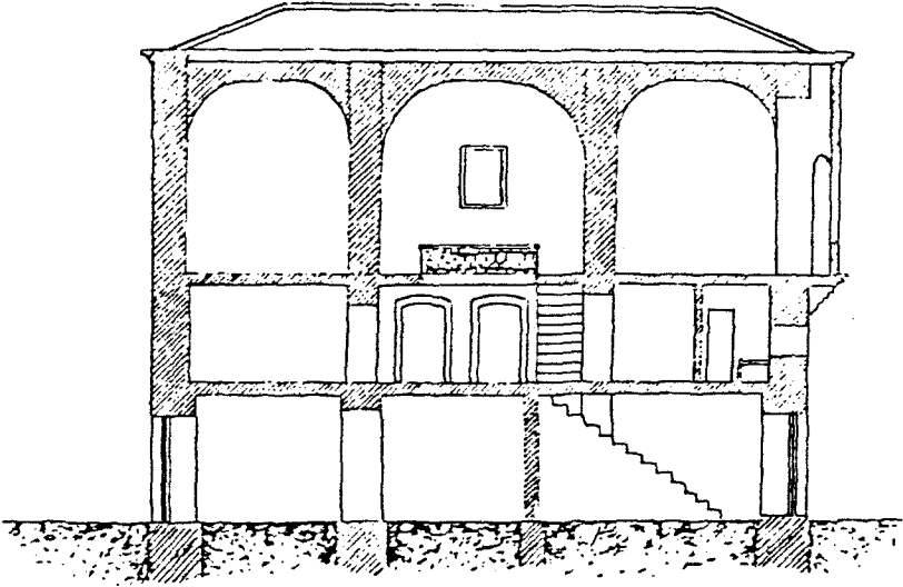
ŞEKİL 21. Kesit Krokisi (Arseven, C.E.)
