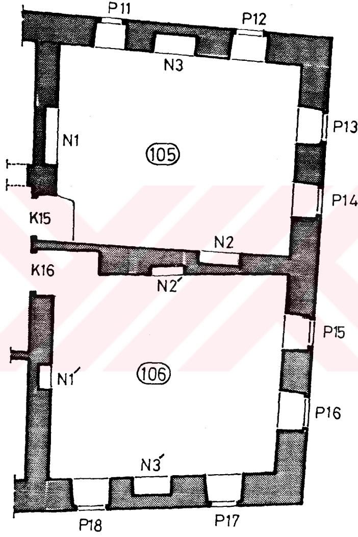
ŞEKİL 15. 105 ve 106 No.lu Üst Kat Mekanlarının Karşılaştırılması
