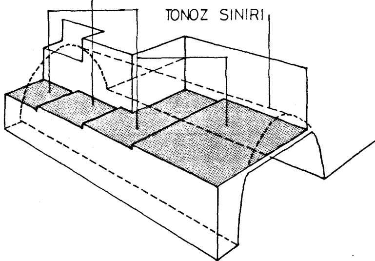
ŞEKİL 14. Saksı Han'ın Perşembe Pazarı Caddesi Cephesindeki Dükkânların Teşkili İçin Bozulan Tonoz Yapısının Şeması YENİDEN TEŞKİL EDİLMİŞ NİTELİKSİZ BETONARME DÖSEMELER
