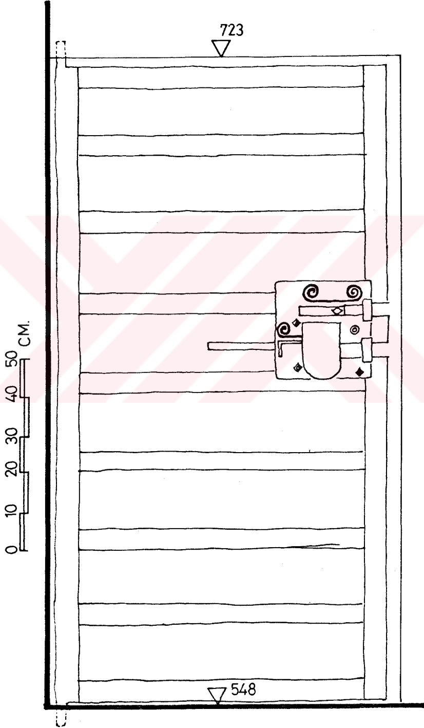
ŞEKİL 24. 201 nolu mekanın kapısı
