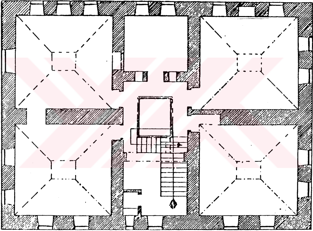
ŞEKİL 19. Saksı Han'ın 20.yy.'ın başındaki durumunu gösteren üst kat planı (Arseven, C.E.)
