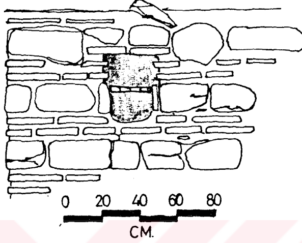
ŞEKİL 22. a) Kuş Kōşkü no:1 rölöve
