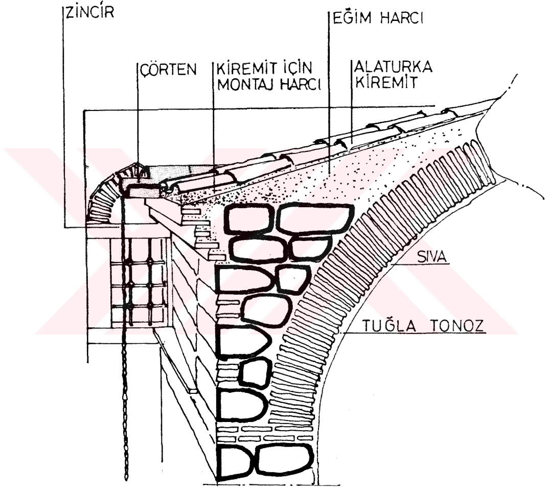
ŞEKİL 28. a) Çatı ve Saçak Detayı, restorasyon
