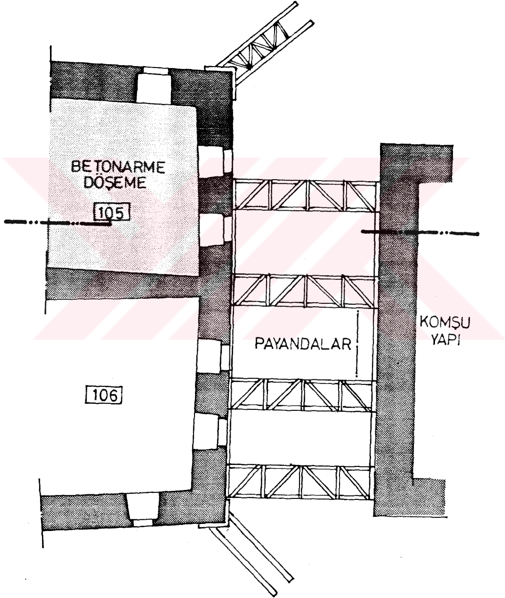
ŞEKİL 33. a) Perşembe Pazarı Caddesi Cephesinin desteklenmesi, Plan 1/100
