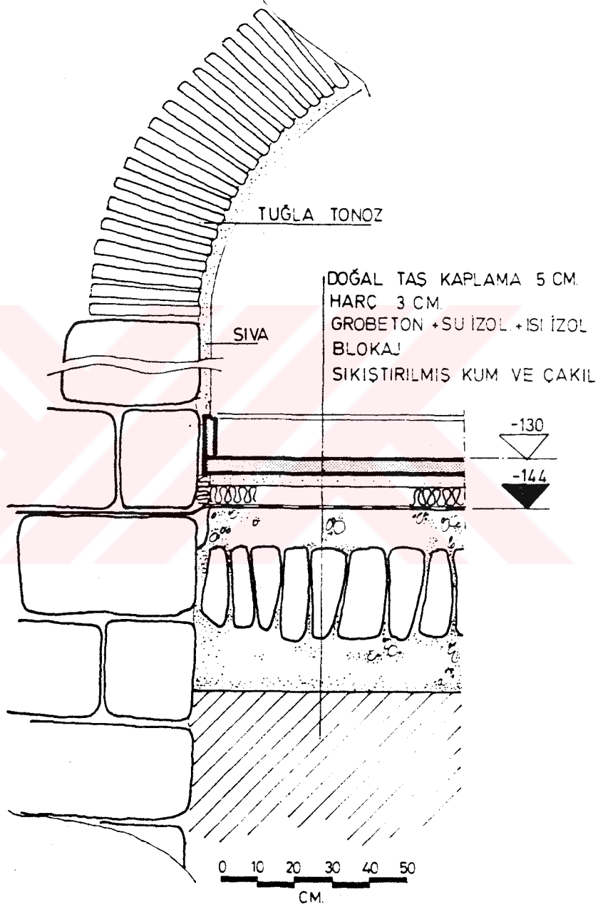
ŞEKİL 30. Zemin Kat Döşemesi, restorasyon
