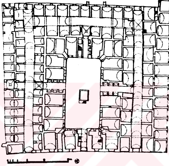
ŞEKİL 27. Kızlarağası Han'ı üst kat planı
