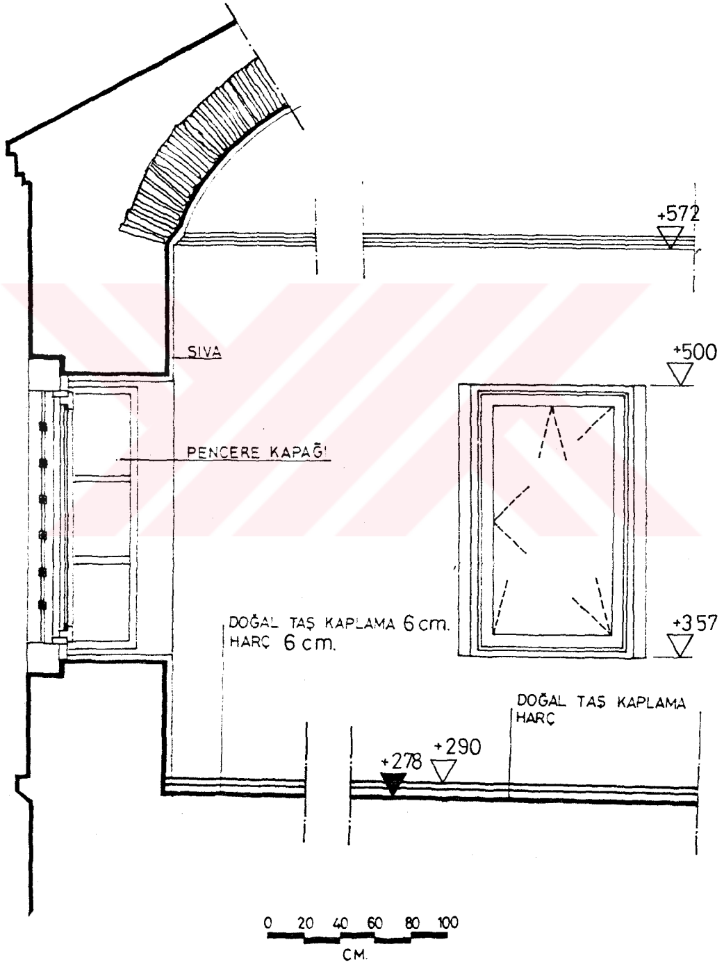
ŞEKİL 31. Üst Kat Penceresi ve döşemesi, restorasyon
