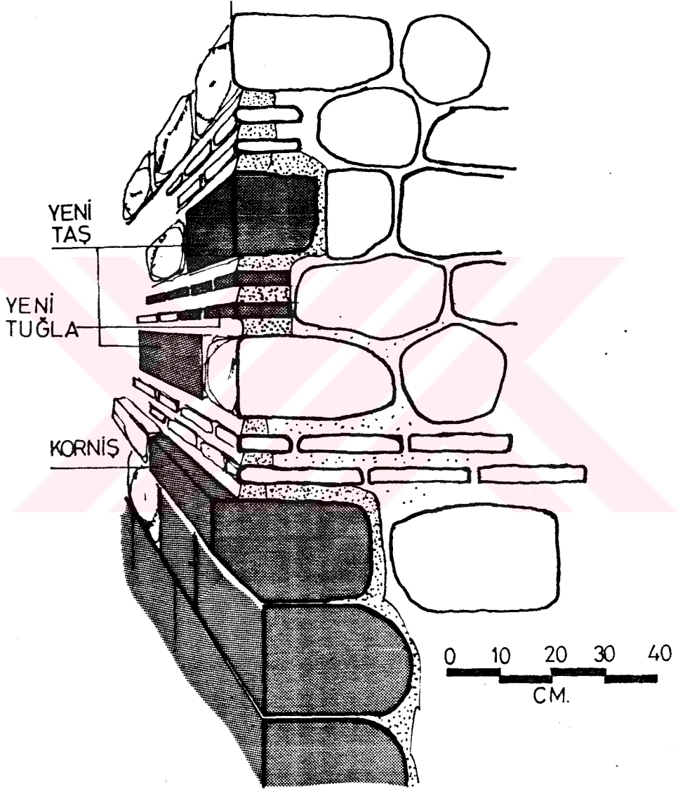
ŞEKİL 29. Taş Değiştirme detayı, restorasyon
