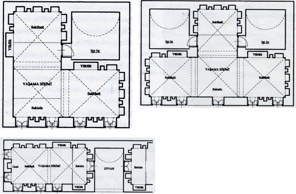
Şekil 4 17: Geleneksel Mardin evinde yaşama birimi Kaynak: F. Aioğlu, 2000.
