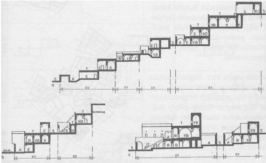
Şekil 4.15: Geleneksel Evlerin Araziye Yerleşimi Kaynak: F. Ai o ğ lu, 2000.
