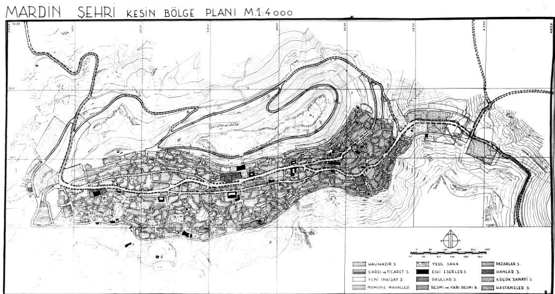
Şekil 3.12: N. Ve T. Pertev tarafından yapılan ilk Mardin İnar Planı
