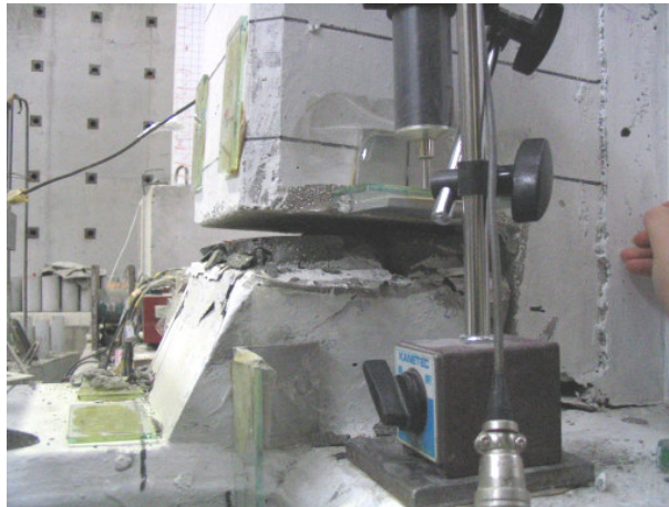
Şekil A. 5 Karma numune #1 döşeme kısmı basınç halinde iken kolon gusesi ile giriş açılması
