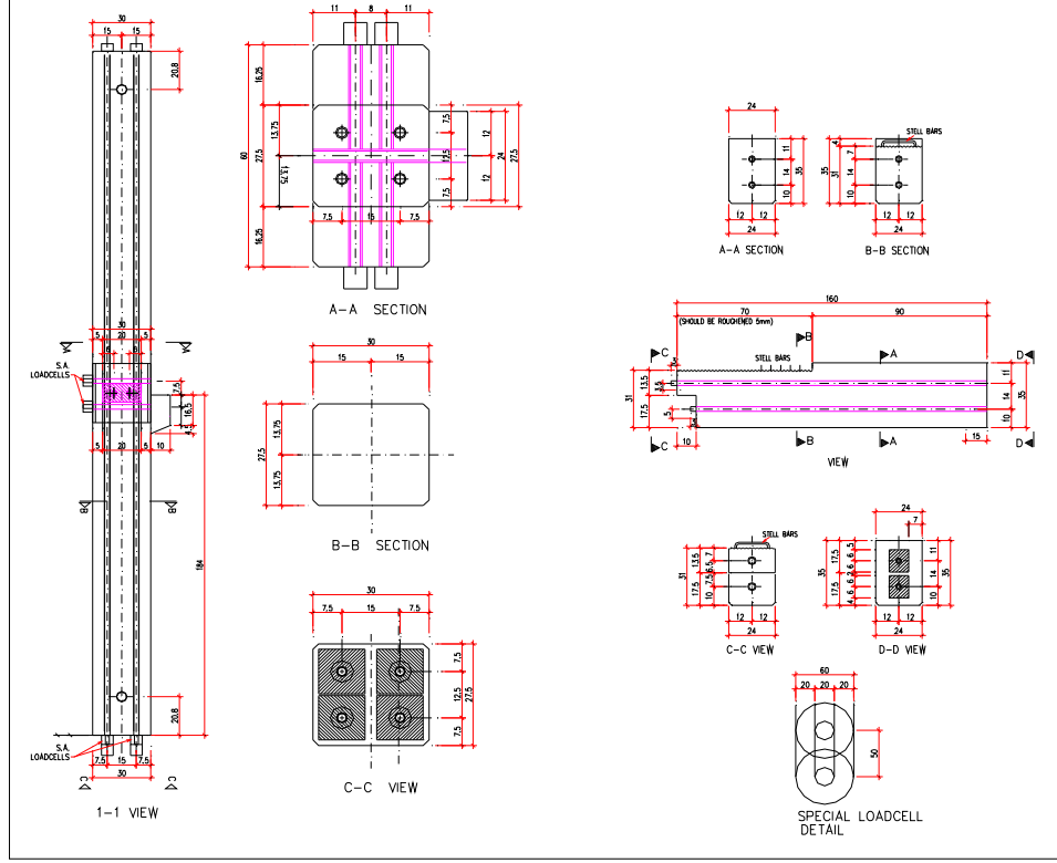
Şekil 3-7 : Karma numune donatı düzeni [5]
