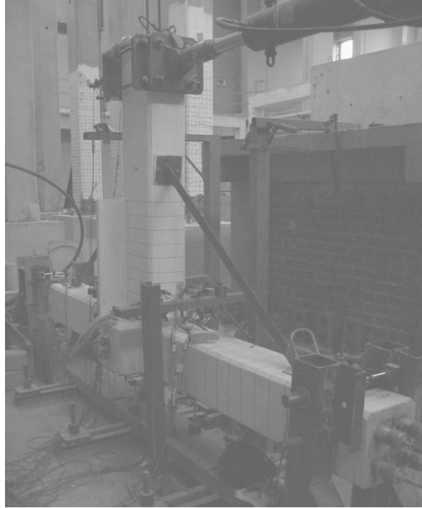
Şekil 3-13 : Karma numunesi
