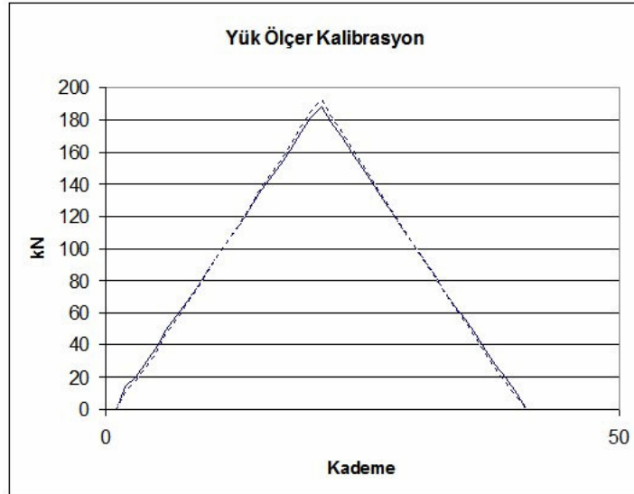
Şekil 3-26 : Yük ölçer ölçümleme
