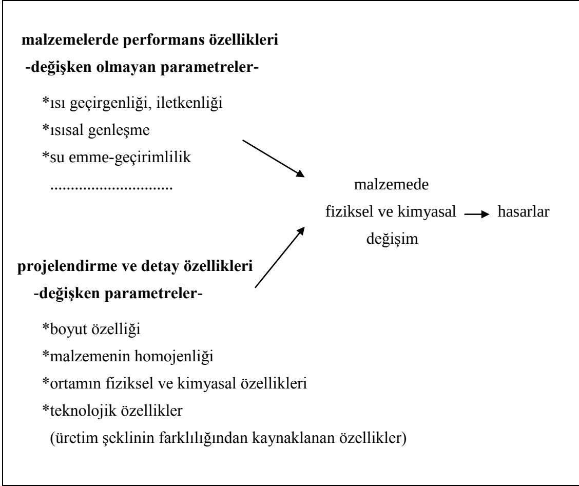
Şekil 2.1 Malzemede hasar oluşturan faktörler
