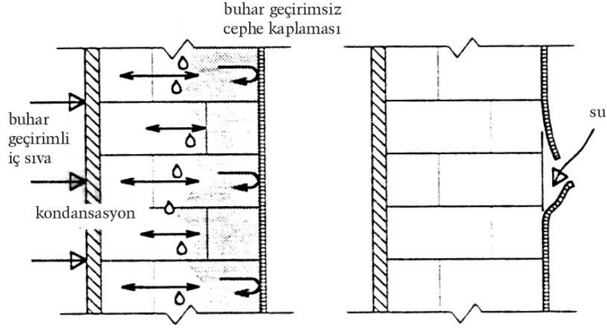
Şekil 4.27 Cephe kaplama malzemesinin buhar geçirimsizliği dolayısıyla yoğuşma [12]
