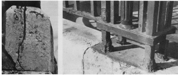
Şekil 3.2 Demirin korozyona uğraması sonucu, içine gömüldüğü taşa yarılmalara [39]
