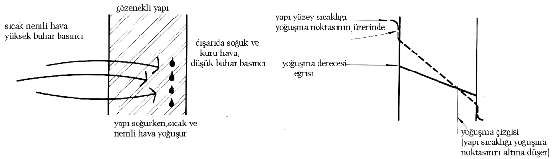
Şekil 4.20 İç yoğuşma [56]
