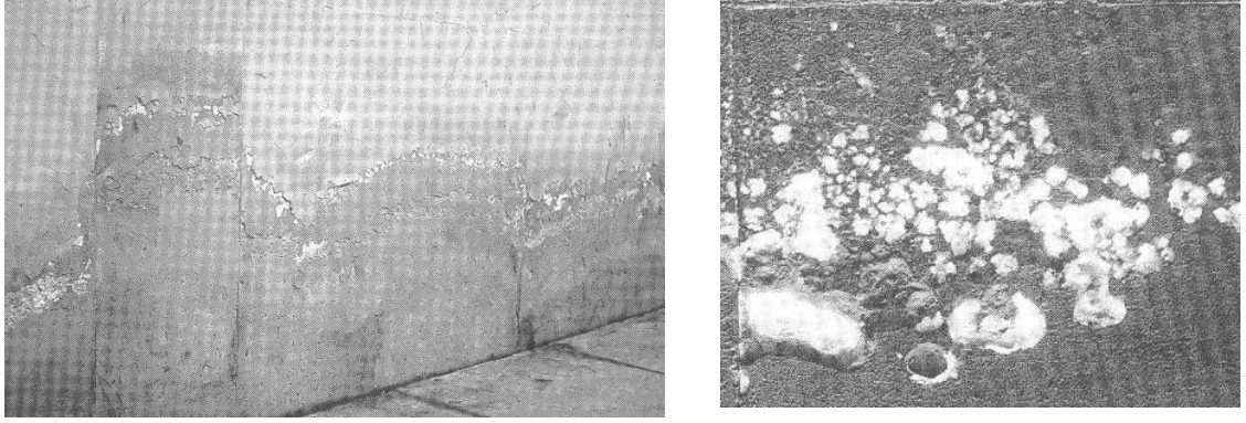
Şekil 4.23 Betonda çiçeklenme [30]
