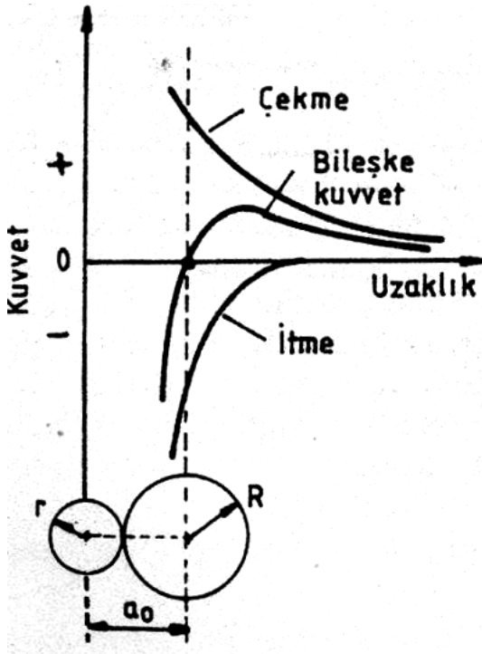
Şekil 2.5 Atomlararası kuvvetler [9]
