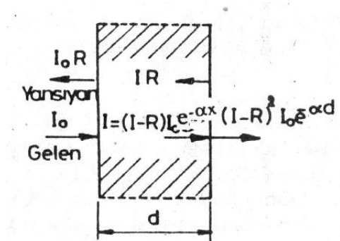
Şekil 2.13 Işığın emilmesi [9]
