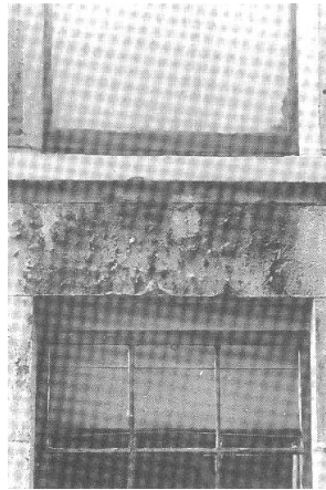
Şekil 3.1 Taşta sülfat etkisi sonucu oluşan bozulmalar [30]
