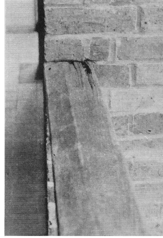
Şekil 4.8 Ahşap-tuğla ilişkisi [39]
