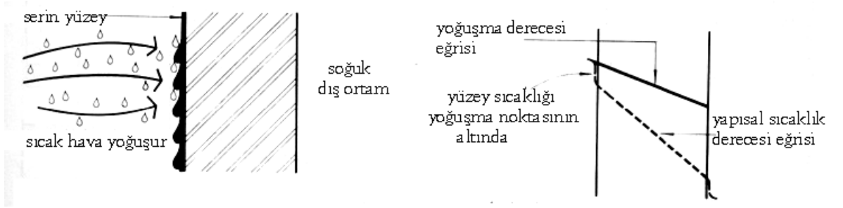
Şekil 4.15 Yüzey yoğuşması [56]
