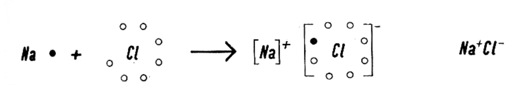
Şekil 2.2 Sodyum klorürde iyonik bağ oluşumu [10]
