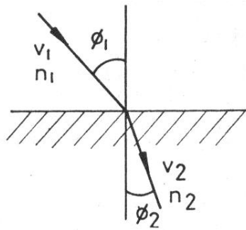
Şekil 2.14 Işık kırılması [9]
