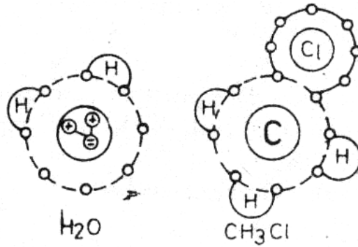
Şekil 2.4 Asimetrik moleküllerde elektriksel kutuplaşma oluşumu [9]
