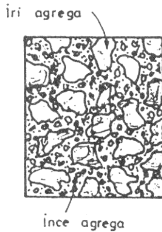
Şekil 3.3 Beton karışımının yapısı [9]
