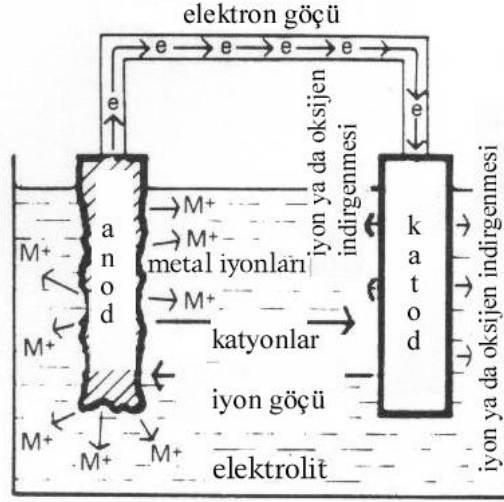
Şekil 2.15 Elektrokimyasal korozyon [30]
