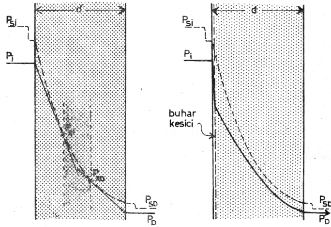
Şekil 4.29 Duvar kesitinde buhar kesicinin rolü [65]
