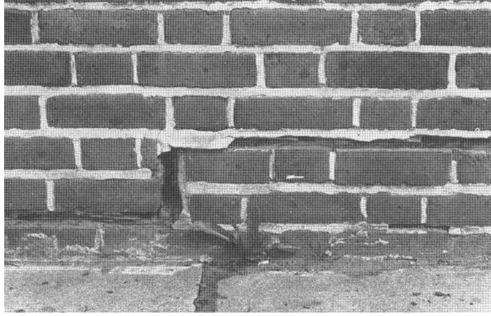
Şekil 4.22 Tuğla duvarda genleşme hasarı [10]
