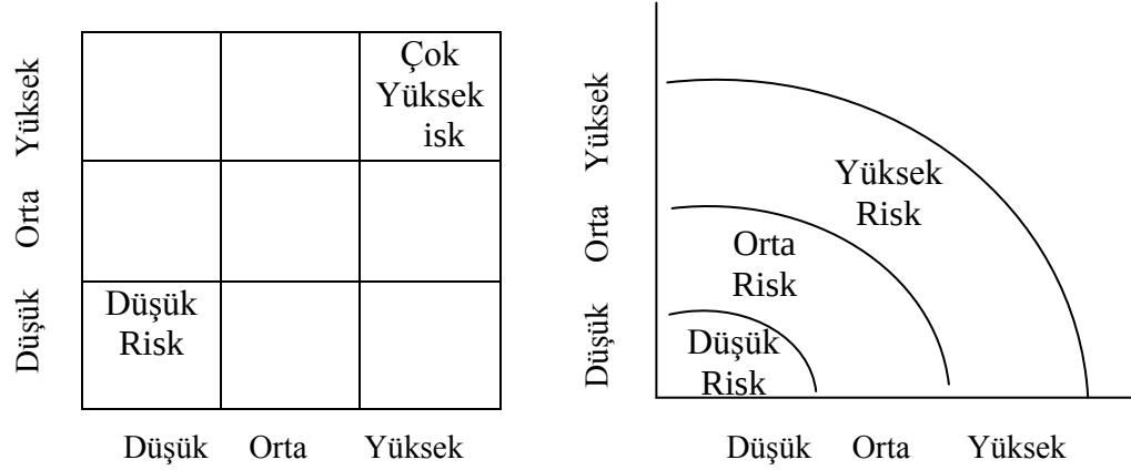
Şekil 4.4 : Oluşma olasılığı risk matrisi ve risk diyagramı (TS IEC 62198, 2003).
