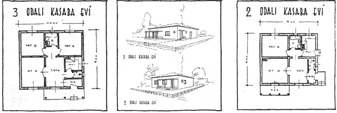
Şekil 4.14 Kasaba Evi planları, Mortaş, Abidin, 'Küçük Kasaba Evi Projesi', Arkitekt 1940, 10 vd.
