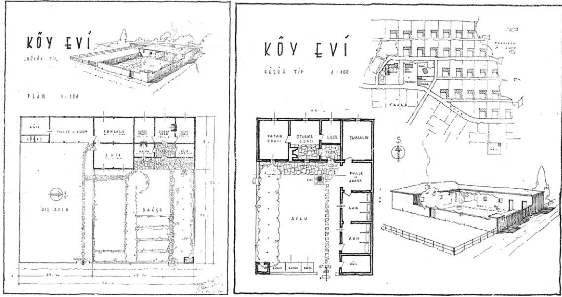
Şekil 4.12 Köy Evi planları, Mortaş, Abidin, 'Köy Evi Tipleri', Arkitekt 1940, 8 vd.
