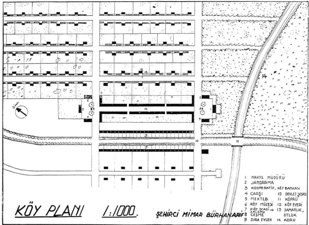
Şekil 4.5 Köy Planı, Mortaş, Abidin, 'Köy Projesi', Arkitekt 1935, 320
