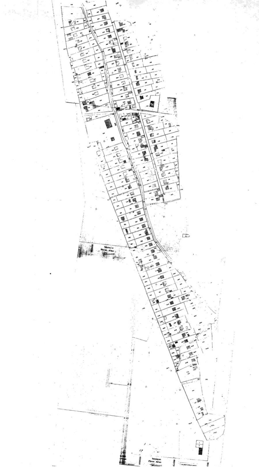
Şekil A.10 Yeşilbayır genel yerleşim planı Yeşilbayır Belediyesi İmar Müdürlüğü
