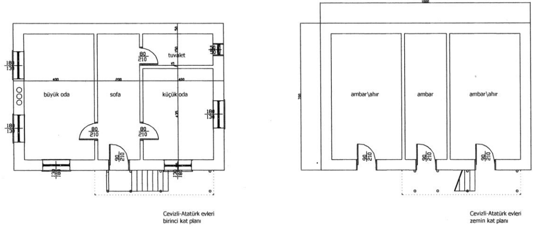
Şekil 4.19 Cevizli’de yapılan tip konutların planları, çizimler H. T. Örmecioğlu
