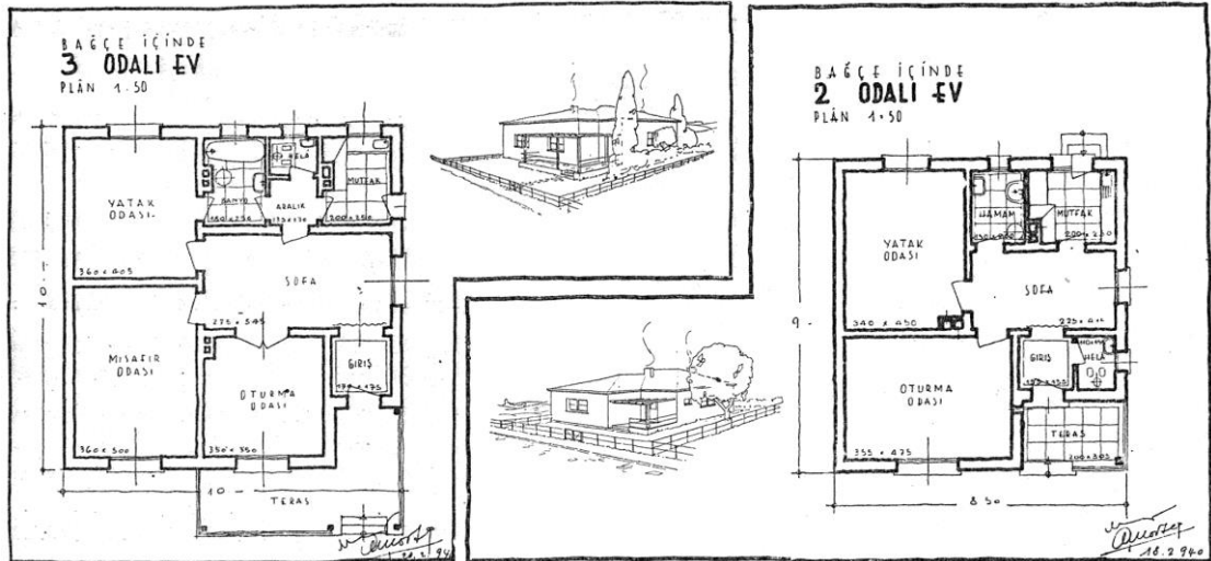
Şekil 4.13 Bahçe içinde ev planları, Mortaş, Abidin, 'Küçük Kasaba Evi Projesi', Arkitekt 1940, 10 vd.
