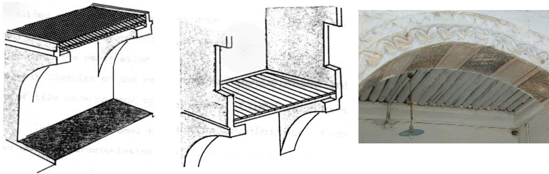
Şekil 6.5 Hezenin üstünde kat olduğu ve olmadığı durumları gösterir kesitler ve bir hezen örneği (A. Erençin, 1979, s: 26)
