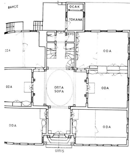
Şekil 7.14 Kayseri'de orta sofalı ev (Gündoğdu, 1986)
