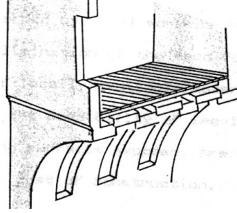
Şekil 6.7 Tonzun üstünde kat olduğu ve olmadığı durumları gösterir kesitler ve bir tonoz örneği (Erençin, 1979, s: 27 v.d.)
