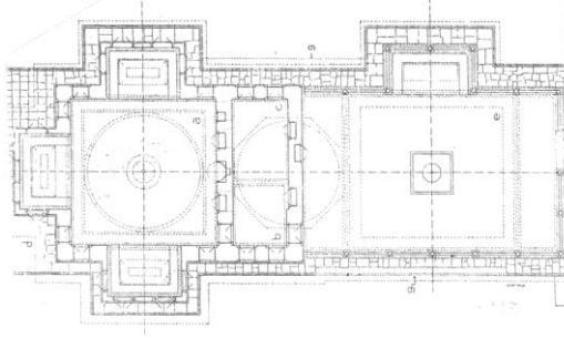
Şekil 7.11 Sepetçiler Köşkü planı (Eldem,1972) Şekil 7. 12 Sepetçiler Köşkü kesiti (Eldem,1972)
