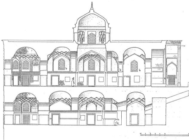
Şekil 7.9 Çinili Köşk, kesit (Eldem, 1969, rs: 39)
