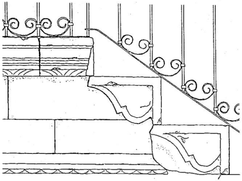
Şekil 6.10 Taş merdiven ile demir korkuluk görünüşü ve bir merdiven örneği (Berk, 1990, s:136)
