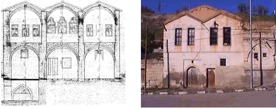
Şekil 6.8 Üçlü eğimli çatı kesiti ve ikili eğimli çatı örneği (Mustafapaşa Belediyesi)
