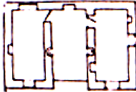
Şekil 4.7 Kahta, Damlacık’ta bir Hilani örneği (Akın, 1984, s: VIII)
