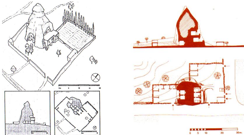
Şekil 4.4 Peri bacasına oyulmuş konut örneklerinin plan ve kesitleri (Stea, Turan, 1993, s: 226), (Giovannini, 1971, sf: 75)
