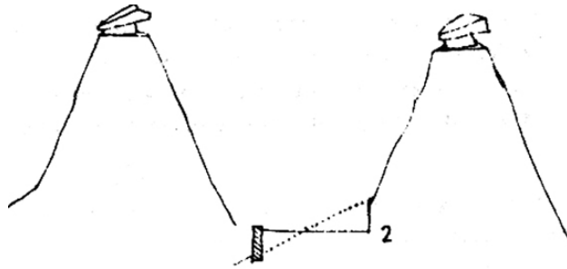
Şekil 6.9 Eğimli kaya zeminde temel yapımını gösteren kesit (Erençin, 1979, s: 24)
