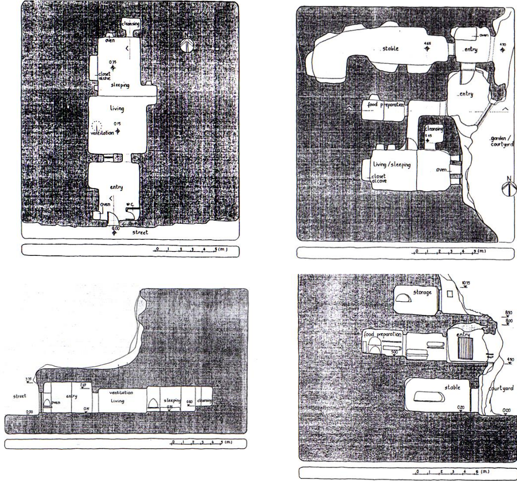
Şekil 4.3 Tek ve çok katlı oyma konut örneklerinin plan ve kesitleri (Stea, Turan, 1993, s: 227)
