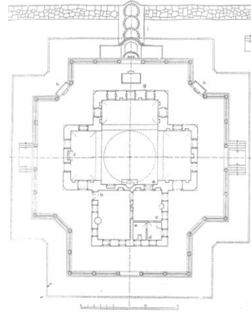
Şekil 7.10 Yalı Köşkü, plan (Eldem, 1969, rs: 132)
