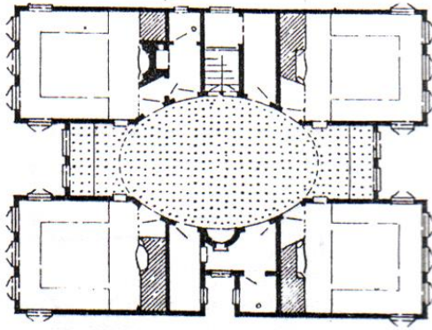
Şekil 7.13 Cihangir'de orta sofalı ev (Eldem, 1955)
