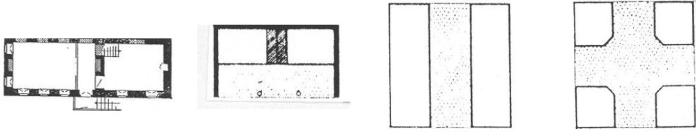
Sofasız plan şeması Dış sofalı plan şeması İç sofalı plan şeması Orta sofalı plan şeması Şekil 7.2 Sofanın konumuna göre Osmanlı evinde plan tipolojisi (Eldem, 1955, s: 25 v.d.)
