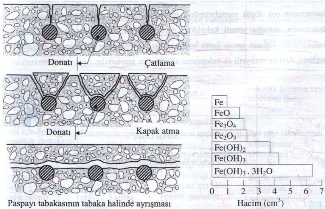
Şekil 2.30: Korozyon ürünlerinin hacimlerinin demire kıyasla gösterimi ve korozyon sonucu betonda görülen hasar çeşitleri
