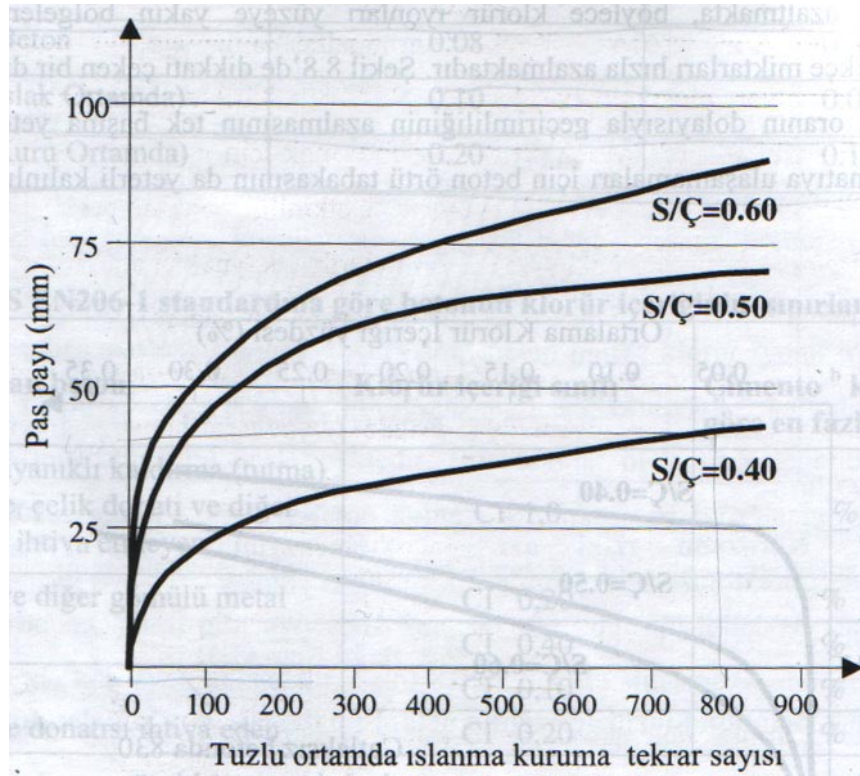
Şekil 2.26: Betonun klorür geçirirliliğine S/Ç oranının ve pas payı tabakasının kalınlığının etkisi
