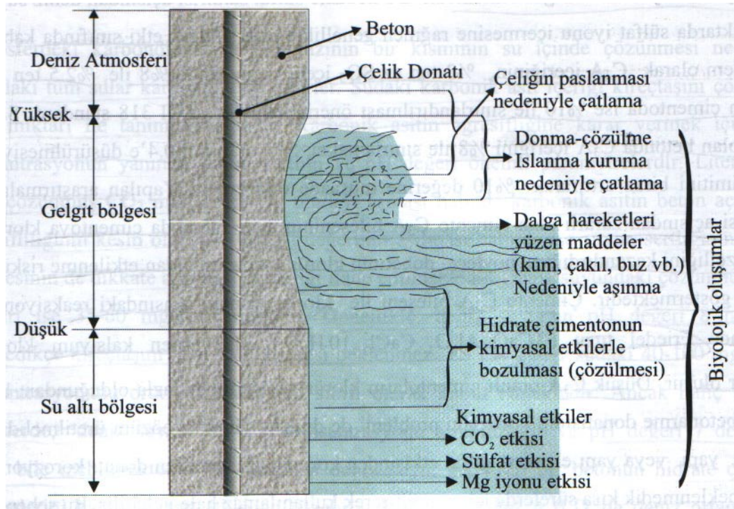
Şekil 2.15: Yapının bulunduğu konuma göre maruz kalabileceği değişik deniz ortamları ve betonarme bir elemanda deniz suyu etkisiyle oluşabilen bozulma mekanizmaları
