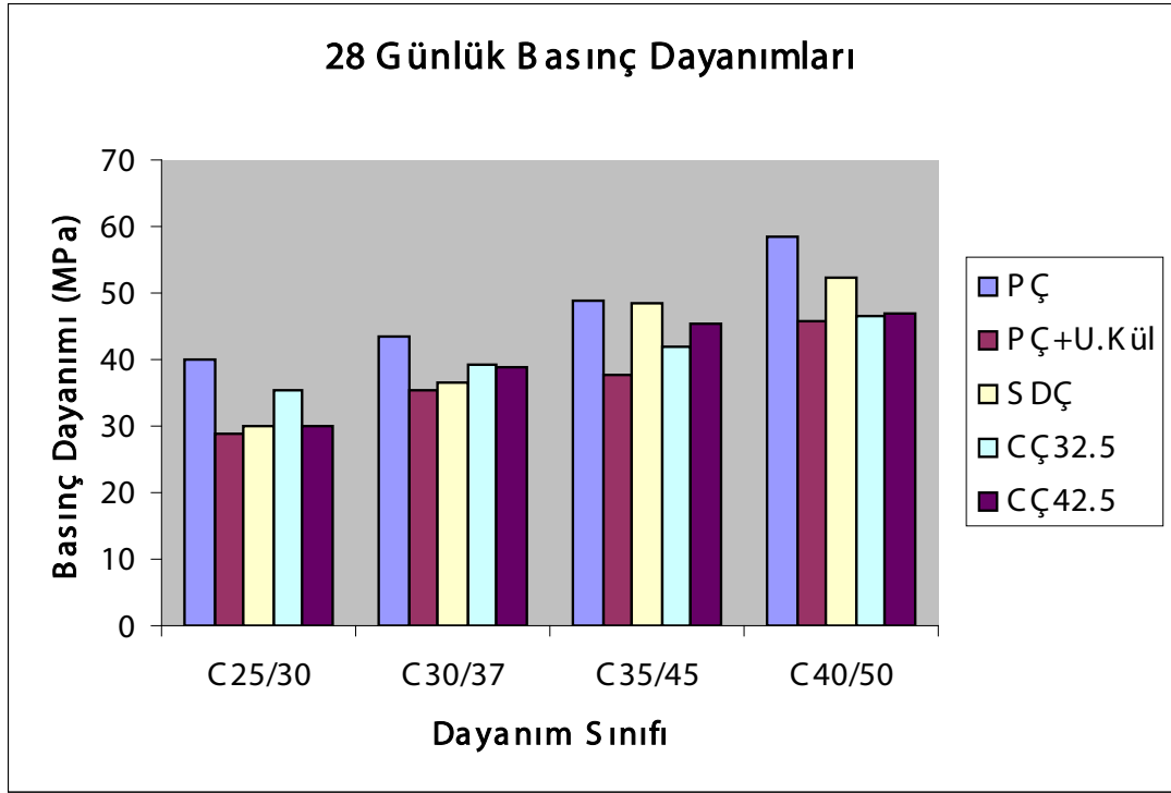
Şekil 4.1: 28 Günlük Basınç Dayanımları
