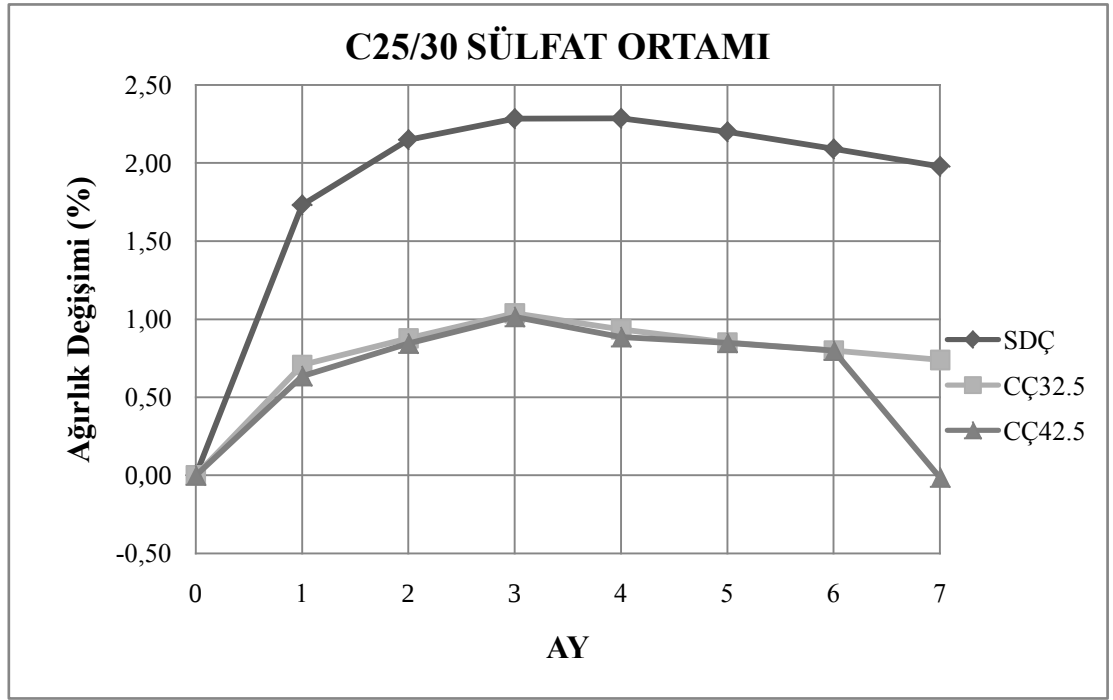
Şekil 4.8: C25 Dayanım Sınıfı Numunelerin Sülfat Ortamında Ağırlık Değişimi
