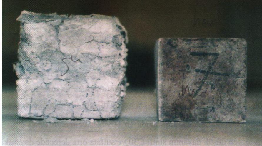
Şekil 2.12: Yüksek oranda alçıtaşı (kalsiyum sülfat) içeren harç örneklerinin havada ve su içinde bekletilmeleri halinde 84 gün sonundaki durumları. Soldaki ağır hasarlı örnek su içinde, sağdaki örnek ise havada bekletilmiştir
