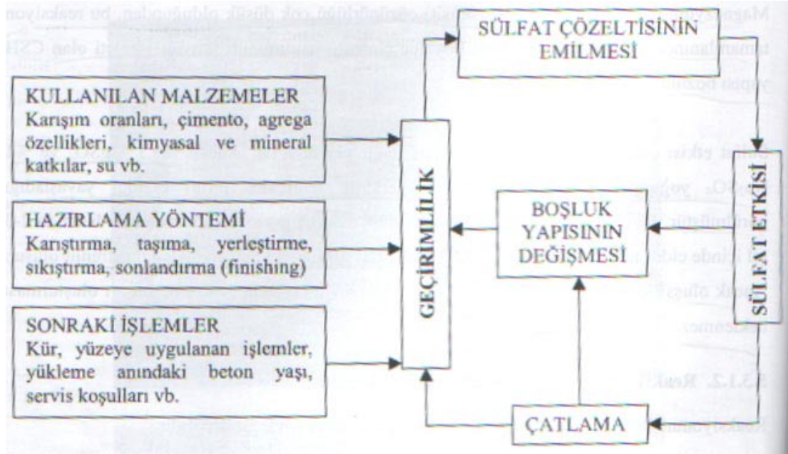
Şekil 2.10: Betonun sülfat dayanıklılığı ile geçirimsizliği arasındaki ilişki
