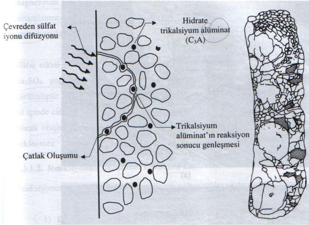
Şekil 2.8: Sülfat etkisiyle betonun bozulması
