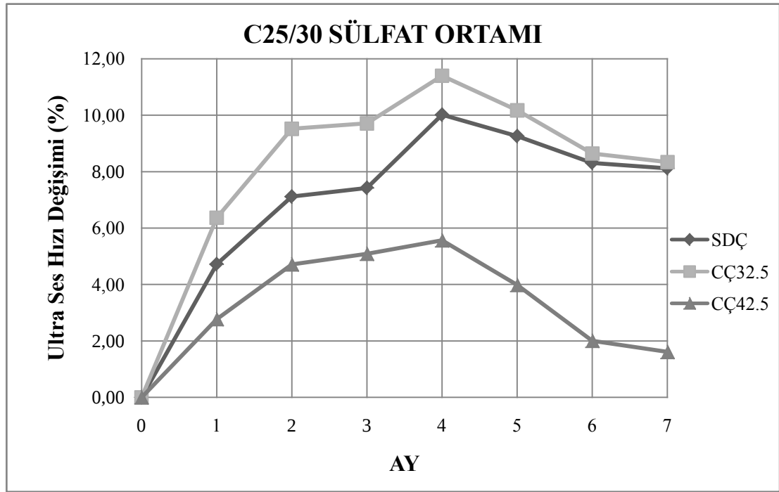
Şekil 4.10: C25 Dayanım Sınıfı Numunelerin Sülfat Ortamında Ultra Ses Hızı Değişimi
