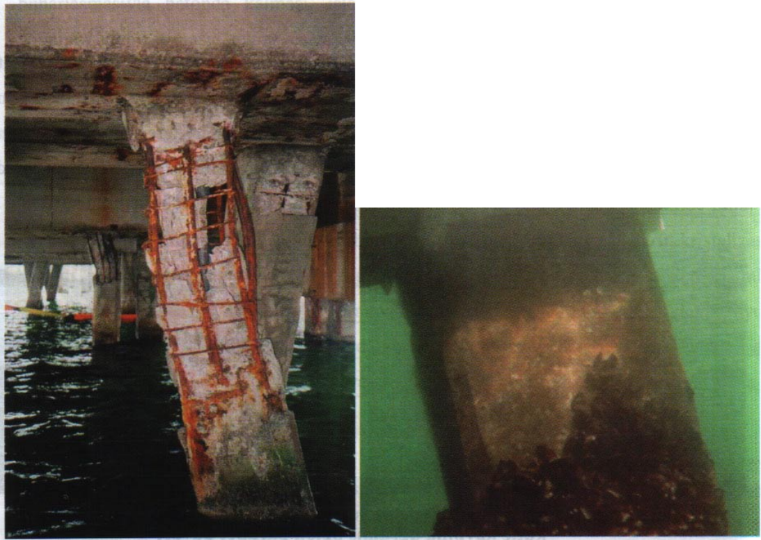
Şekil 2.16: Yarmca Pektim İskelesi'nde 1999 Marmara Depremi sonrası korozyon ve deprem hasarı (Solda) aynı yerde deniz altında kalan betonarme elemanlar (Sağda)
