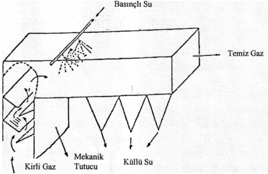
Şekil 2.4: Uçucu küllerin nemlendirme yöntemi ile tutulması
