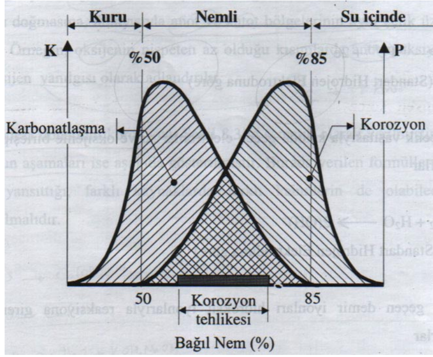
Şekil 2.20: Betonun karbonatlaşmasının ve betonarme donatısının korozyon hızının bağıl hava nemi ile değişimi
