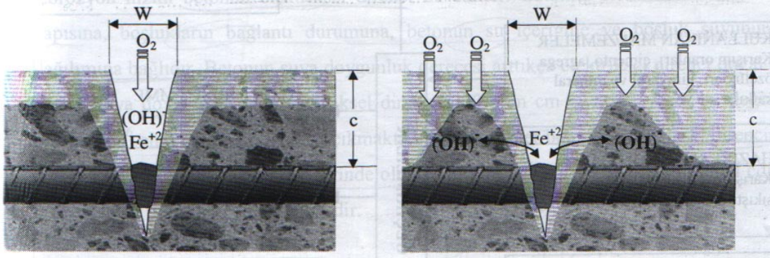
Şekil 2.27: Çatlak bölgesinde korozyonun gelişimi
