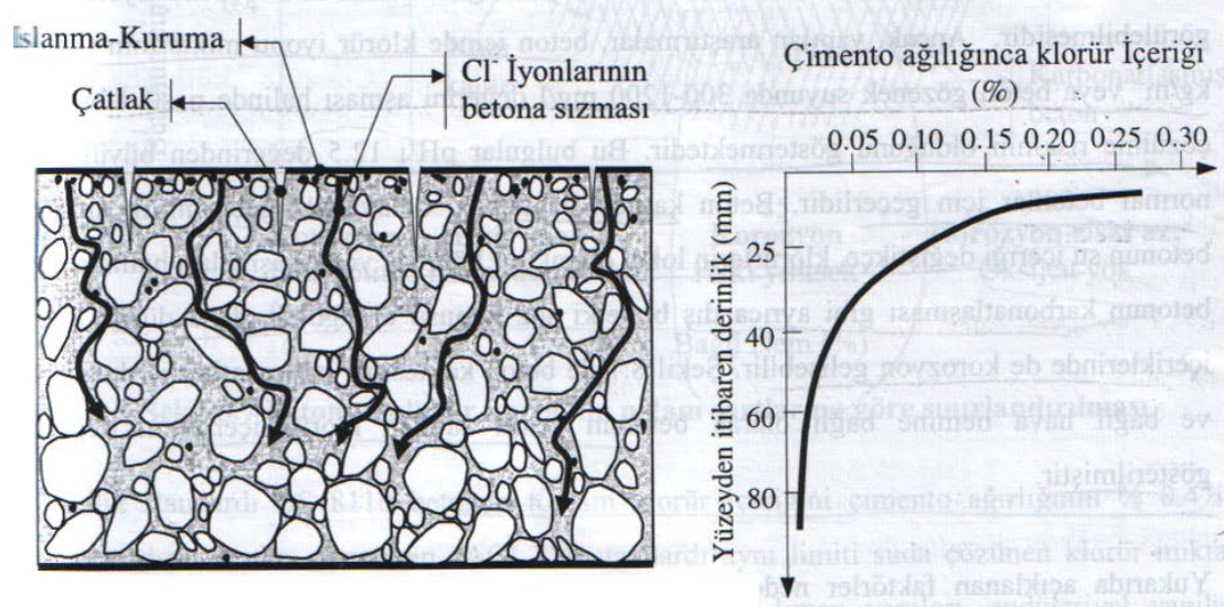
Şekil 2.23: Beton içine sonradan giren klorürlerin yüzeyden derine doğru miktarlarının değişimi
