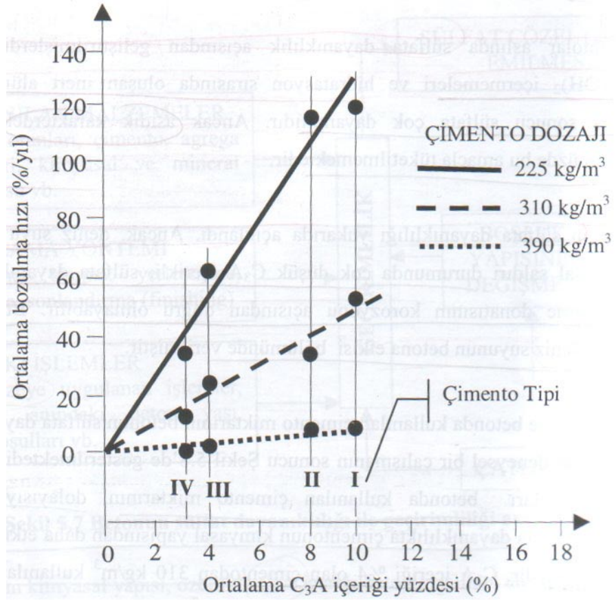
Şekil 2.11: Farklı tip çimentolarla değişik çimento içeriklerinde üretilmiş betonların sülfat etkisiyle bozulma hızları
