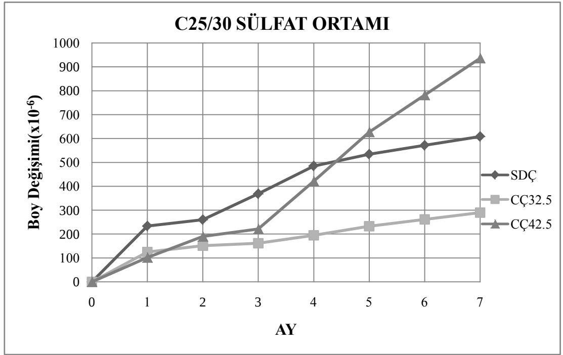
Şekil 4.9: C25 Dayanım Sınıfı Numunelerin Sülfat Ortamında Boy Değişimi
