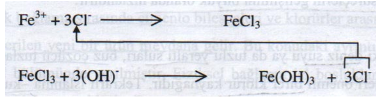
Şekil 2.21: Klorür bulunan ortamda korozyonun gelişimi
