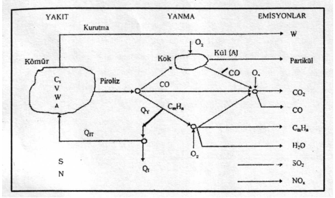
Şekil 2.3: Bir Kömür Taneciğinin yanması ve yanma ürünleri
