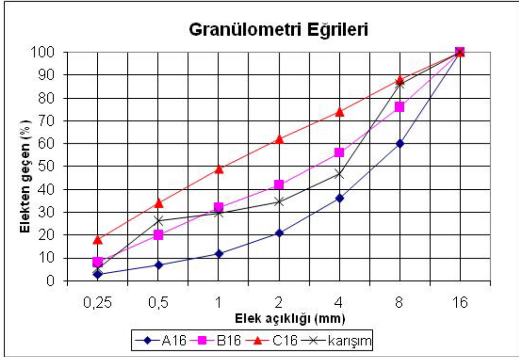
Şekil 3.1: Beton agregası karışımının granülometri
