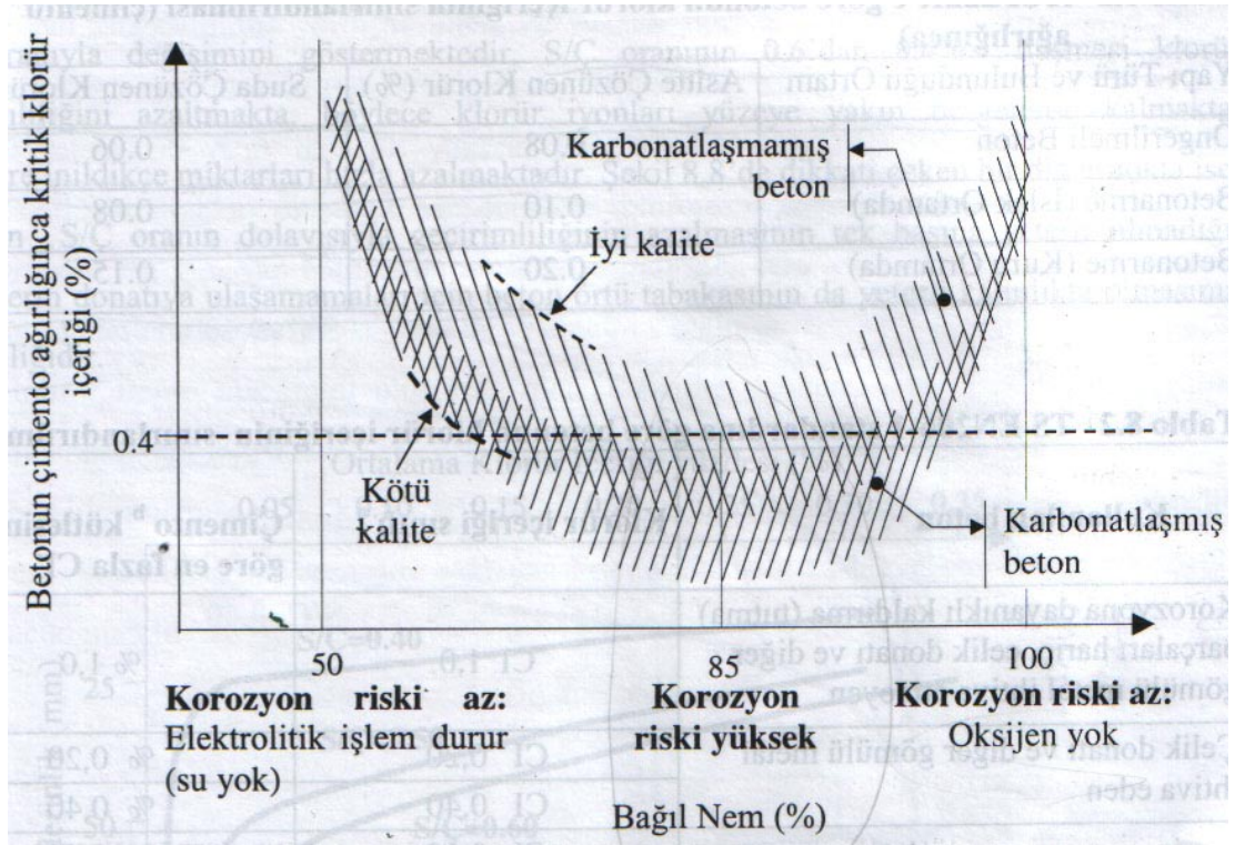
Şekil 2.24: Betonun klorür içeriğinin ortam şartlarına göre sınıflandırılması
