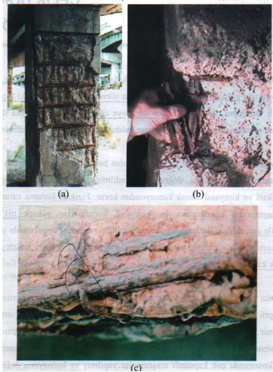
Şekil 2.17: Değişik korozyon hasarları a) Korozyon ürünlerinin genleşme etkisi ile pas payı tabakasını azaltması b) Donatının korozyon nedeniyle parçalanması c) Korozyon nedeniyle etriyelerin kopması
