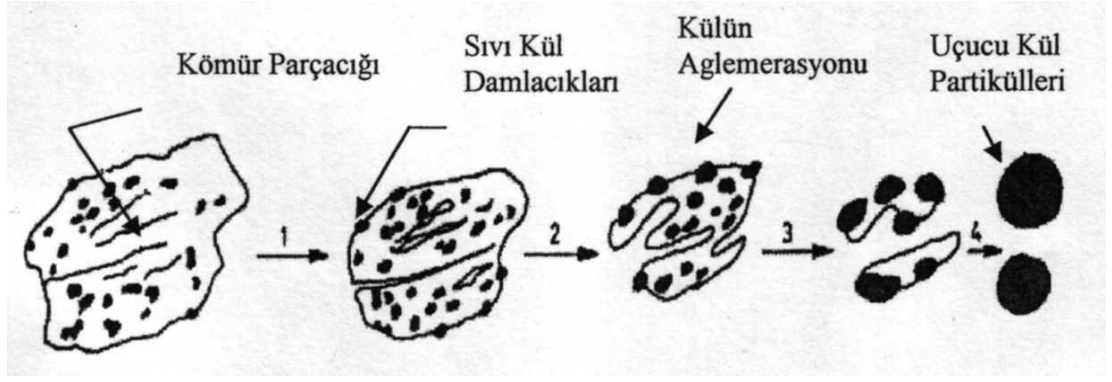
Şekil 2.2: Uçucu Külün Oluşum Safhaları
