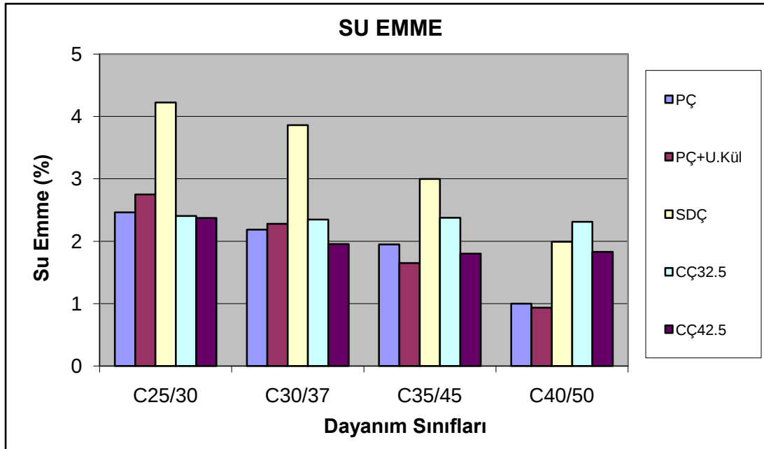
Şekil 4.5: Ağırlıkça Su Emme
