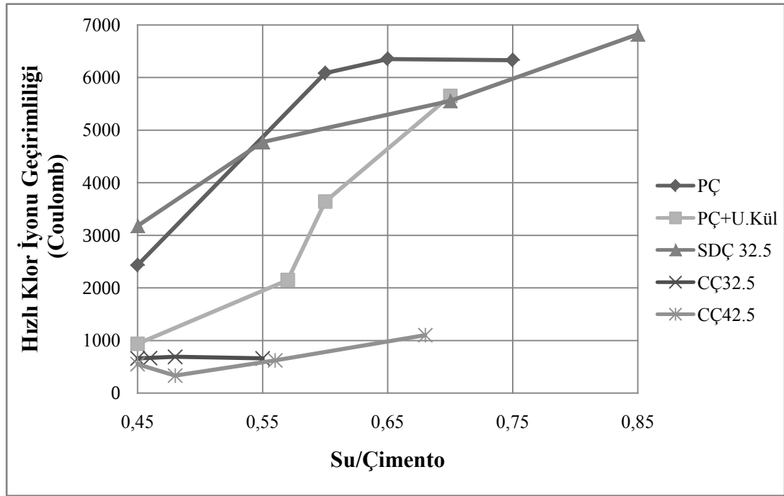
Şekil 4.7: Klor iyonu geçirirliiğinin S/Ç oranına göre değişimi
