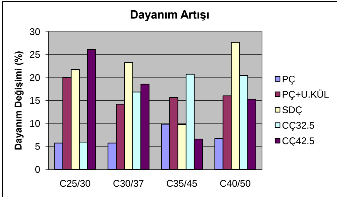
Şekil 4.3: Havada kür süresince dayanım artışı (%)
