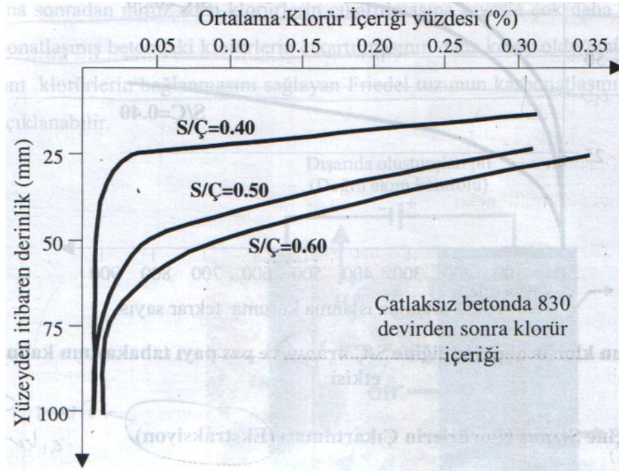
Şekil 2.25: Betonun klorür geçirimliliğine S/Ç oranının etkisi
