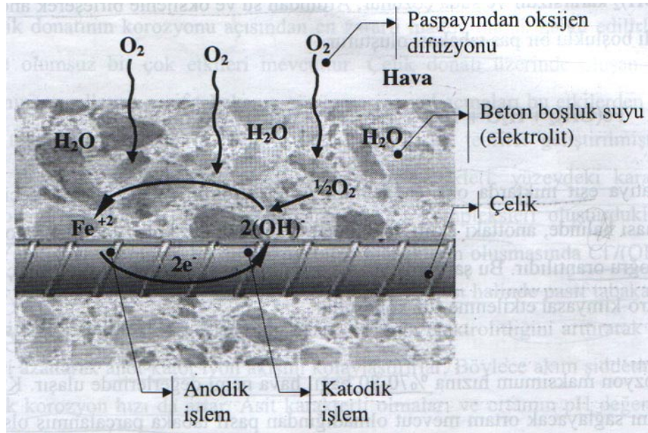
Şekil 2.19: Beton içinde gömülü çeliğin elektro-kimyasal korozyonu
