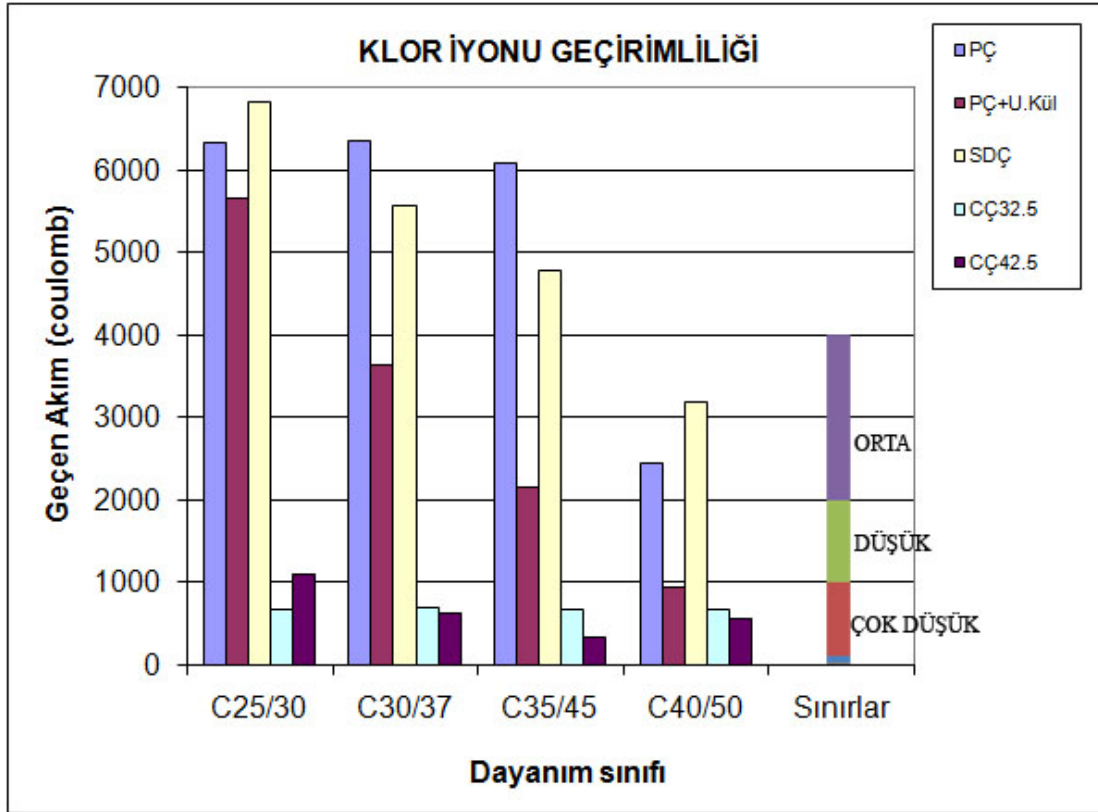
Şekil 4.6: Farklı çimento türlerinin klor iyonu geçirimsizliğine etkisi
