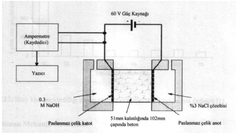
Şekil 3.2: Hızlı klor geçirimliliği deney düzeneği
