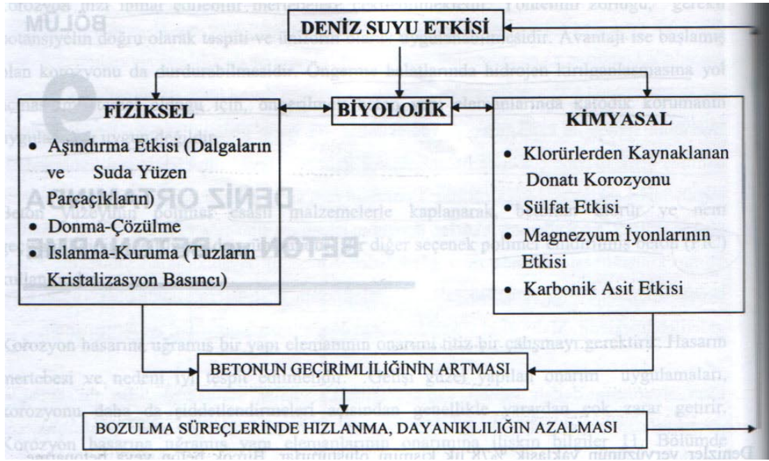
Şekil 2.14: Deniz ortamında bulunan yapıların maruz kalabilecekleri yıpratıcı etkiler
