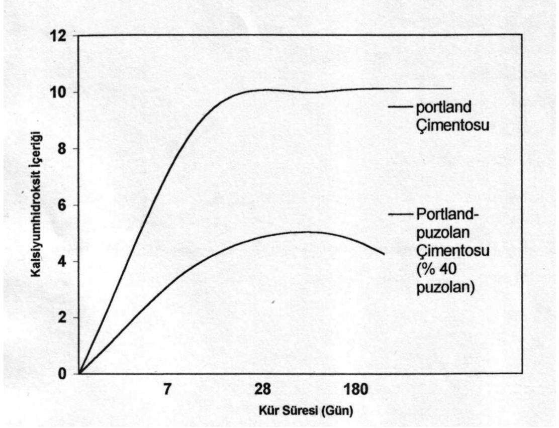
Şekil 2.1: Bir hidrate portlant-puzolan çimentosundaki kalsiyum hidroksit içeriğinin değişimi
