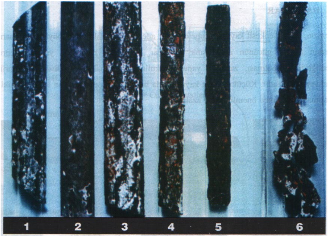
Şekil 2.29: Donatının korozyonu sonucu kesit kaybı ve parçalanması
