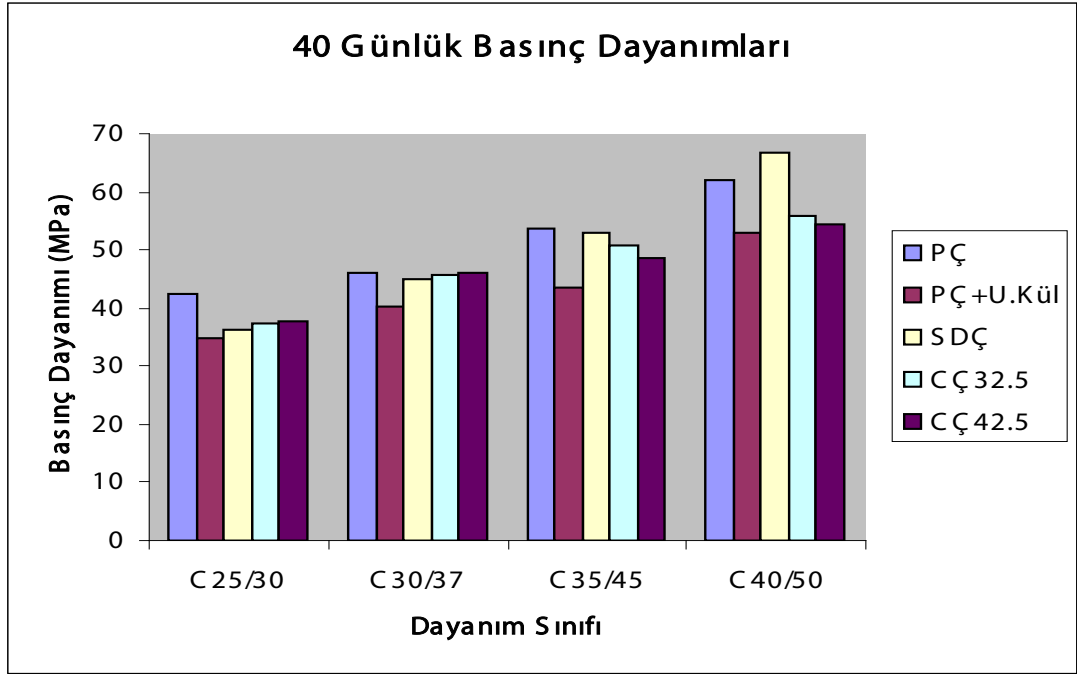
Şekil 4.2: 40 günlük basınç dayanımları
