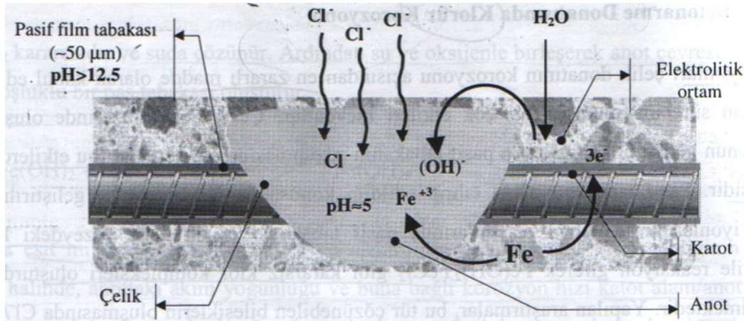
Şekil 2.22: Betonarme donatısında klorür iyonlarının yol açtığı oyulma tarzı korozyon
