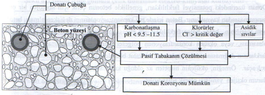
Şekil 2.18: Karbonatlaşma veya klorür iyonları nedeniyle betonun donatıyı korozyondan koruma etkinliğinin kaybolması
