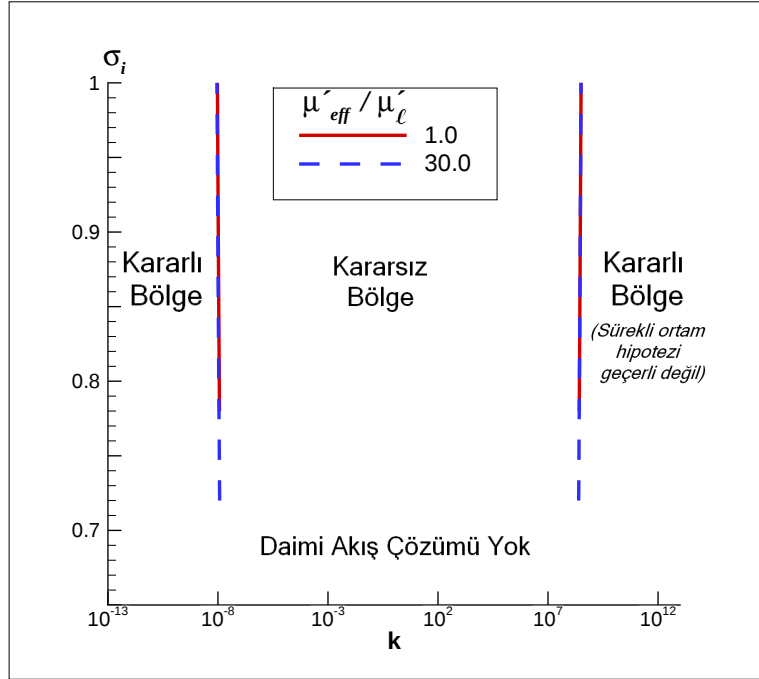
Şekil 3.3: Karışımın ideal akış durumunda sönüm katsayısının ( \mu'_{eff}/\mu'_\ell ) farklı değerleri için (1.0 ve 30.0) lüle girişindeki kavitasyon sayısının ( \sigma_i ) pertürbasyon dalga sayısı ( k ) değişimi ve kararlılık bölgeleri.
