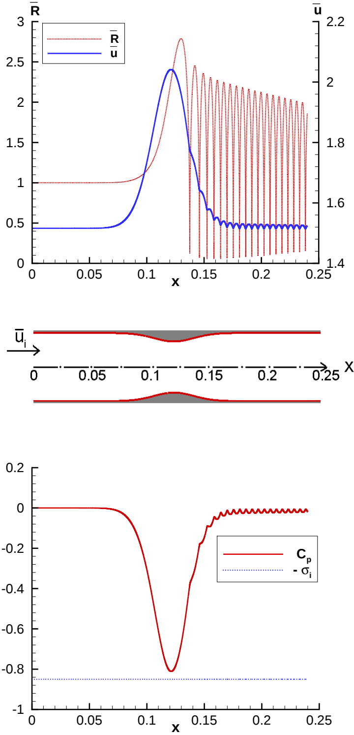
Şekil 3.1: Hava kabarcıkları içeren suyun daimi akışında kavitasyonsuz kabarcık yarıçapı ve akış hızının (üst şekil) ve basınç katsayısının (alt şekil), (3.28) denklemiyle kesit alanı verilen lülenin (orta şekil) eksen koordinatı boyunca değişimleri. Burada sönüm katsayısı \mu'_{eff}/\mu'_\ell = 1.0 , kabarcık/kabarcık etkileşim parametresi \Lambda = 1.0 , giriş kabarcık yarıçapı R'_i = 40\mu m , mikrodan makroya ölçek oranı L = 8 \times 10^{-4} , giriş basıncı p'_i = 1.013 bar, giriş hacimsel kabarcık oranı \beta_i = 10^{-3} ve kavitasyon sayısı \sigma_i = 0.85 olarak alınmıştır.
