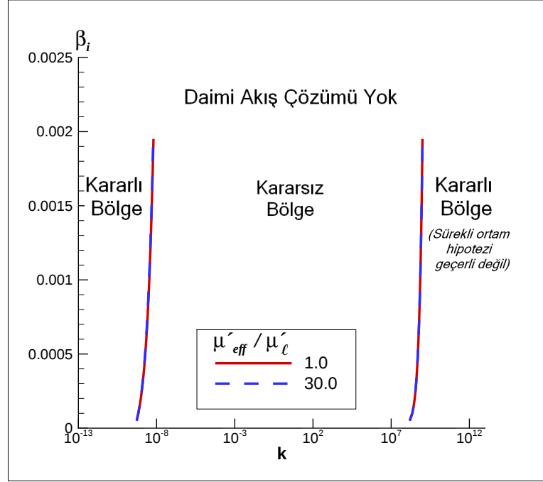
Şekil 3.4: Karışımın ideal akış durumunda sönüm katsayısının ( \mu'_{eff}/\mu'_\ell ) farklı değerleri için (1.0 ve 30.0) lüle girişindeki hacimsel kabarcık oranının ( \beta_i ) pertürbasyon dalga sayısı ( k ) değişimi ve kararlılık bölgeleri.
