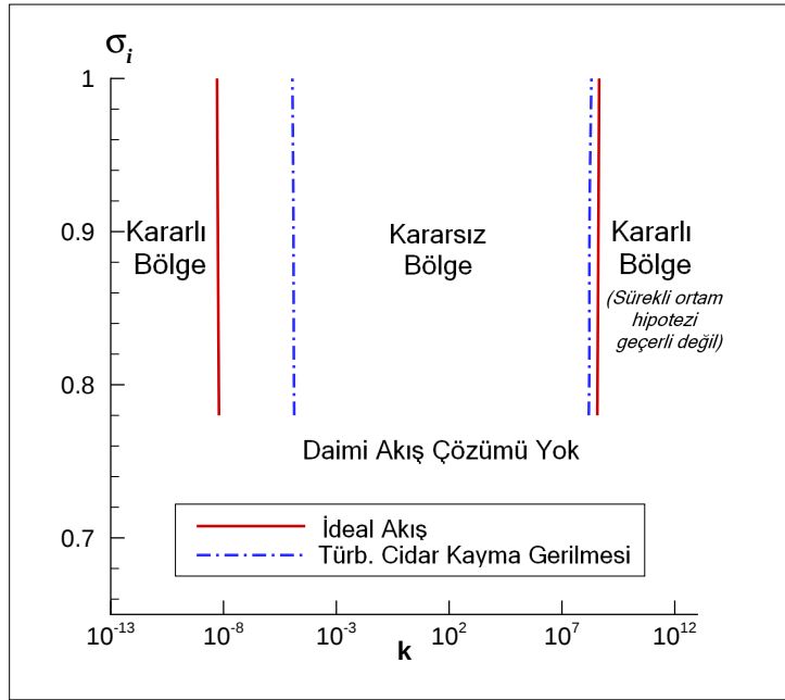
Şekil 3.7: Karışımın ideal akış ve türbülanslı cidar kayma gerilmesinin gözönüne alındığı hallerde lüle girişindeki kavitasyon sayısının ( \sigma_i ) pertürbasyon dalga sayısı ( k ) değişimi ve kararlılık bölgeleri.
