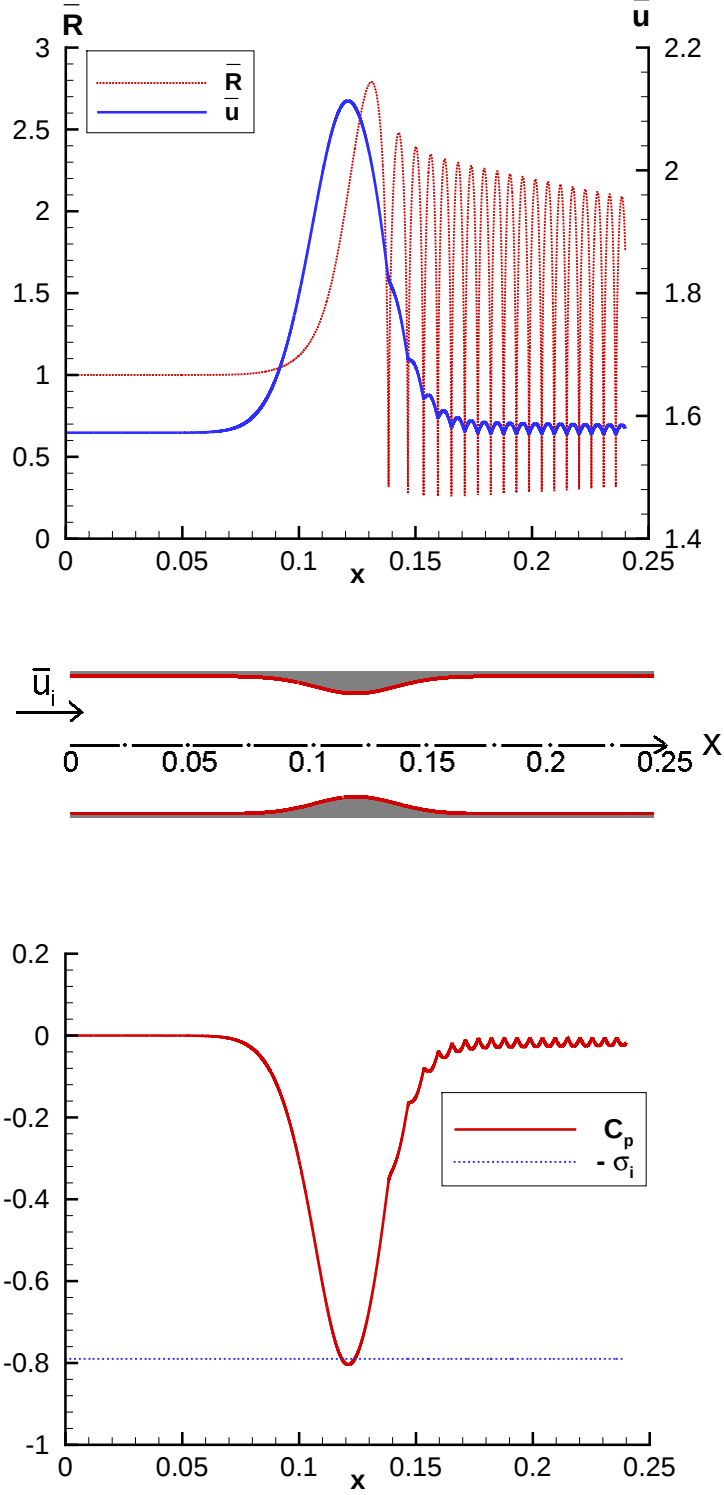
Şekil 3.2: Hava-su buharı kabarcıkları içeren suyun kaviteasyonlu daimi akışında kabarcık yarıçapı ve akış hızının (üst şekil) ve basınç katsayısının (alt şekil), (3.28) denklemiyle kesit alanı verilen lülenin (orta şekil) eksen koordinatı boyunca değişimleri. Burada sönüm katsayısı \mu'_{eff}/\mu'_\ell = 1.0 , kabarcık/kabarcık etkileşim parametresi \Lambda = 1.0 , giriş kabarcık yarıçapı R'_i = 40\mu m , mikrodan makroya ölçek oranı L = 8 \times 10^{-4} , giriş basıncı p'_i = 1.013 bar, giriş hacimsel kabarcık oranı \beta_i = 10^{-3} ve kaviteasyon sayısı \sigma_i = 0.79 olarak alınmıştır.
