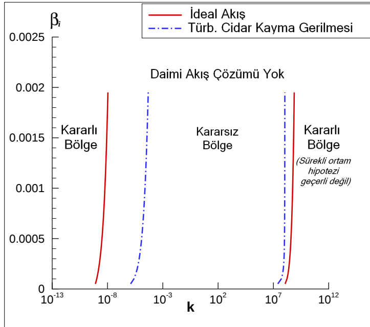
Şekil 3.8: Karışımın ideal akış ve türbülanslı cidar kayma gerilmesinin gözönüne alındığı hallerde lüle girişindeki hacimsel kabarcık oranının ( \beta_i ) pertürbasyon dalga sayısı ( k ) değişimi ve kararlılık bölgeleri.
