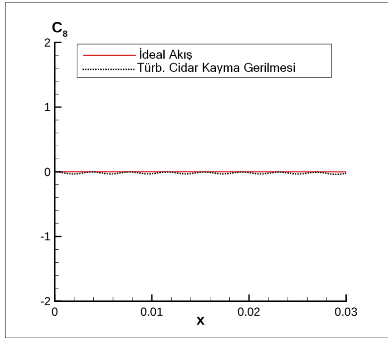
Şekil E.17: Kavitasyon katsayısı \sigma_i = 0.79 ve Şekil 3.2’deki koşullar altında (3.9)-(3.10) denklem sistemindeki C_8 katsayısının lüle giriş bölgesindeki değişimi.
