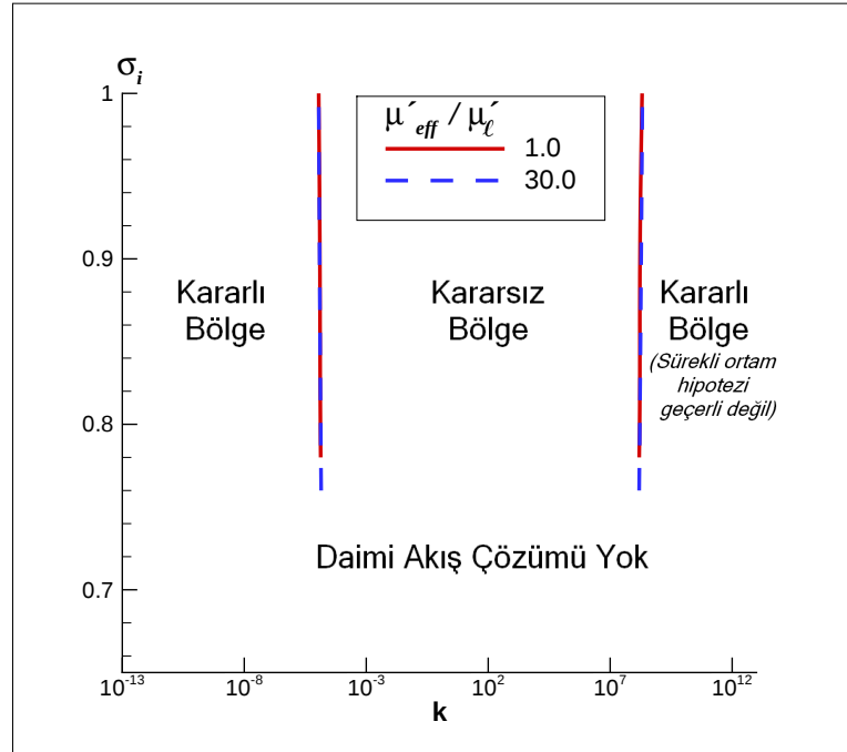
Şekil 3.5: Karışımın türbülanslı cidar kayma gerilmesinin gözönüne alındığı durumda sönüm katsayısının ( \mu'_{eff}/\mu'_\ell ) farklı değerleri (1.0 ve 30.0) için lüle girişindeki kavitasyon sayısının ( \sigma_i ) pertürbasyon dalga sayısı ( k ) değişimi ve kararlılık bölgeleri.
