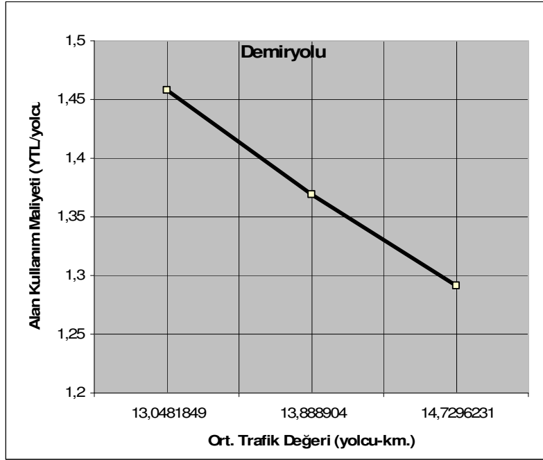
Şekil 3.2 – Demiryolu için Alan Kullanım Maliyeti / Trafik Değeri Yaklaşımları Grafiği
