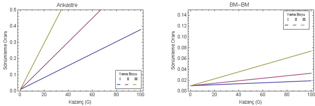
Şekil 3.17 : Farklı yama boyları için modal sönümleme oranı ile kazanç değişimi (birinci mod)
