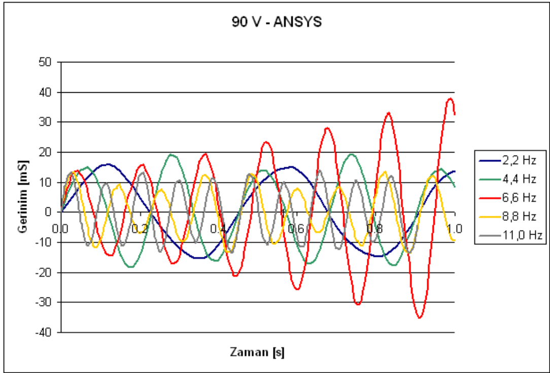
Şekil 4.12 : Farklı frekanslardaki sinüzoidal sinyaller için analiz sonucunda elde edilen gerinim değerleri (90 V).
