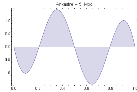
Şekil 3.13 : Ankastré ve iki ucundan basit mesnetlenmiş kiriş için mod şekilleri.
