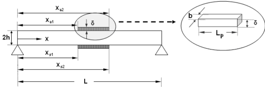
Şekil 3.12 : Çift piezoelektrik yamalı kiriş yapısı.
