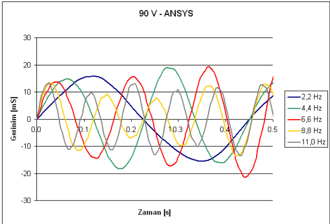
Şekil 4.13 : Farklı frekanslardaki sinüzoidal sinyaller için analiz sonucunda elde edilen gerinim değerleri (90 V – 0,5 s).
