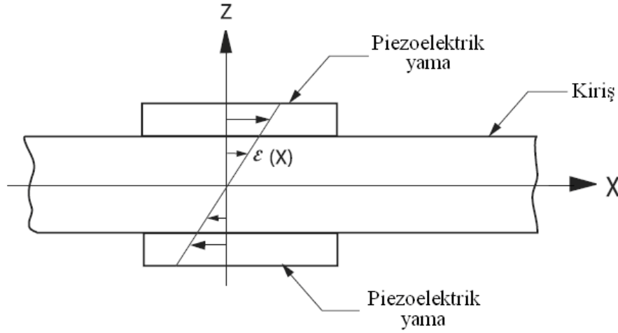
Şekil 3.8 : Simetrik yamalı kiriş yapıda gerinim dağılımı [44].
