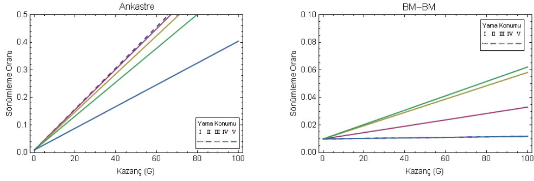
Şekil 3.16 : Farklı yama konumları için modal sönümleme oranı ile kazanç değişimi (birinci mod)
