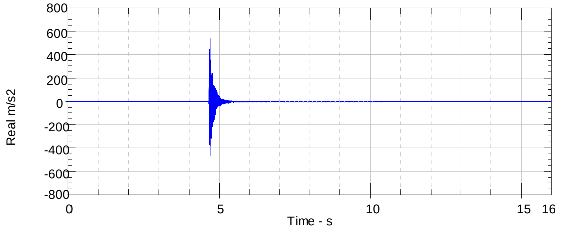
Şekil B.4 : Tek yamalı kiriş için çekiç testi ile elde edilen ivme-zaman grafiği.
