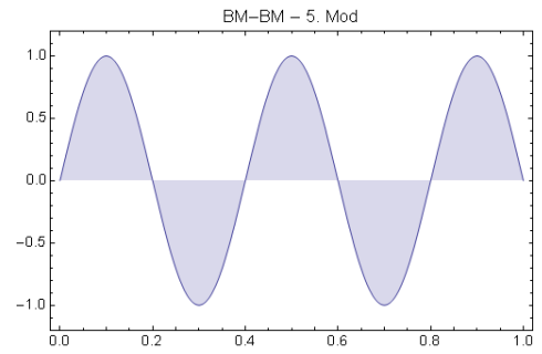
Şekil 3.13 : Ankastré ve iki ucundan basit mesnetlenmiş kiriş için mod şekilleri.
