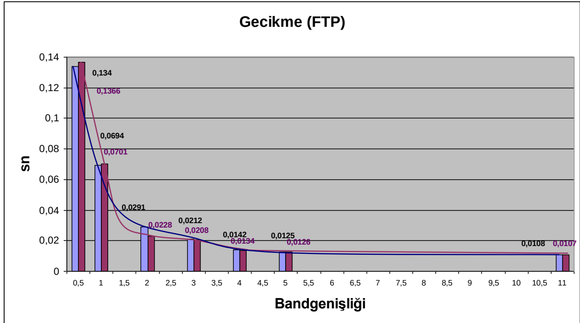
Şekil 8.8: FTP trafięindeki paket gecikmesi
