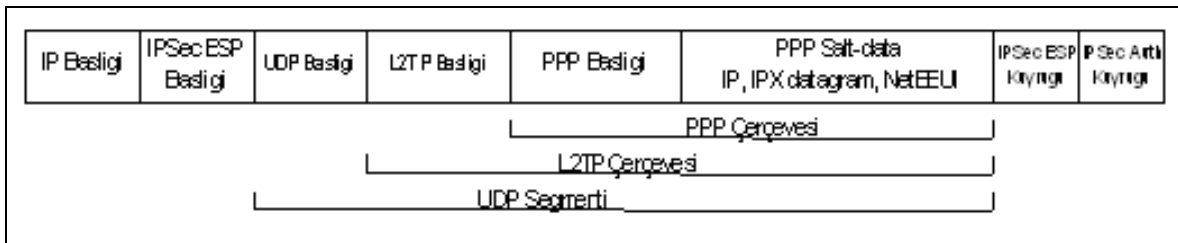
Şekil 5.4: L2TP/IPSec ESP Kapsülleme
