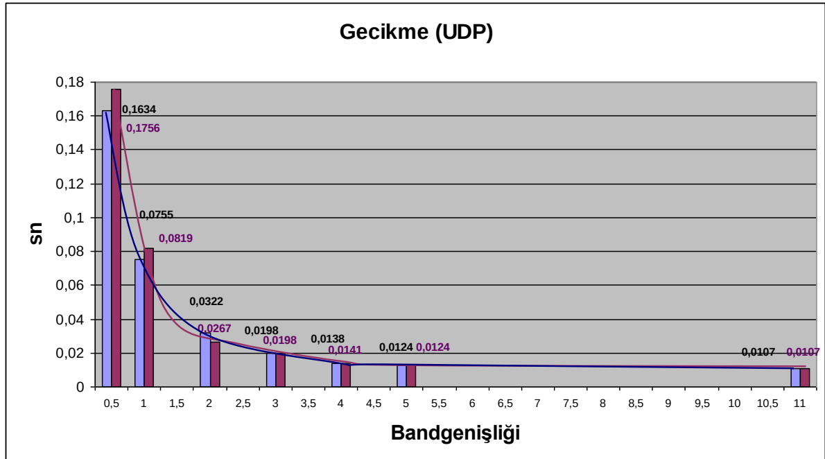
Şekil 8.9: UDP trafięindeki paket gecikmesi
