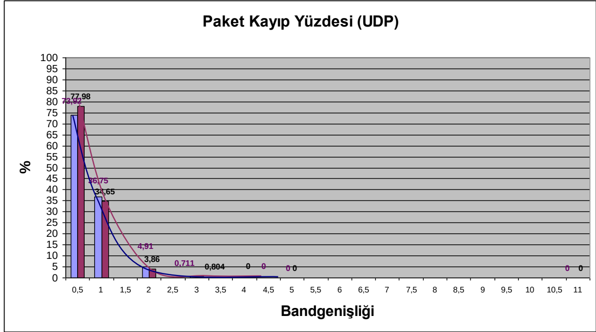
Şekil 8.5: UDP trafięindeki paket kaybı
