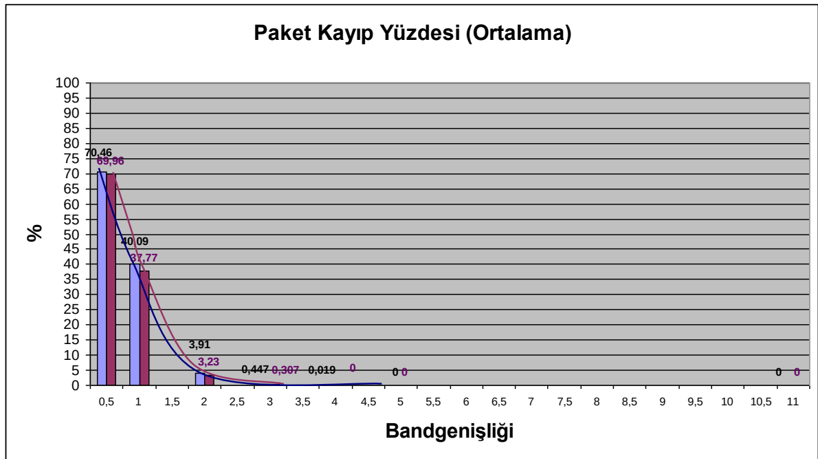
Şekil 8.2: Ortalama paket kaybı
