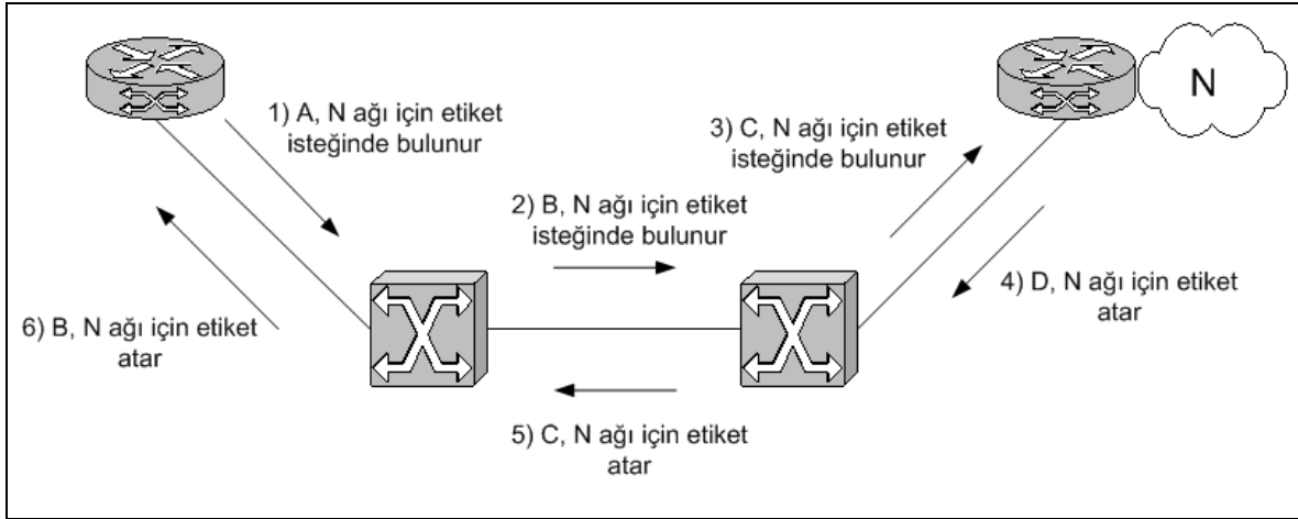
Şekil 4.7: Sıralı kontrol
