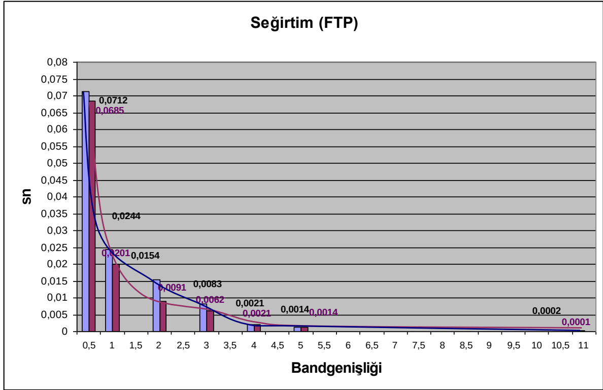
Şekil 8.11: FTP trafiğindeki seğirtim
