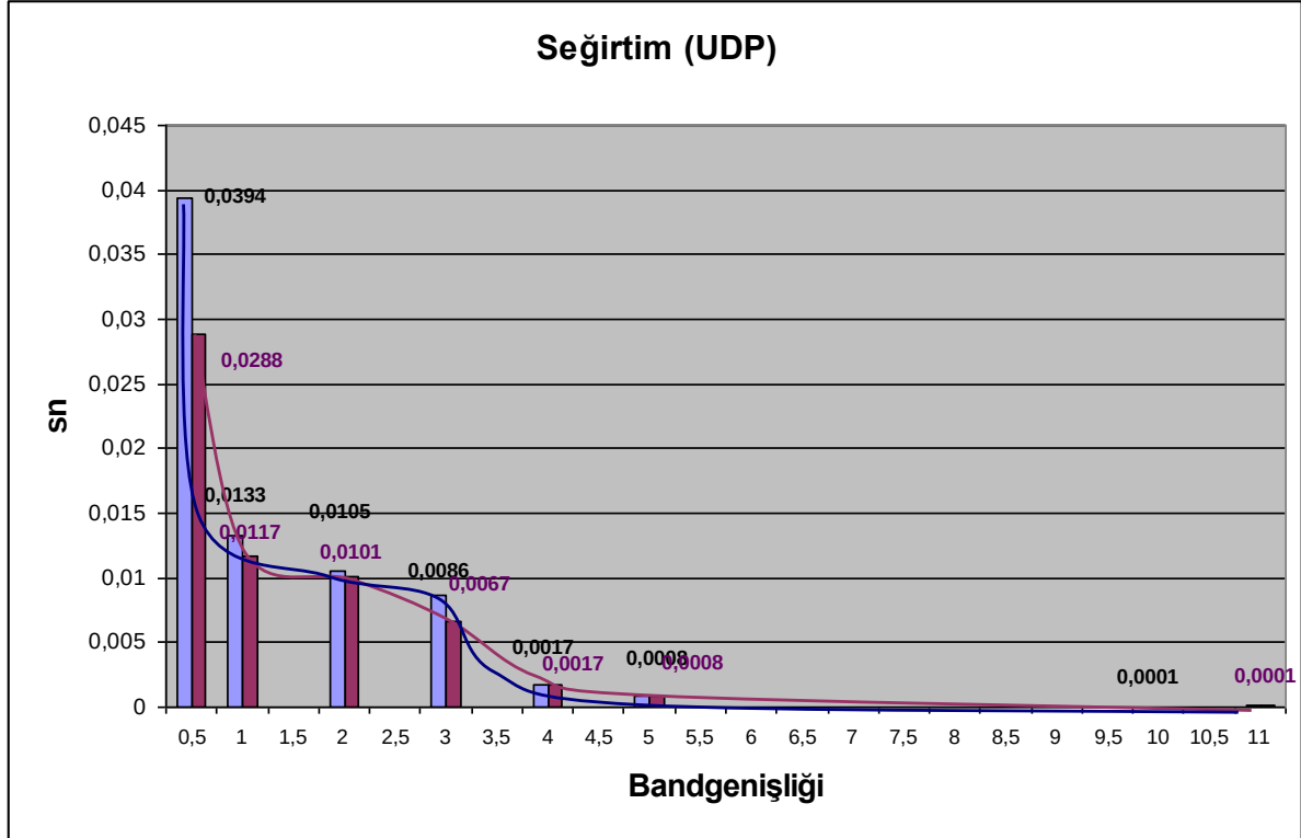
Şekil 8.12: UDP trafiğindeki seğirtim
