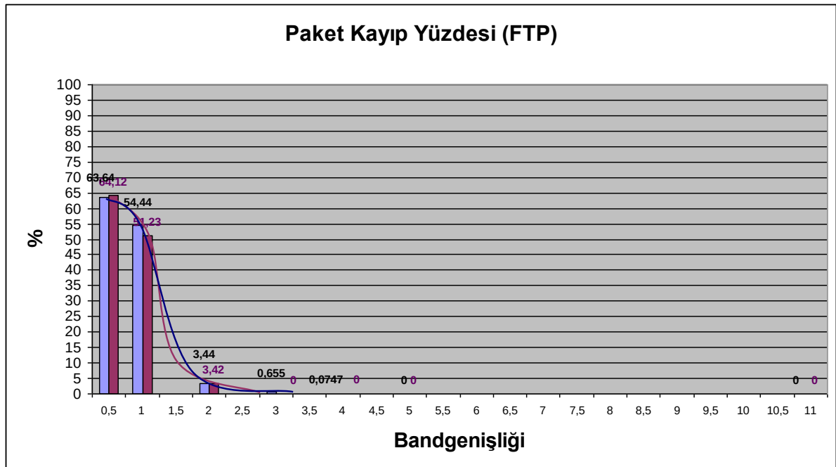
řekil 8.4: FTP trafiđindeki paket kaybı
