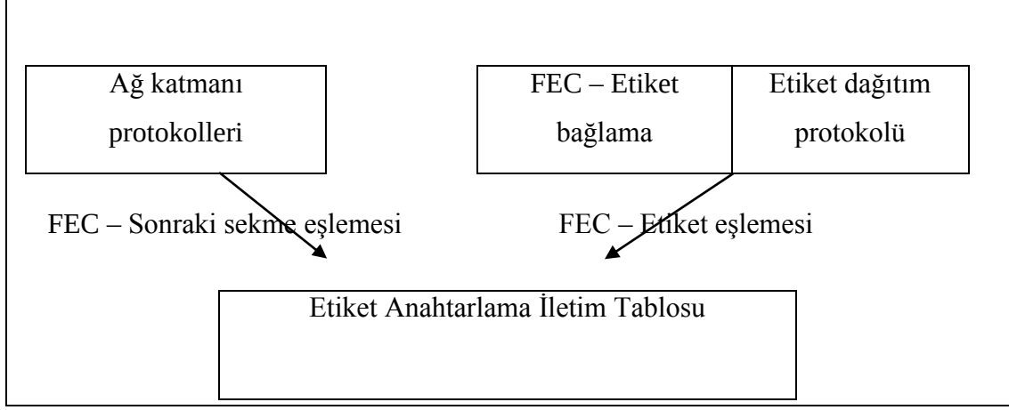
Şekil 3.5: Etiket Anahtarlama Denetim Düzlemi
