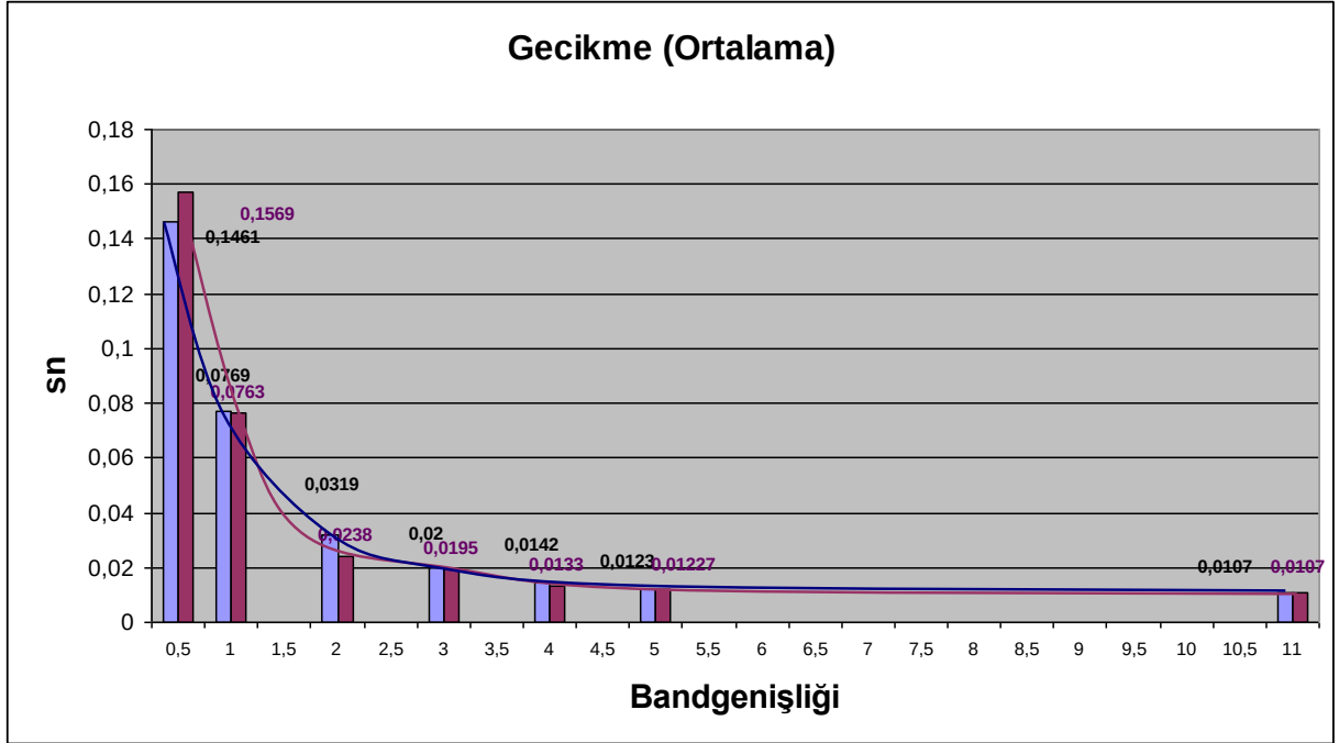
řekil 8.6: Ortalama paket gecikmesi
