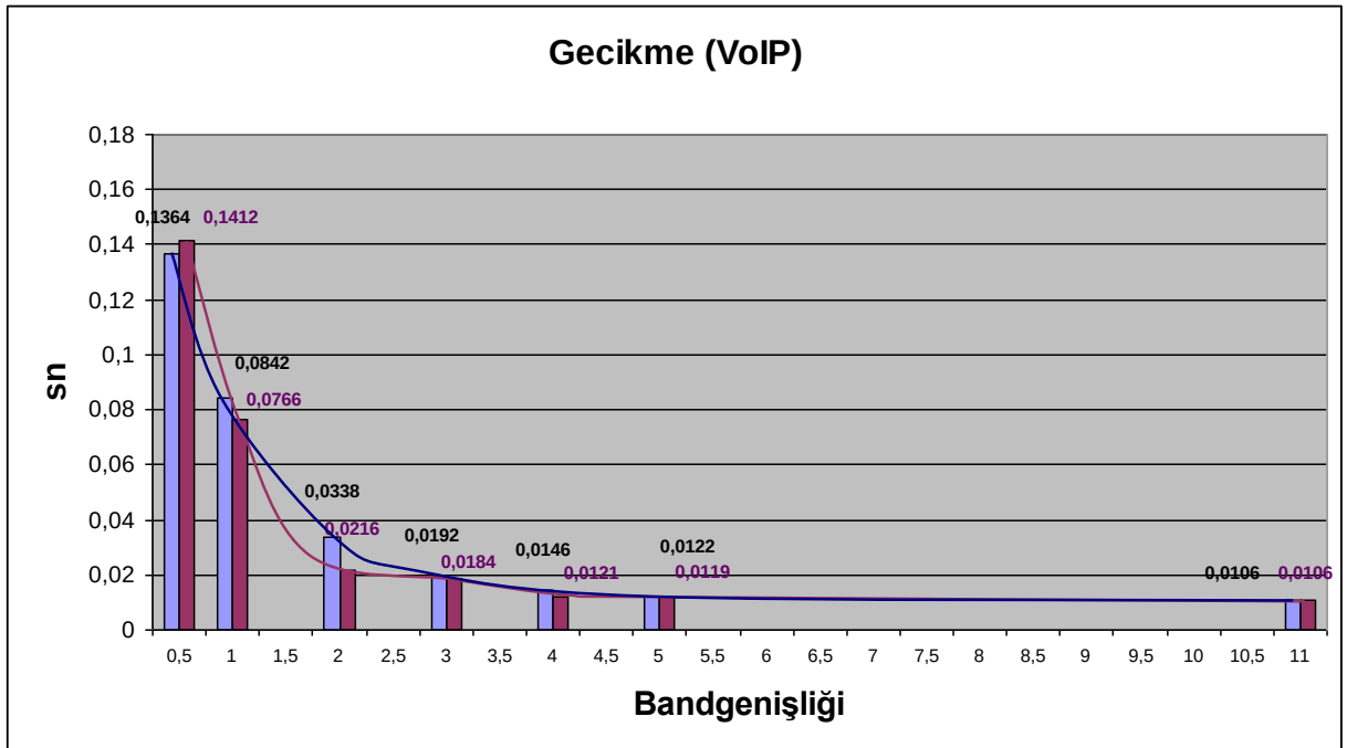
řekil 8.7: VoIP trafiđindeki paket gecikmesi
