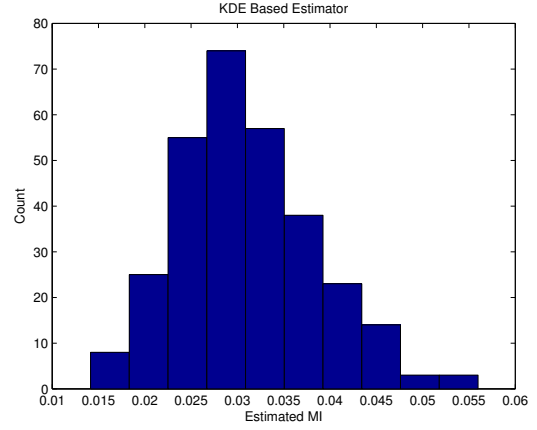
(d) KDE based estimator
