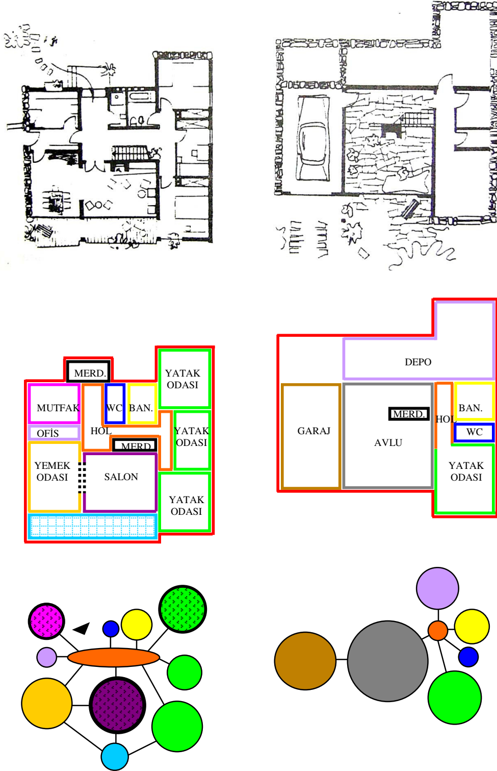
Şekil 5.15: 4. Levent K Tipi Konut Plan Örneği, 1954–1960 (Dülgeroğlu, 1995)
