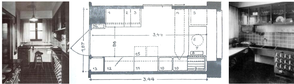
Şekil 4.3: Frankfurt Mutfağı'nın Plan ve Fotoğrafları ( www.arkitera.com.tr ; Eroğlu, 2000)
