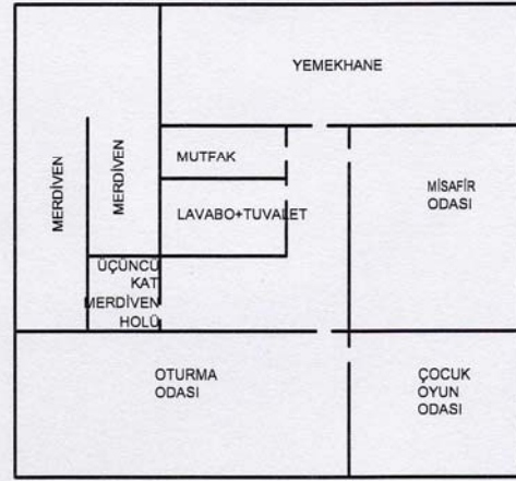
ÜÇÜNCÜ KAT
