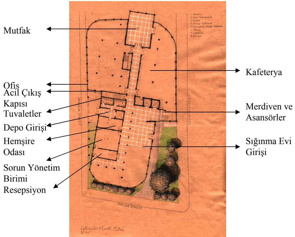
Şekil 5.35: Sığınma Evi Projesi Giriş Katı Planı (Kronawitter,2005)
