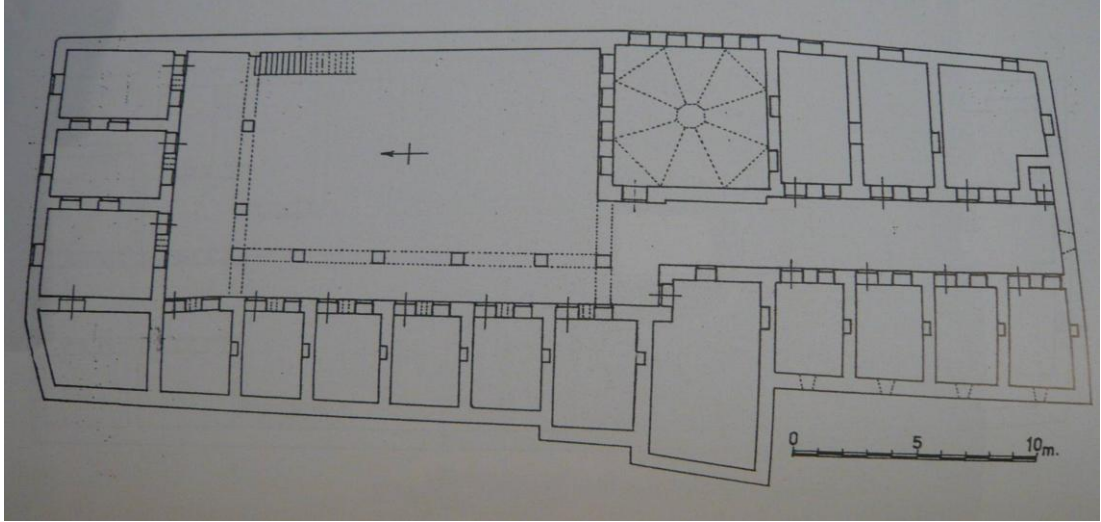
Şekil 5.45 : Gümrük Hanı üst kat planı (Çam, 2006).
