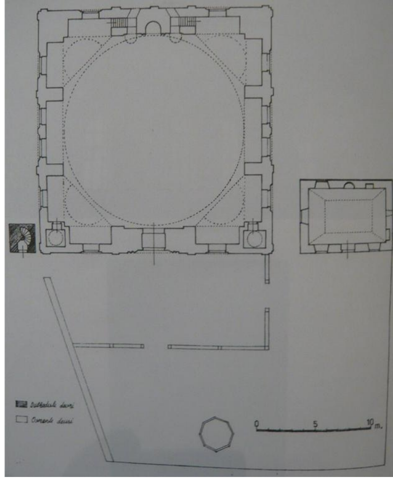
Şekil 5.63 : Alaüddevle Camisi planı (Çam, 2006).
