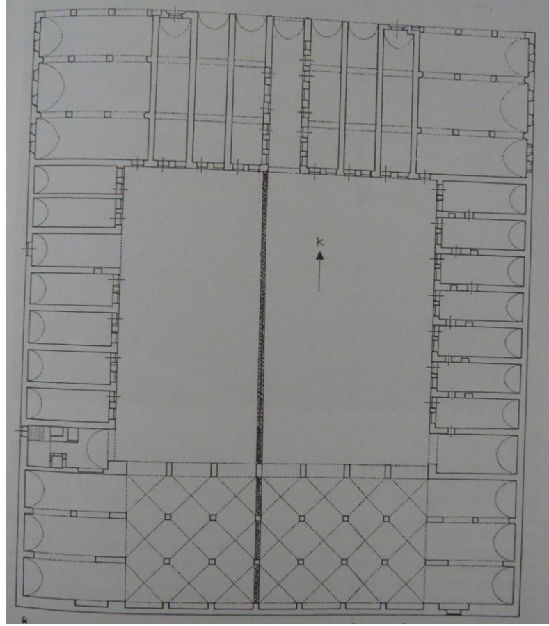
Şekil 5.40 : Bayaz Han zemin kat planı (Çam, 2006).
