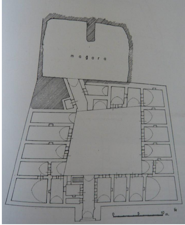
Şekil 5.61 : Yüzükü Han zemin kat planı (Çam, 2006).
