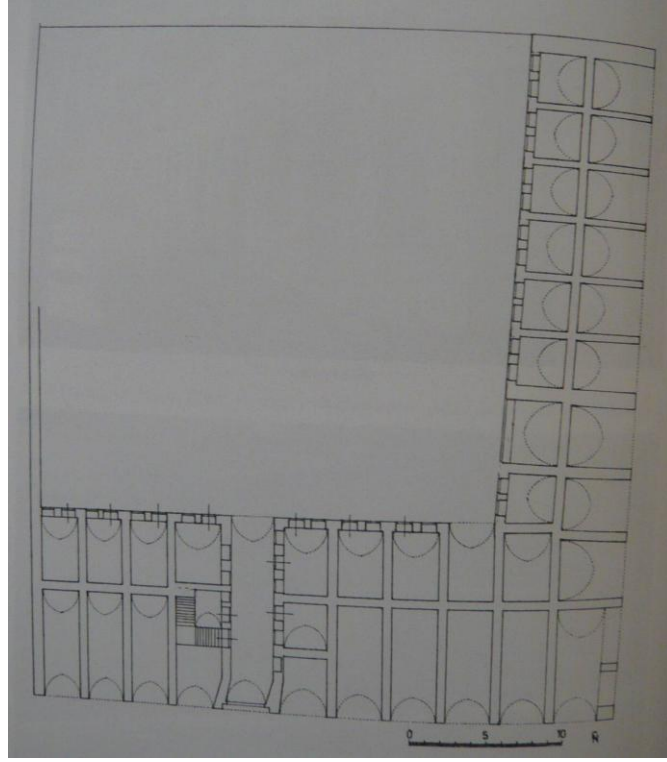
Şekil 5.47 : Güven Hanı zemin kat planı (Çam, 2006).
