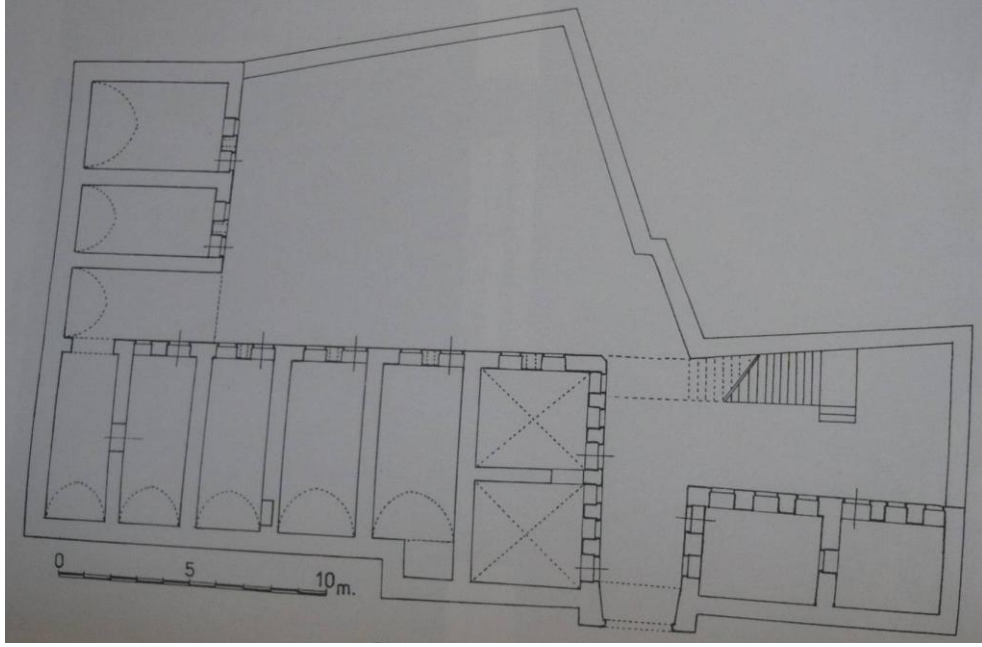
Şekil 5.57 : Şeker Hanı zemin kat planı (Çam, 2006).
