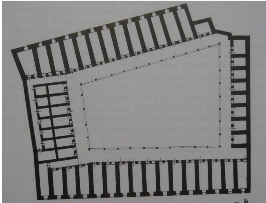
Şekil 5.36 : Mecidiye Hanı üst kat planı (Çam, 2006).
