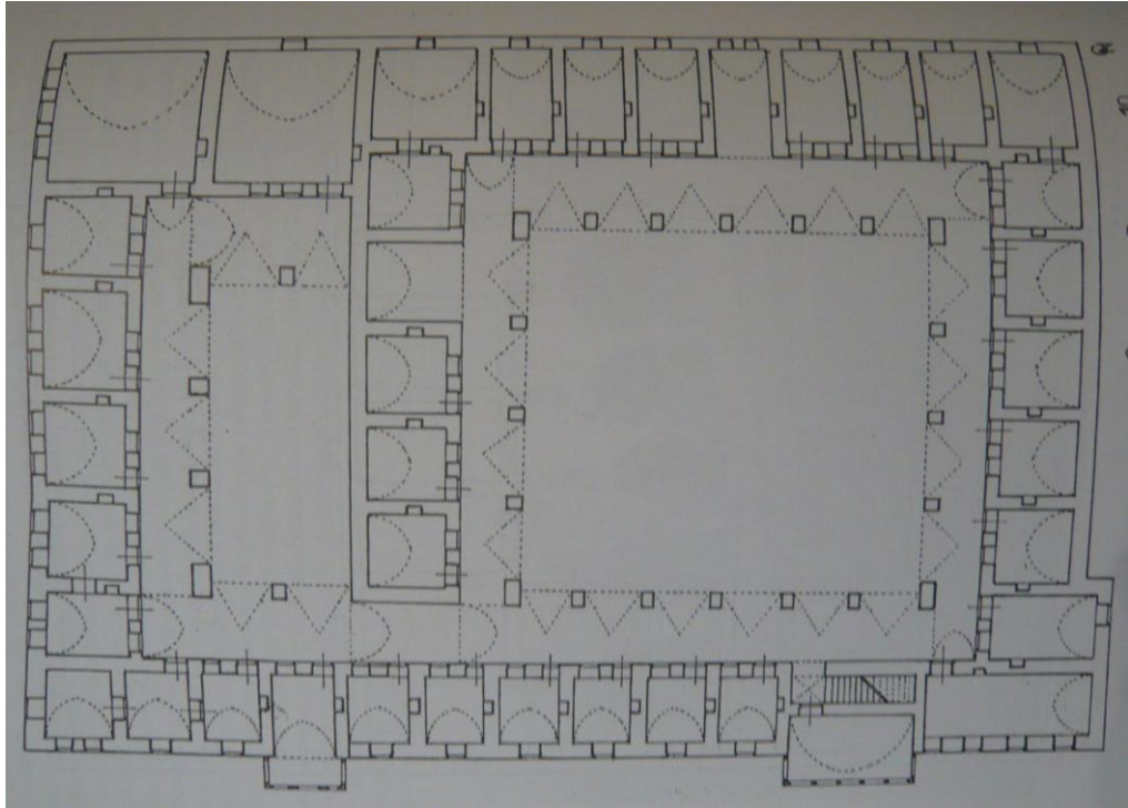
Şekil 5.43 : Elbeyli Hanı üst kat planı (Çam, 2006).
