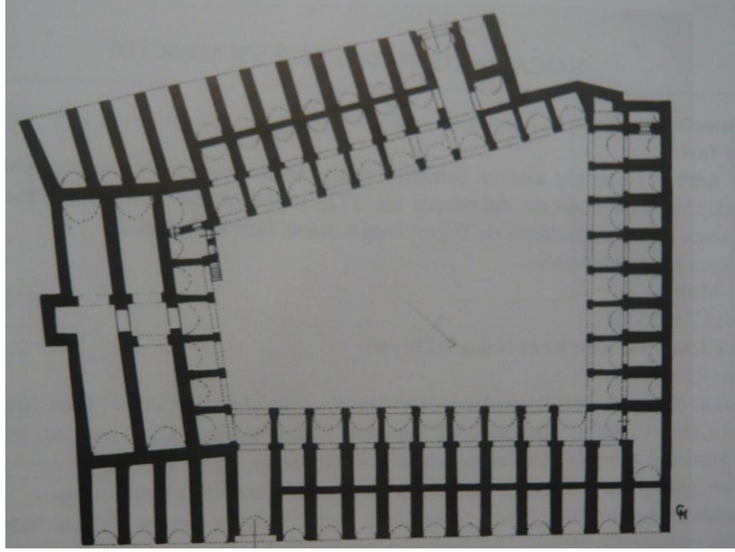
Şekil 5.35 : Mecidiye Hanı zemin kat planı (Çam, 2006).
