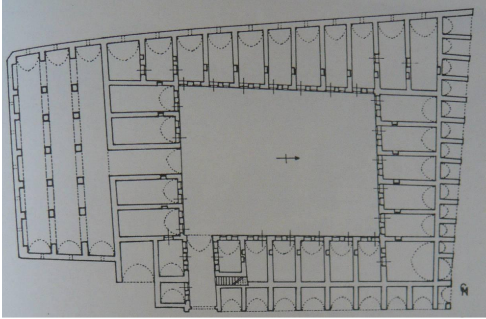
Şekil 5.54 : Millet Hanı zemin kat planı (Çam, 2006).
