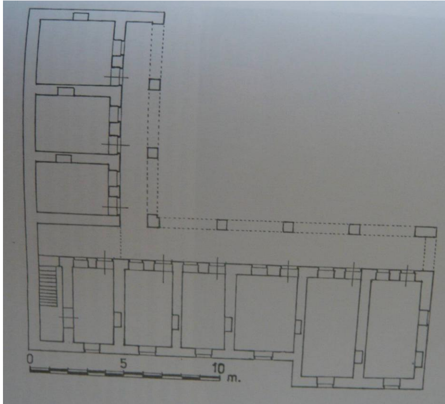
Şekil 5.58 : Şeker Hanı üst kat planı (Çam, 2006).
