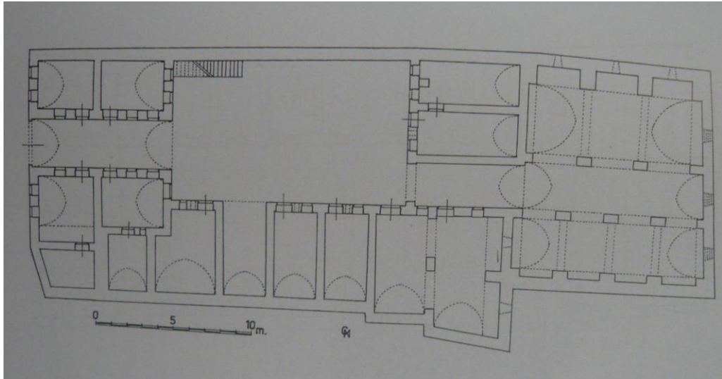
Şekil 5.44 : Gümrük Hanı alt kat planı (Çam, 2006).
