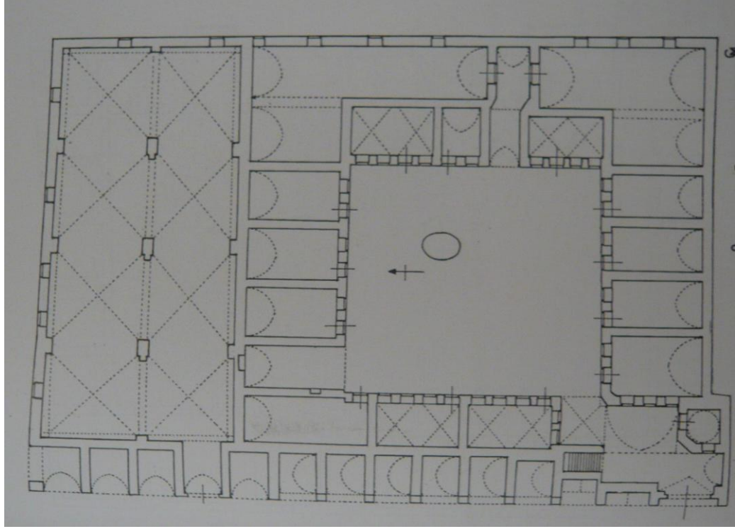
Şekil 5.42 : Elbeyli Hanı zemin kat planı (Çam, 2006).
