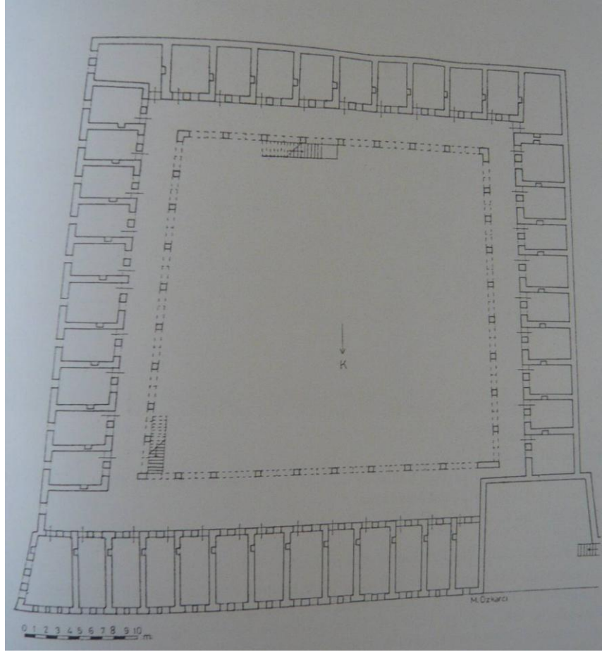
Şekil 5.60 : Tuz Hanı zemin kat planı (Çam, 2006).
