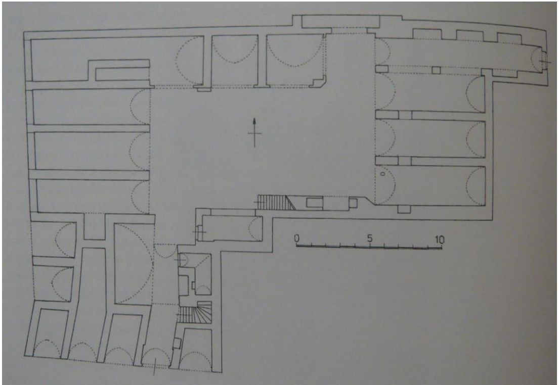
Şekil 5.49 : Kumruoğlu Hanı zemin kat planı (Çam, 2006).
