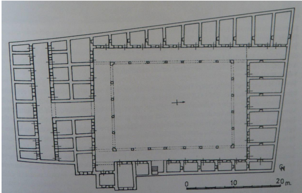
Şekil 5.55 : Millet Hanı üst kat planı (Çam, 2006).
