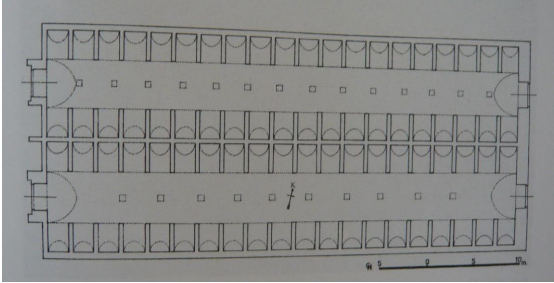
Şekil 5.62 : Kemikli Bedesten planı (Çam, 2006).
