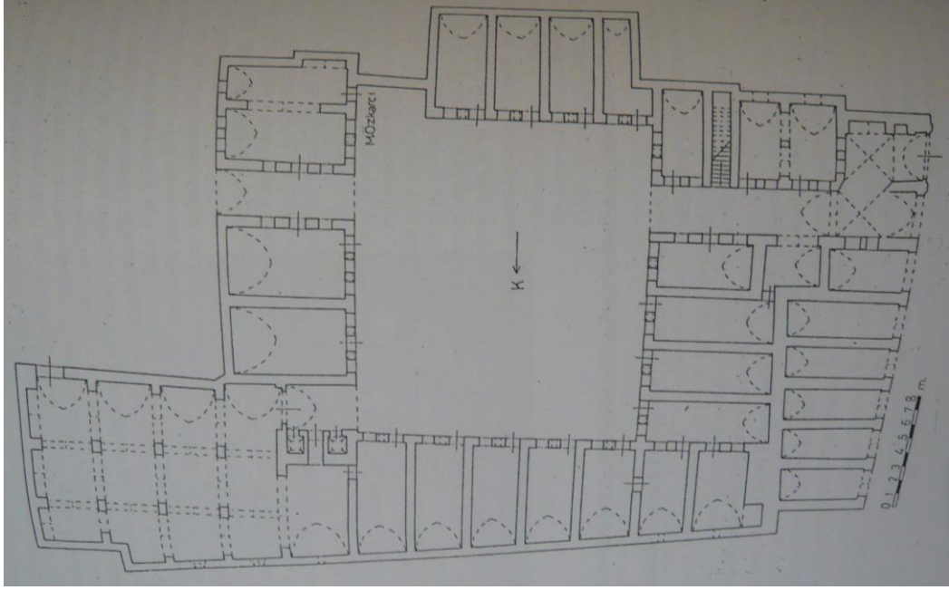
Şekil 5.51 : Kürkçü Hanı zemin kat planı (Çam, 2006).
