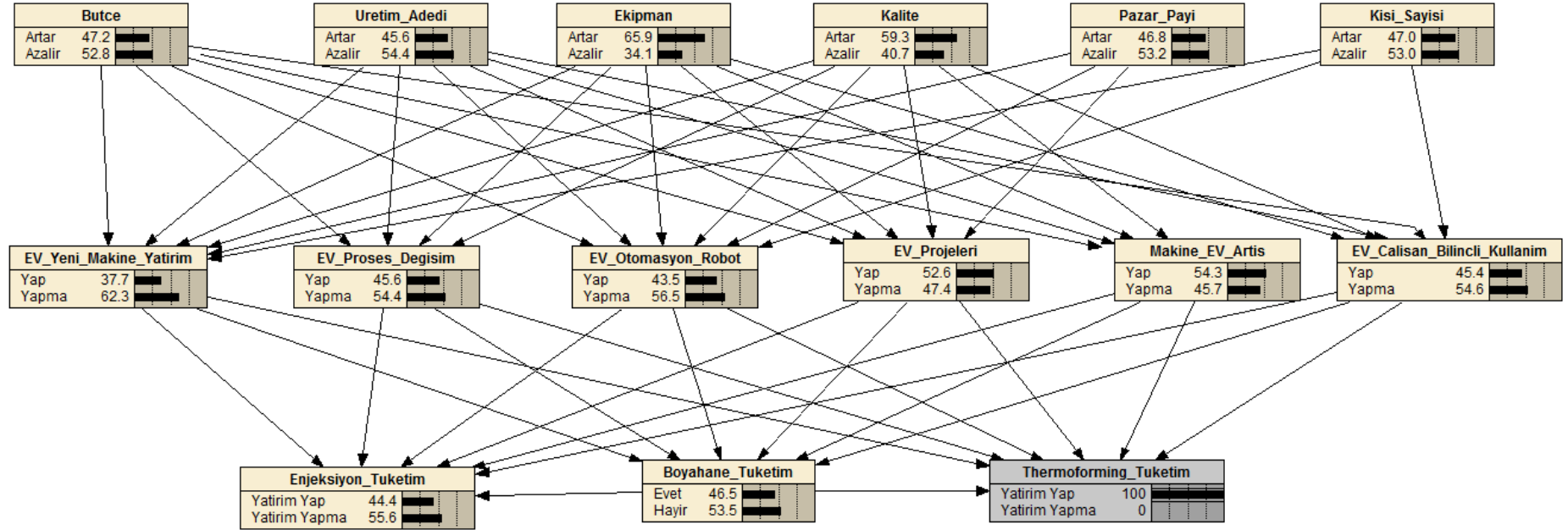
Şekil A.10 : Thermoform. enerji tüketimi yatırım yap durumu için NETICA modeli.
