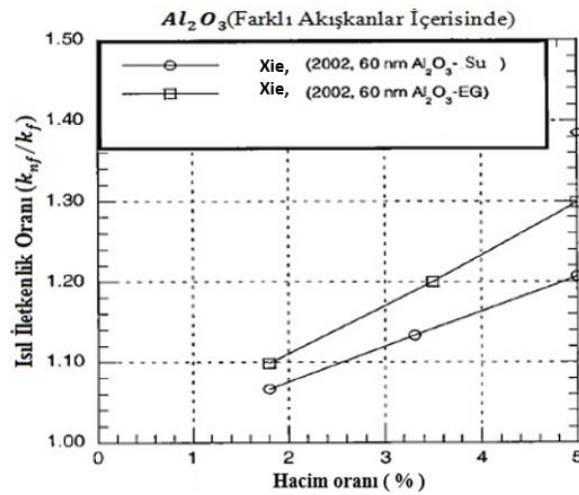
Şekil 3.7 : Ana akışkan malzemesinin etkisi (Yu ve diğ. 2007).
