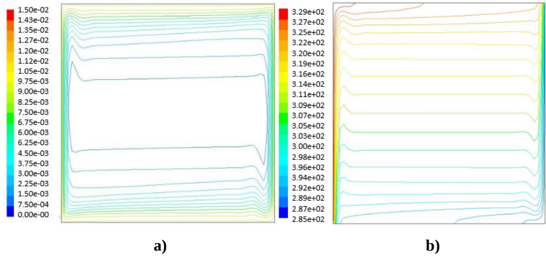
Şekil 4.8: Ra = 7,6 \times 10^7 için tez çalışması a) akım çizgileri b) eş sıcaklık eğrileri.
