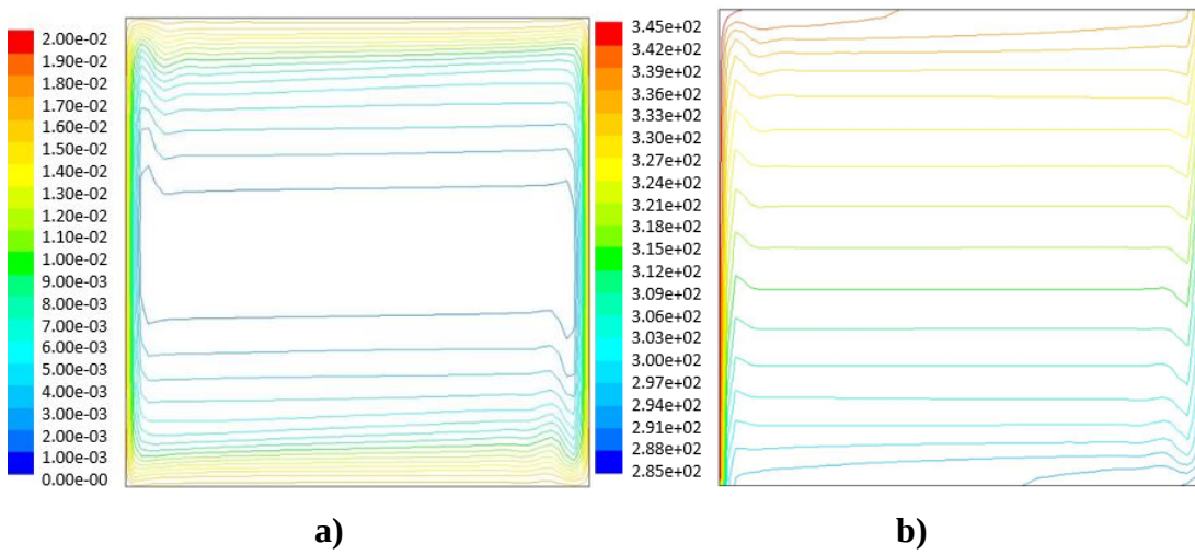
Şekil 4.22 : Ra = 1,61 \times 10^8 'de CuO – Su nanoakışkanı için a) akım çizgileri b) eş sıcaklık eğrileri.
