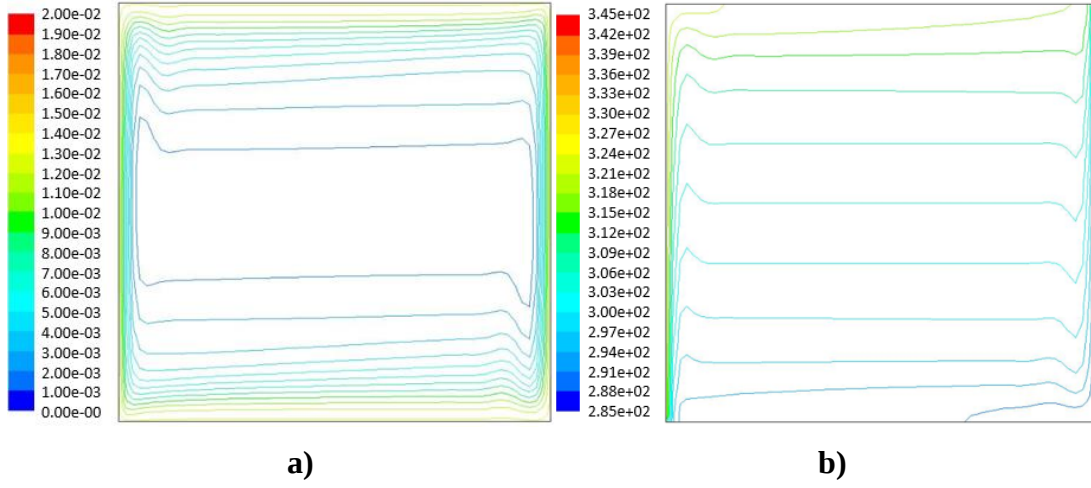
Şekil 4.20 : Ra = 4,8 \times 10^7 'de CuO – Su nanoakışkanı için a) akım çizgileri b) eş sıcaklık eğrileri.
