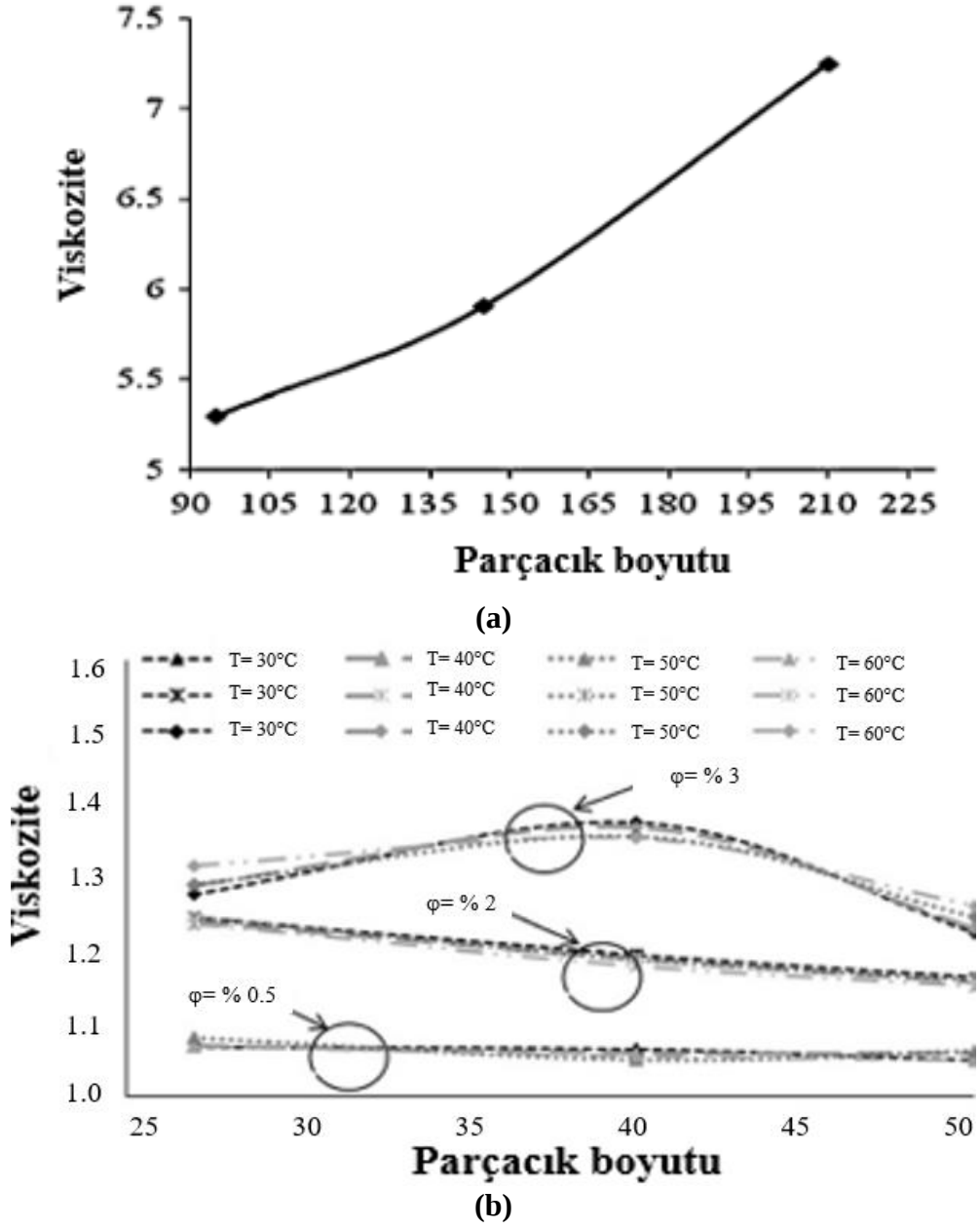
Şekil 3.13: Parçacık boyutunun viskozite üzerindeki etkisi (a) (He 2007)'nin sonuçları, (b) (Prasher ve diğ. 2006)'ın sonuçları.
