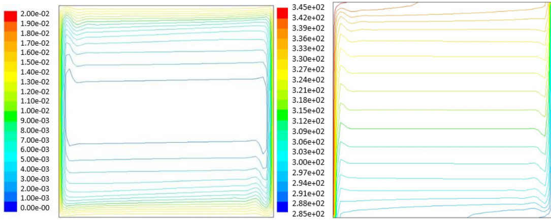
Şekil 4.12: CuO – Su, \phi = \% 2 için a) akım çizgileri b) eş sıcaklık eğrileri.
