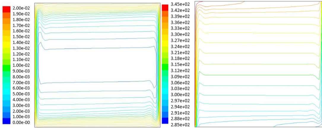
Şekil 4.13: CuO – Su, \phi = \% 5 için a) akım çizgileri b) eş sıcaklık eğrileri.
