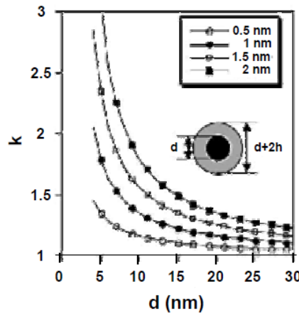
Şekil 3.5: Arayüz boyutunun ısı iletkenlik üzerindeki etkisi (Kebllinski ve diğ. 2004).
