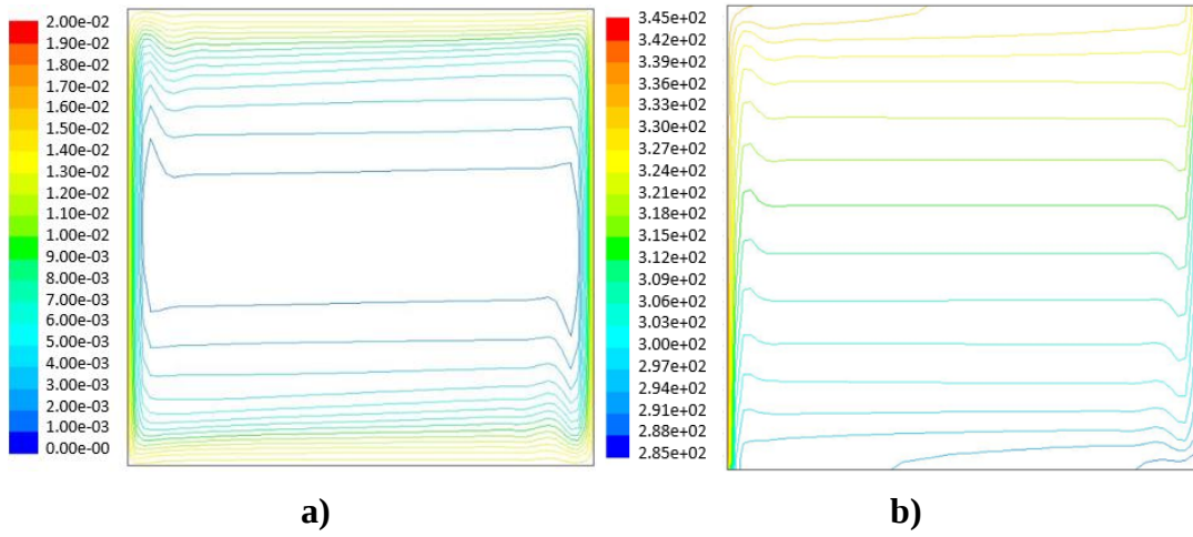
Şekil 4.21 : Ra = 9,8 \times 10^7 'de CuO – Su nanoakışkanı için a) akım çizgileri b) eş sıcaklık eğrileri.
