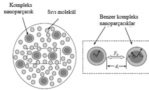
Şekil 3.1: Nanoakışkanlarda Brownian Hareketi (Murshed ve Nieto 2011).
