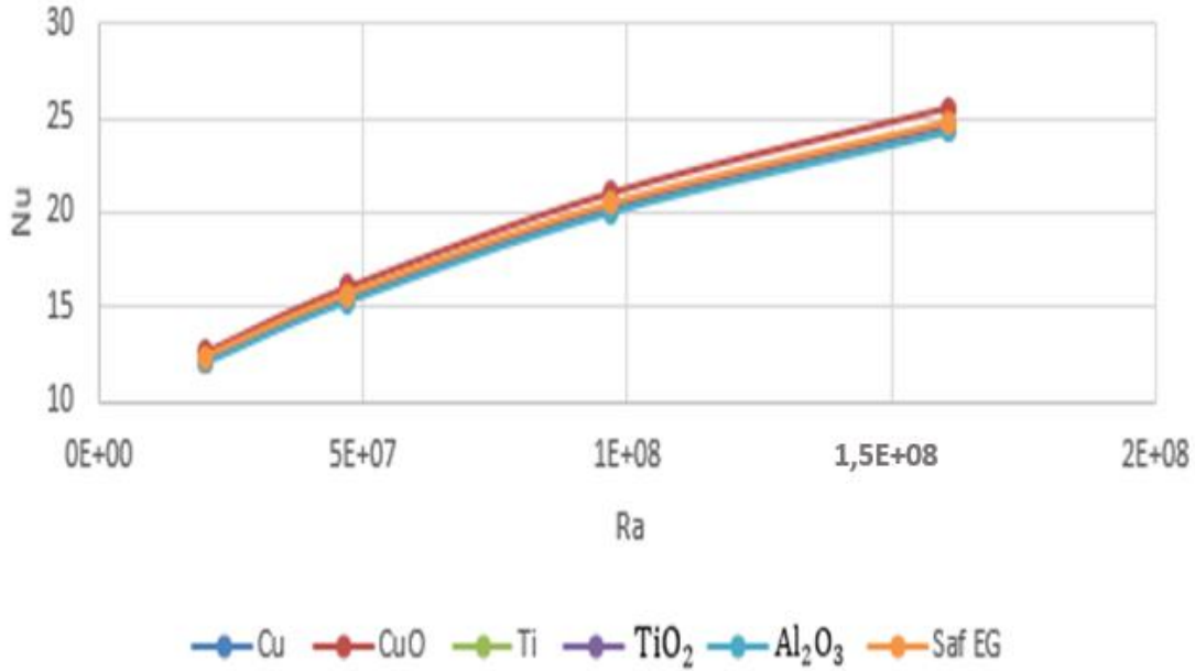
Şekil 4.27: Tüm Etilen Glikol bazlı nanoakışkanların % 7,5 hacim oranında Rayleigh sayısının değişiminin Nusselt sayısı üzerindeki etkisi.
