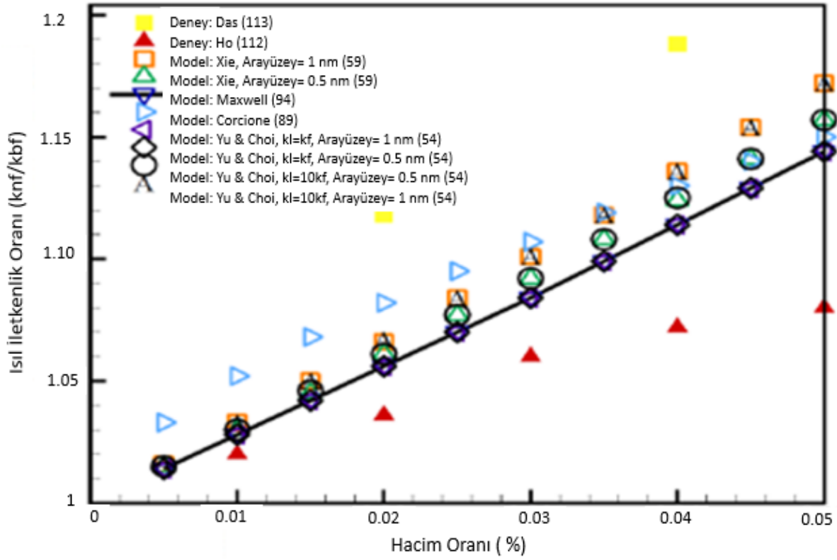
Şekil 3.12: CuO-Su için farklı ısı iletim modellerinin karşılaştırılması (Aybar ve diğ. 2015).
