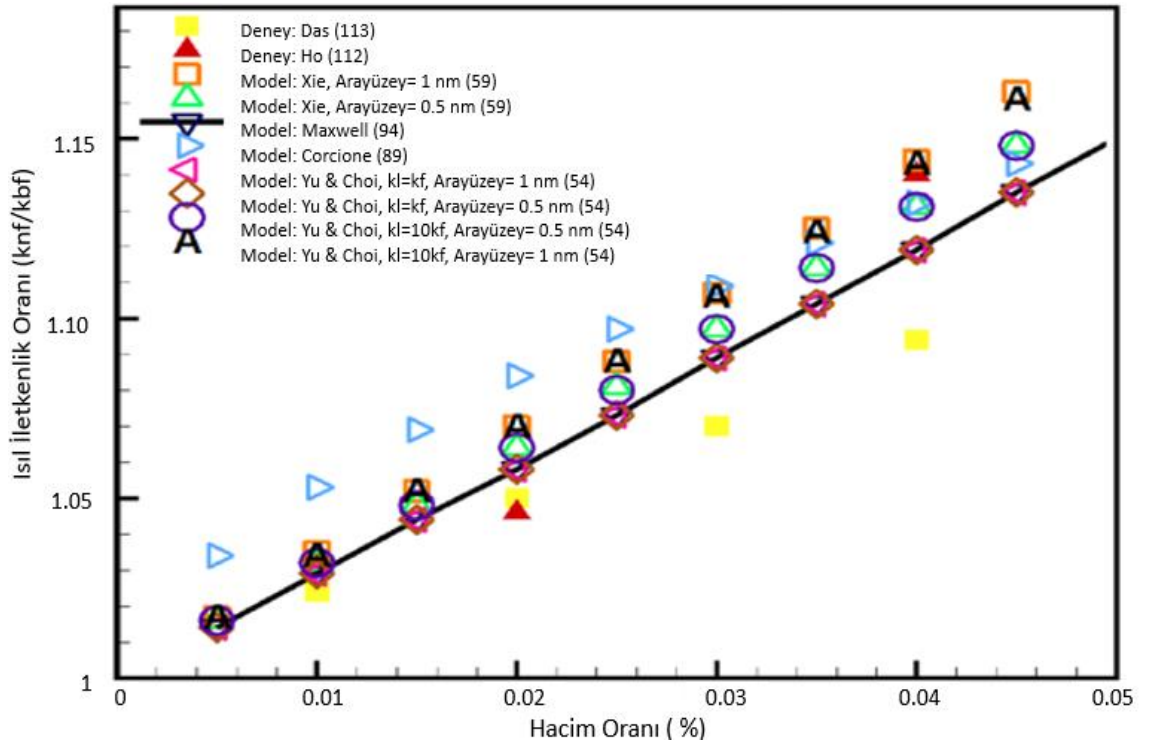
Şekil 3.11: Al_2O_3 -Su için farklı ısı iletim modellerinin karşılaştırılması (Aybar ve diğ. 2015).
