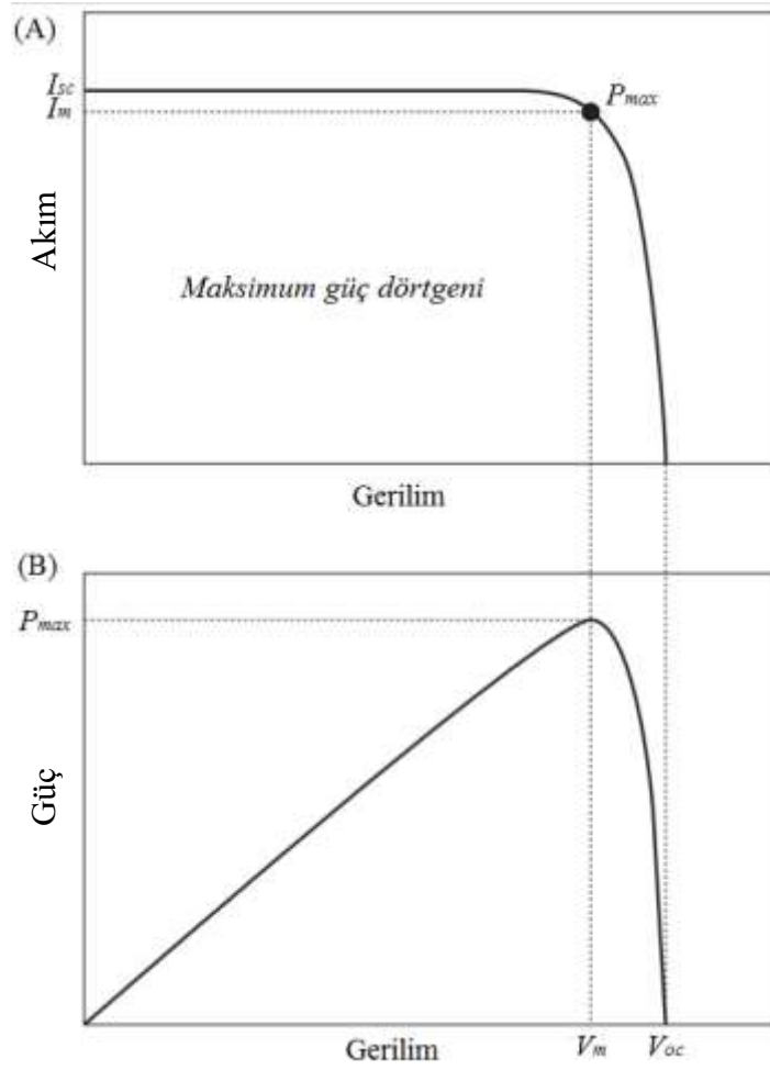
Şekil 2.8 : Güneş hücresinin akım-gerilim (I-V) ve güç-gerilim (P-V) eğrileri [43].
