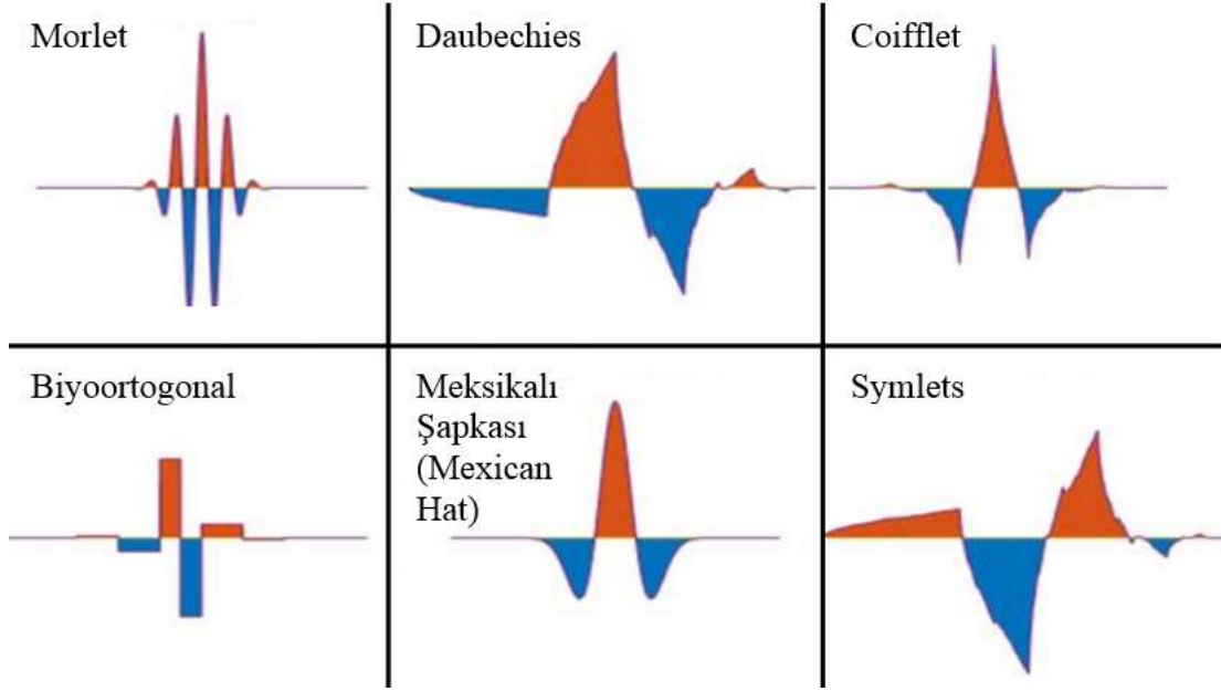
Şekil 5.2 : Bazı dalgacık ailelerinden sıklıkla kullanılan dalgacıklar.
