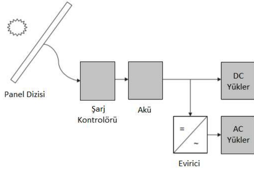
Şekil 3.3 : Doğru akım ve alternatif akımla çalışan yüklerin bulunduğu şebekeden bağımsız fotovoltaik sistem şeması [39].
