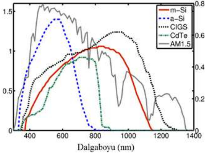
Şekil 4.2 : Solar radyasyon ve güneş hücrelerinin soğurma spectrumları[78].
