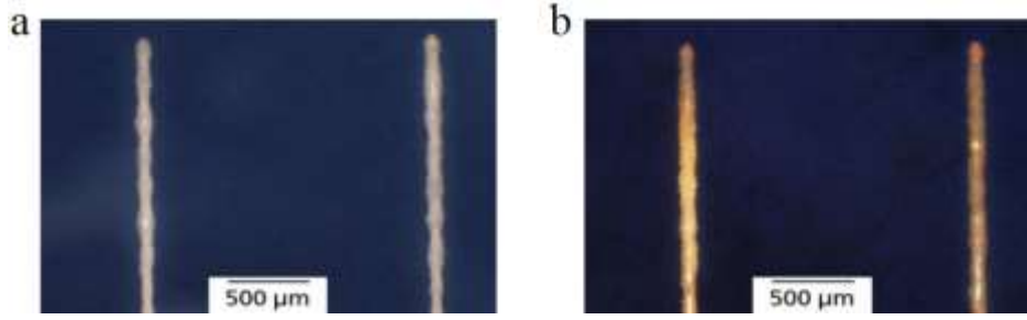
Şekil 4.5 : Kontakları salyangoz izine karşı dayanıklı malzemeden (a) ve salyangoz izine karşı hassas malzemeden (b) yapılmış hücrelerin mikroskopik görünümü [64].
