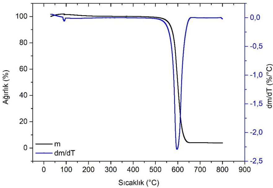
Şekil 6.3 : F-MWCNT’lerin termogravimetrik analizi.
