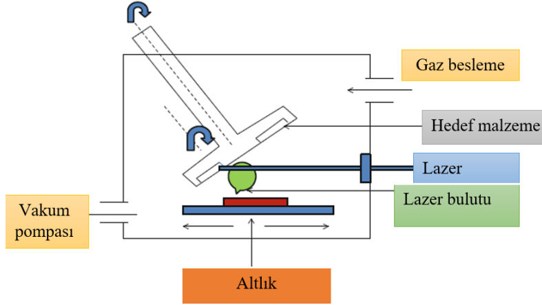
Şekil 2.5 : Darbeli lazer biriktirme prosesi [38].
