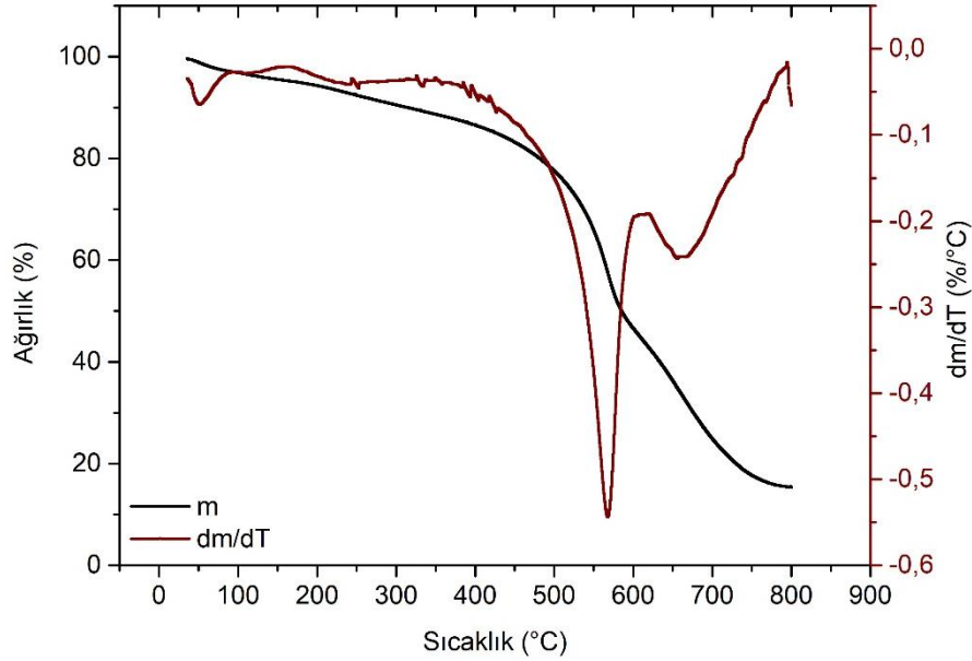
Şekil 6.5 : F-SWCNT'lerin termogravimetrik analizi.
