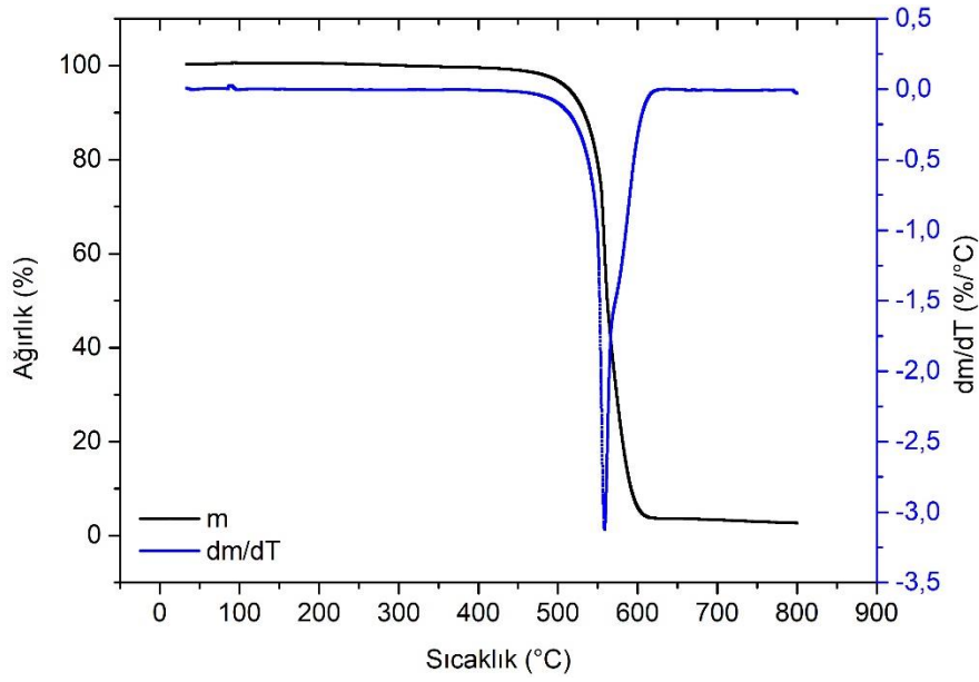
Şekil 6.2 : MWCNT’lerin termogravimetrik analizi.
