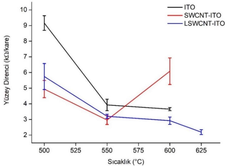
Şekil 6.17 : ITO, SWCNT-ITO ve LSWCNT-ITO ince filmlerin sıcaklığa bağlı yüzey direnci değişimi.
