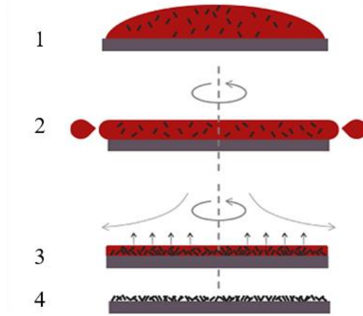
Şekil 2.10 : Dönel kaplama işlemi [50].
