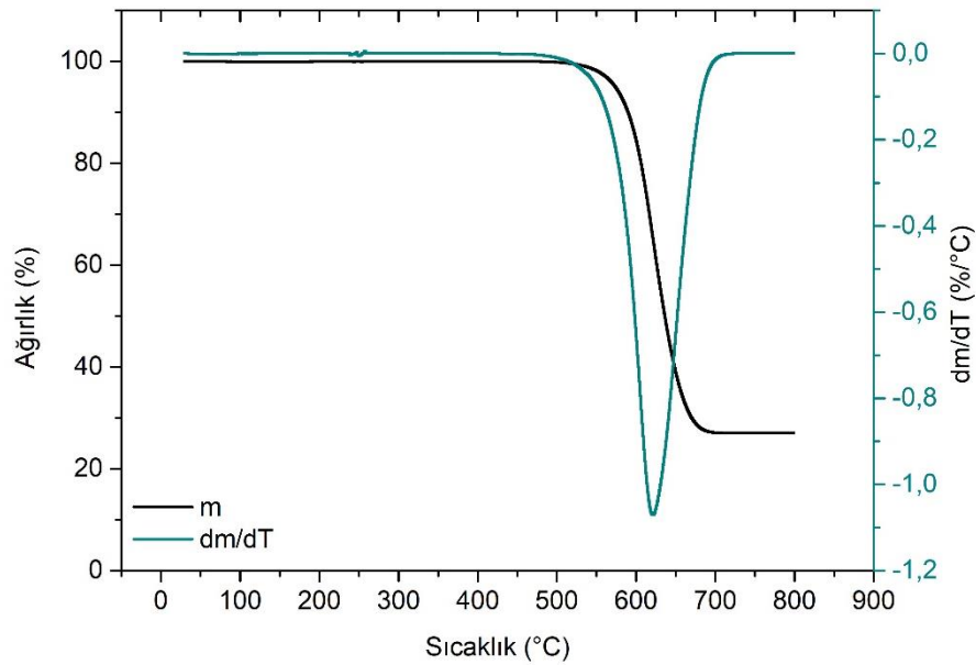
Şekil 6.6 : LSWCNT'lerin termogravimetrik analizi.
