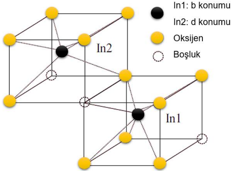
Şekil 2.1 : In_2O_3 'ün kristal yapısı [17].
