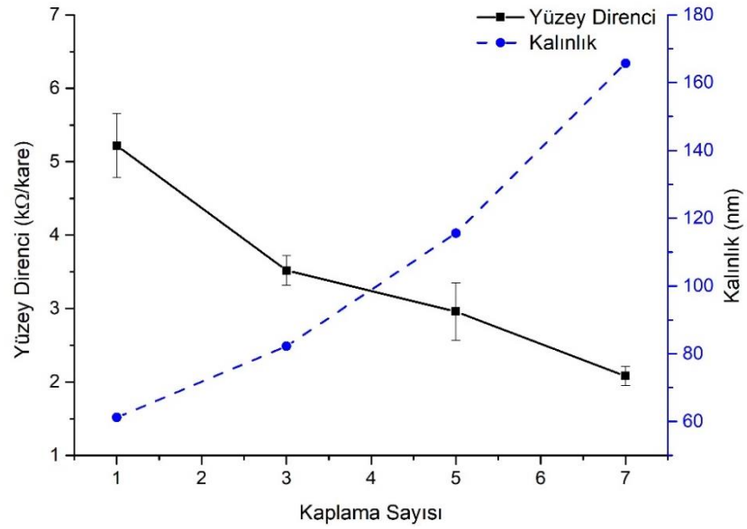
Şekil 6.9 : ITO filmlerin kalınlık ve yüzey direnci değişimi.
