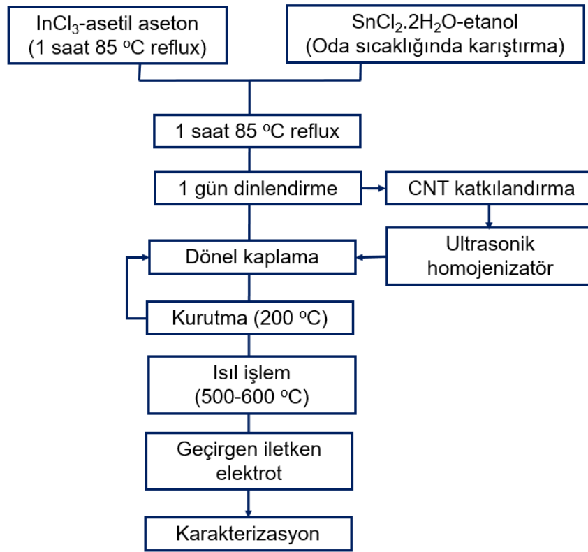
Şekil 5.1 : ITO ve CNT-ITO hibrit elektrot üretimi akış şeması.
