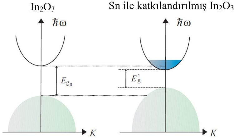
Şekil 2.3 : Sn katkılandırmanın In 2 O 3 bant aralığına etkisi [17].
