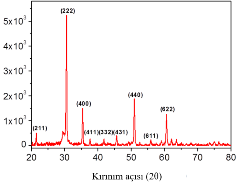
Şekil 2.12 : 600 °C’de ısıtıl işlem görmüş ITO ince filmin XRD deseni [56].
