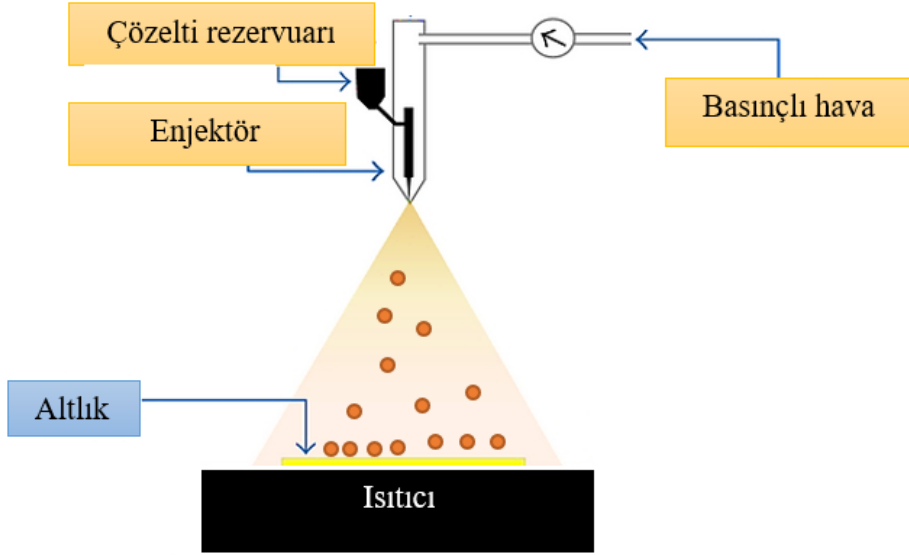
Şekil 2.9 : Spreyci kaplama ile ince film oluşumu.
