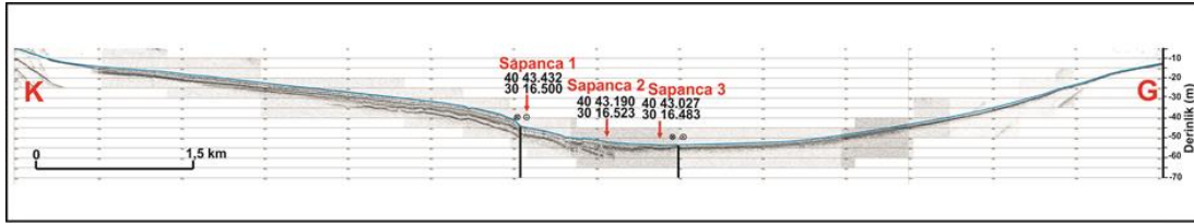
Şekil 1.2: Sapanca gölünden alınan karotların sismik kesit üzerindeki yerleri ve koordinatları
