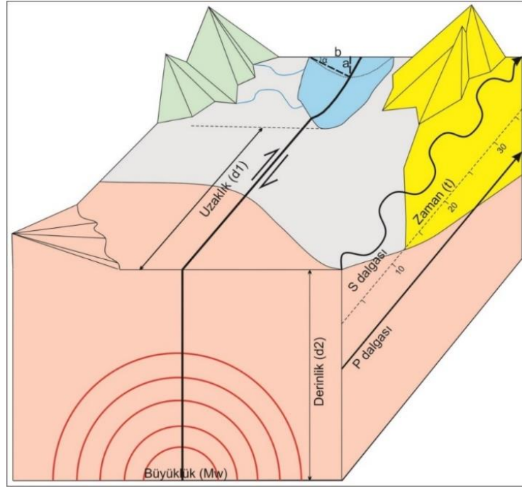
Şekil 4.11: Sismo-türbiditlerin kalınlığını etkileyen deprem parametrelerinin (depremin büyüklüğü, deprem merkezinin depolanma alanına uzaklığı, depremin derinliği, gölün geometrisi) blok diyagramda gösterimi.
