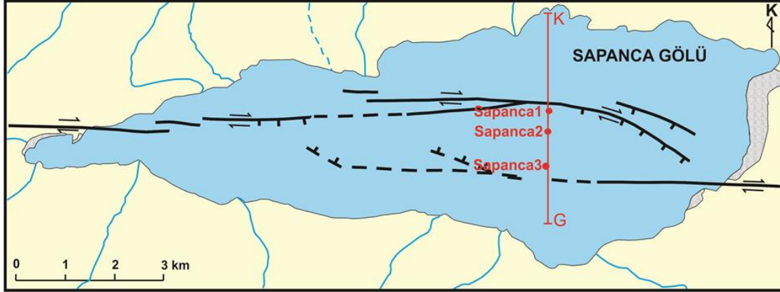
Şekil 1.1: Sapanca gölünden geçen Kuzey Anadolu Fayının ve gölden alınan karotların yer bulduru haritası (TUJJB-UDP-03-10).
