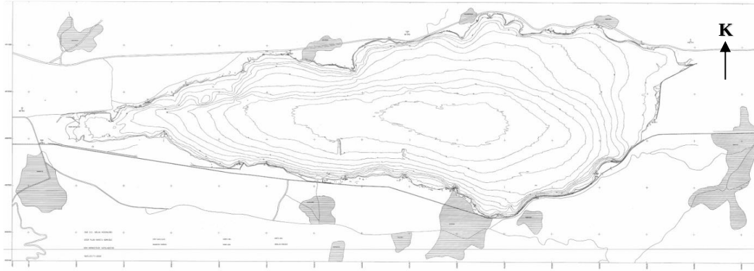
Şekil 1.3: Devlet Su İşleri tarafından 2002 yılında yapılan Sapanca Gölünün derinlik haritası
