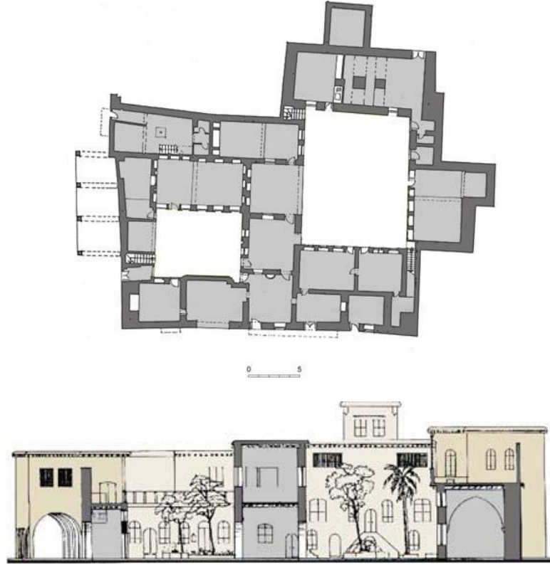
Şekil 4.8 : İç avlulu kentsel alan konutu plan ve cephe çizimleri (Fakouch, 2004).
