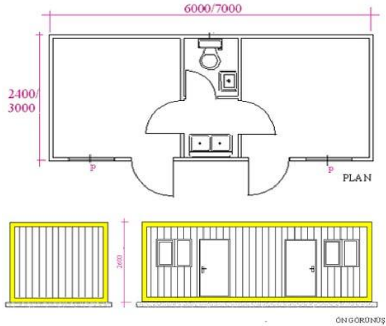
Şekil 5.3: Tipik konteyner boyutları (Url-17).
