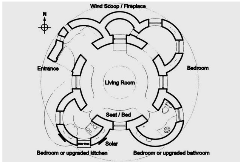
Şekil 3.4: Sandbag barınağı plan şeması (2004 Review Report,2004).
