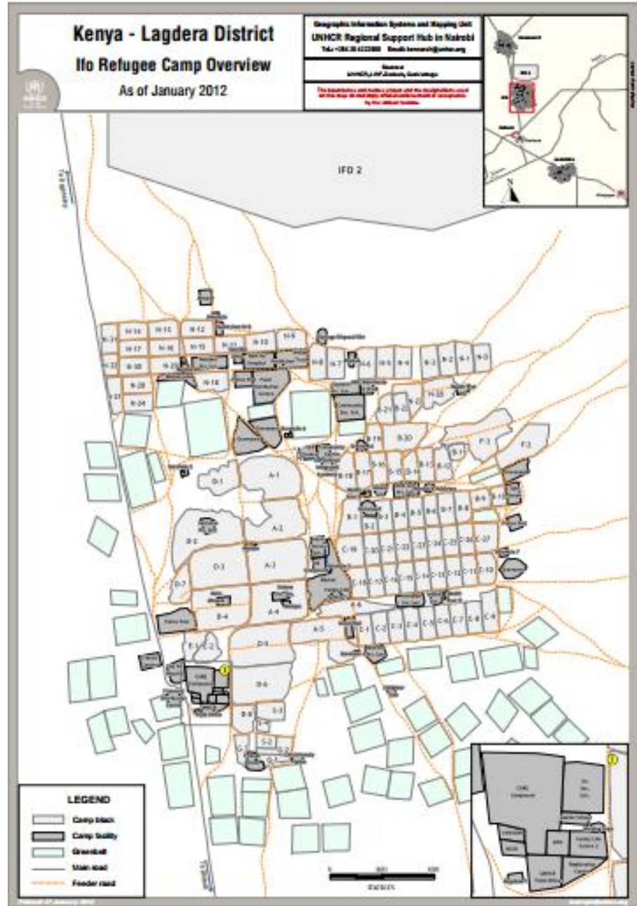
Şekil 3.11: Ifo kampı vaziyet planı (UNHRC,2012).
