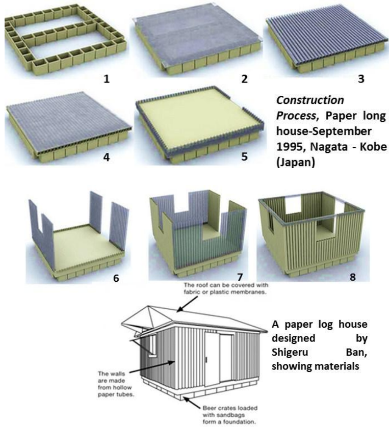
Şekil 3.9: Kağıt tüp konutunun üretim aşamaları. (Safaei, 2012)
