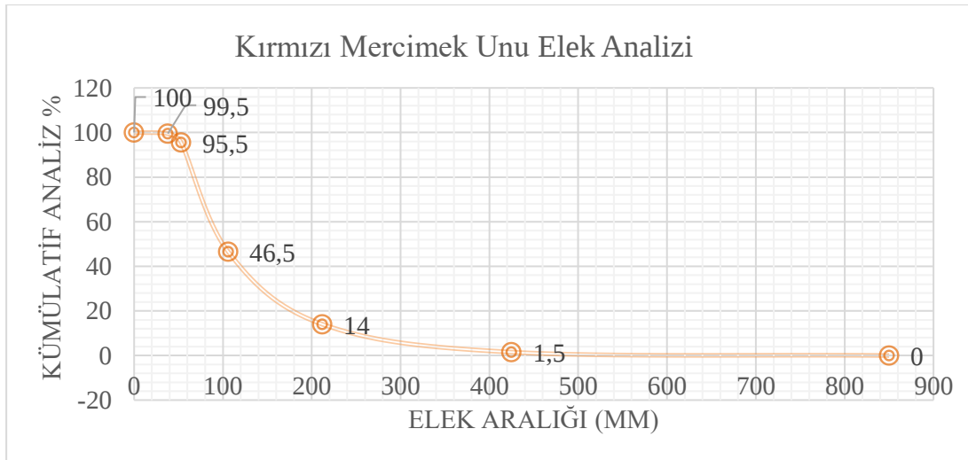
Şekil 4.1: Öğütülmüş kırmızı mercimek için boyut dağılım grafiği.
