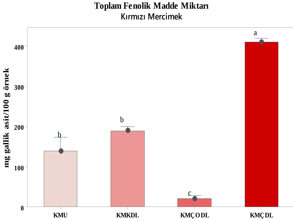
Şekil 4.8 : Kırmızı mercimek grubu örneklerin fenolik madde miktarları.
