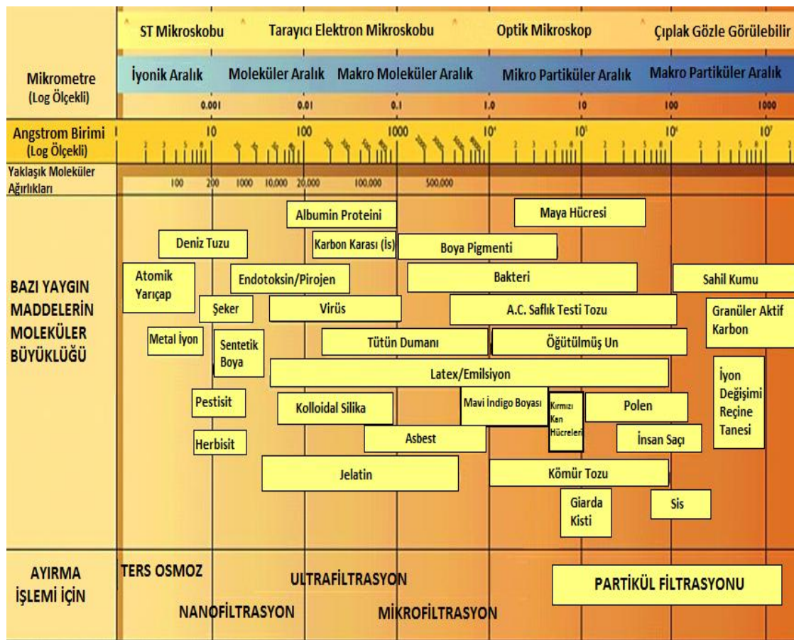
Şekil 2.2. Membran filtrasyon spektrumu (Osmonics Inc, 1996).
