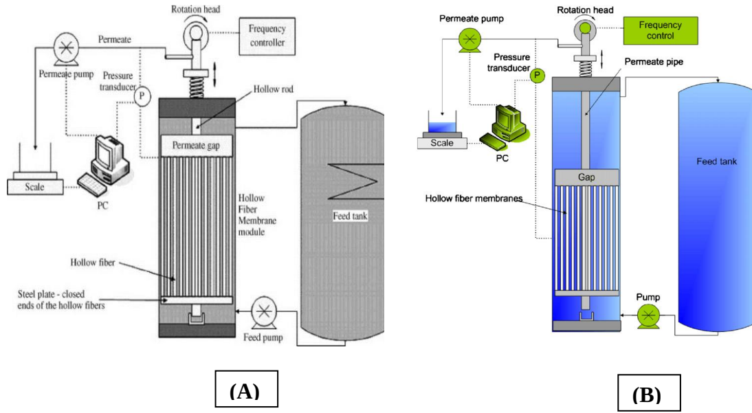
Şekil 2.14. Beier et al tarafından kullanılan titreşimli sistemin şematik çizimi (A eski versiyon, B yeni versiyon).
