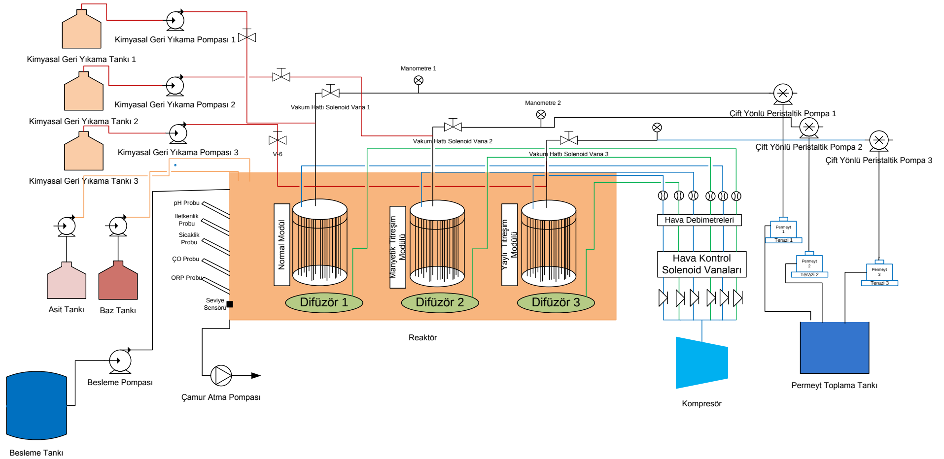
Şekil 3.1 : Laboratuvar ölçekli MBR sisteminin akım şeması
