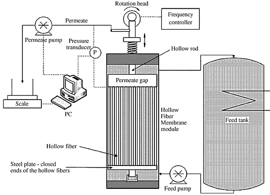
Şekil 2.35. Deney amaçlı kullanılan bir titreşim sistemli batık MBR düzeneği şeması (Beier ve diğ., 2006).
