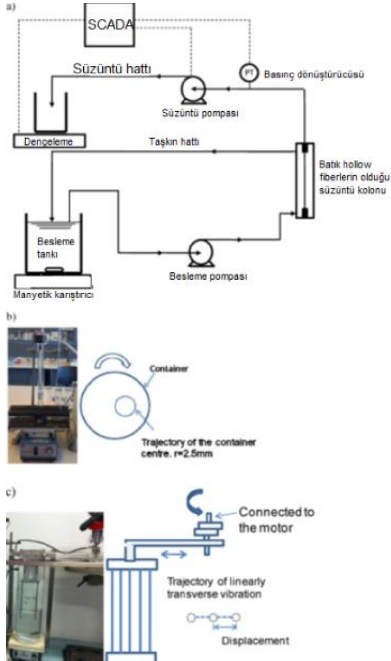
Şekil 2.19. Anusha Kola tarafından kullanılan enine titreşim sisteminin şematik gösterimi (Kola ve diğ., 2014).
