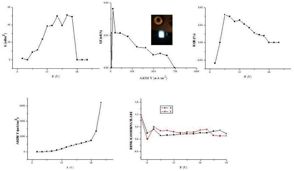
Şekil 4.10 : OLED1. PEDOT/P1/TPBi/LiF/Al.
