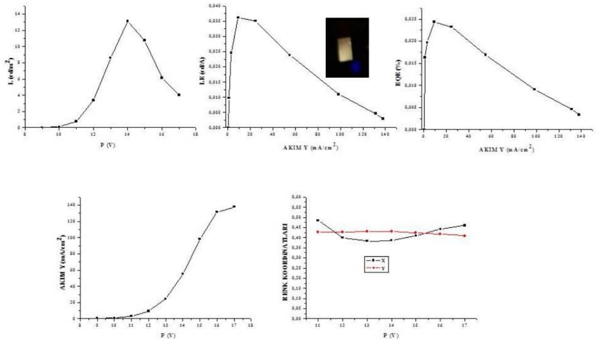
Şekil 4.11 : OLED2. PEDOT/P2/TPBi/LiF/Al.
