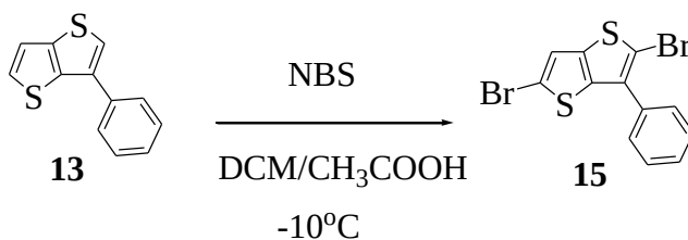
Şekil 3.14 : (PhTTBr 2 ) (15) sentezi.
