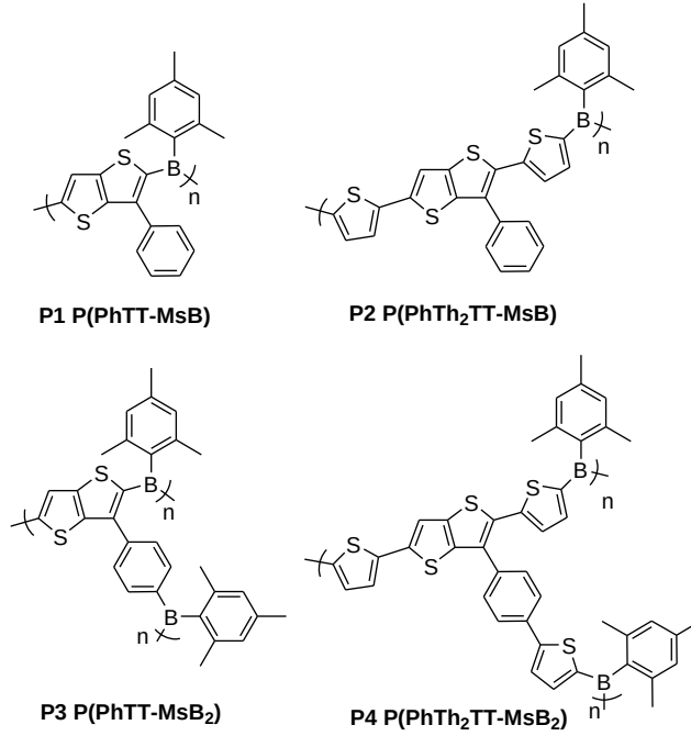
Şekil 4.2 : Donör-akseptör polimerler.
