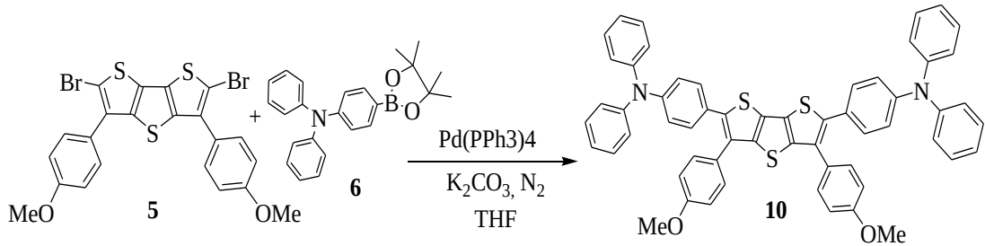
Şekil 4.15 : DTT-TPA kenetlenme sonuç ürünü.
