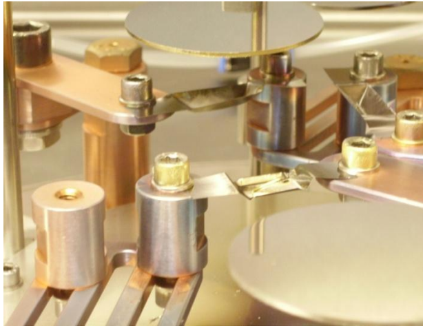
Şekil 3.28 : Metal katmanın kaplanması.
