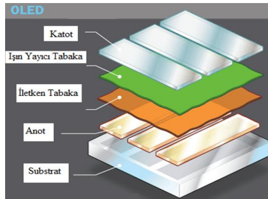
Şekil 2.17 : OLED tabaka gösterimi.
