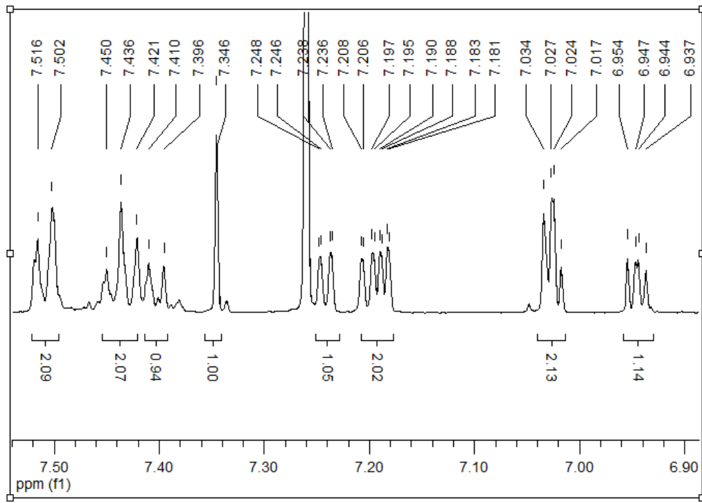
Şekil A.9 : PhTTTh2 için 1 H-NMR spektrumu.
