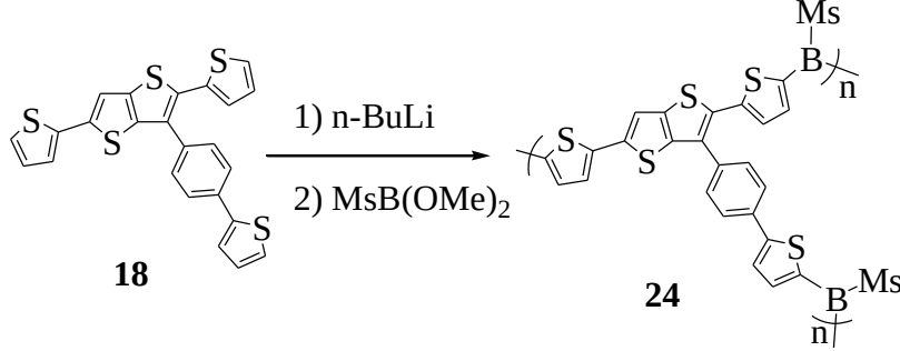
Şekil 3.25 : P(PhTh 2 TT-MsB 2 ) sentezi.
