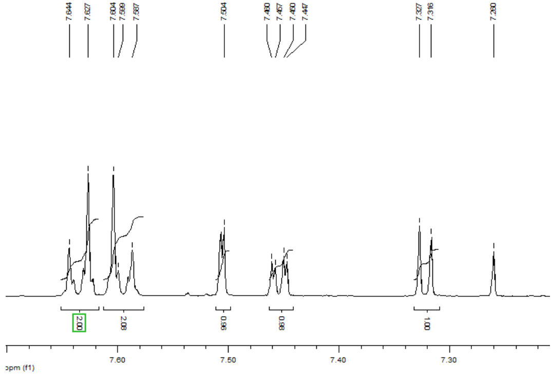
Şekil A.15 : BrPhTT için 1 H-NMR spektrumu.
