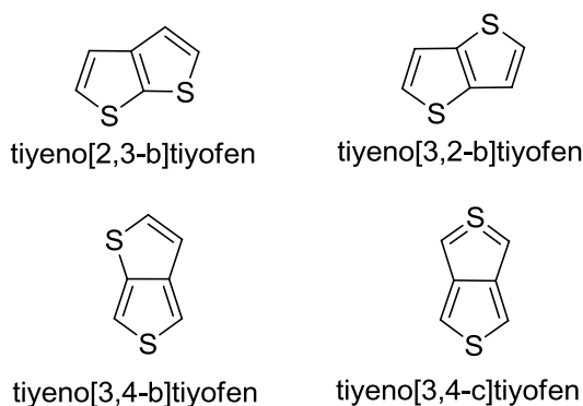
Şekil 2.15 : Tiyenotiyofen izomerleri.
