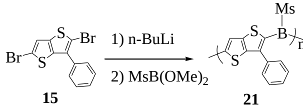
Şekil 3.22 : P(PhTT-MsB) sentezi.
