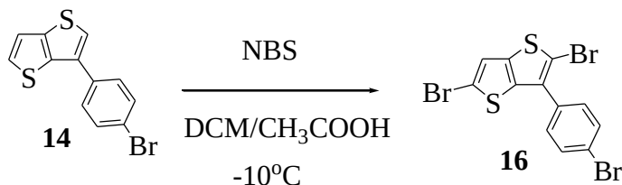
Şekil 3.15 : (PhTTBr 3 ) ( 16 ) sentezi.
