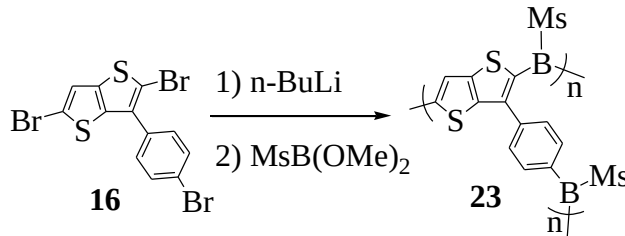
Şekil 3.24 : P(PhTT-MsB 2 ) sentezi.
