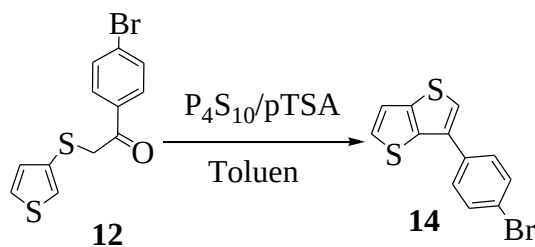
Şekil 3.13 : 3-(4-Bromofenil)tiyeno[3,2- b ]tiyofen (14) sentezi.
