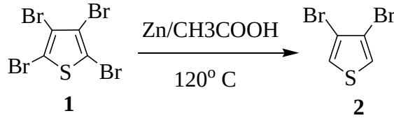
Şekil 3.2 : 3,4-Dibromtiyofen sentezi.
