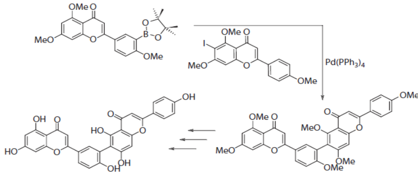
Şekil 2.6 : Robustaflavon sentezi.
