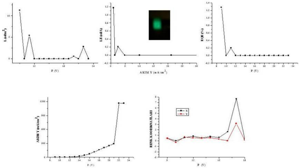
Şekil 4.13 : OLED4. PEDOT/P4/TPBi/LiF/Al.
