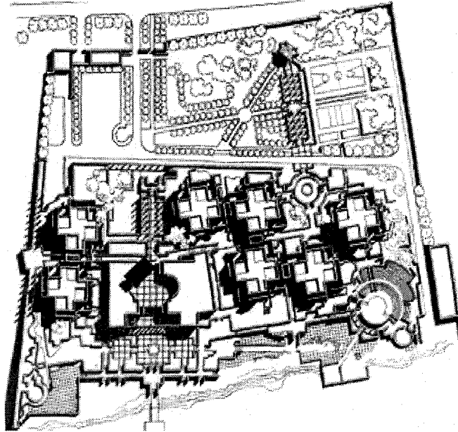
Şekil 3.11: Konut yerleşim projesi 1970, Aşkabat.
