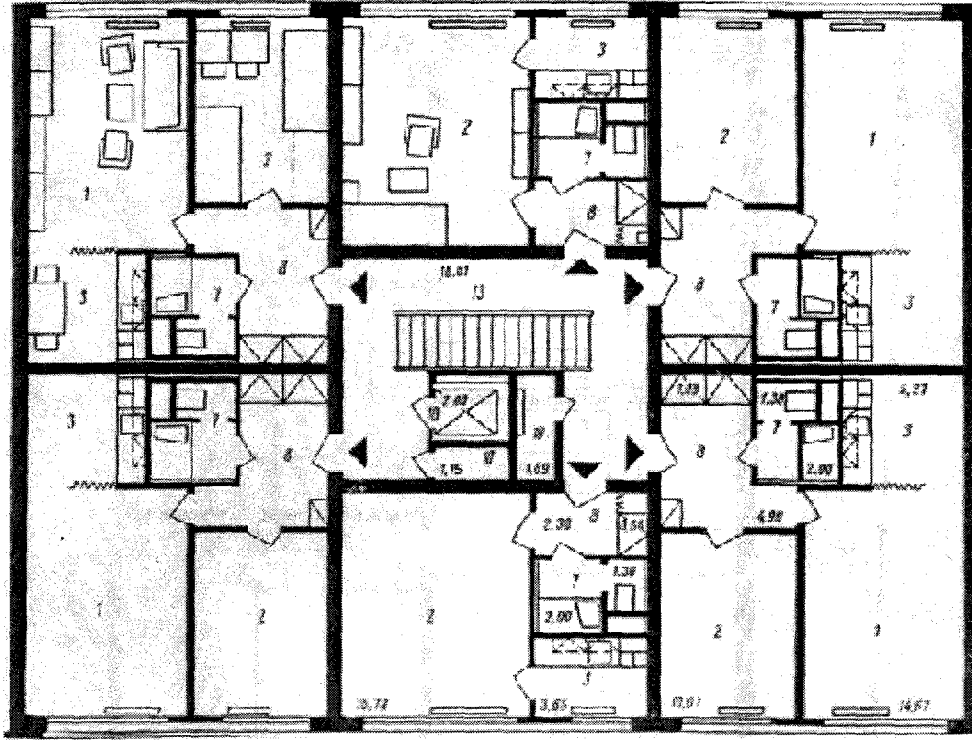
İki odalı konut tipi, 39 M2
