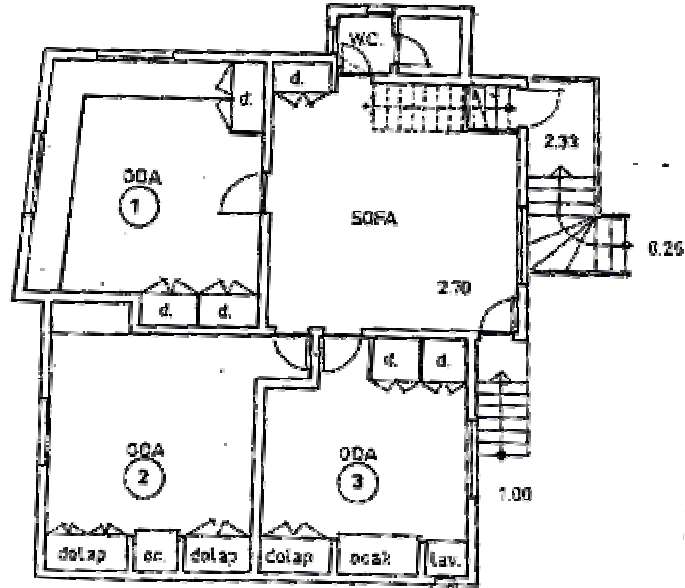
ARA KAT PLANI
