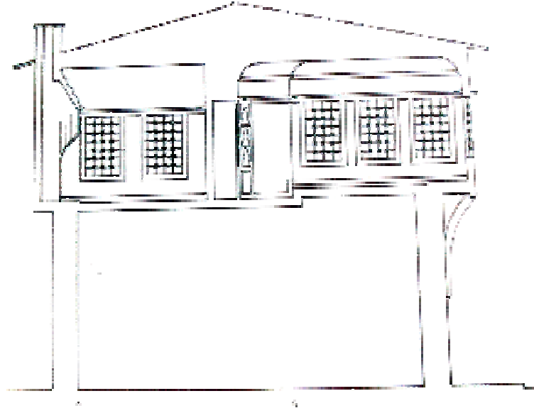
Şekil3.3: İki katlı bir Türk Evi'ne ait bir kesit. (Eldem, 1972).
