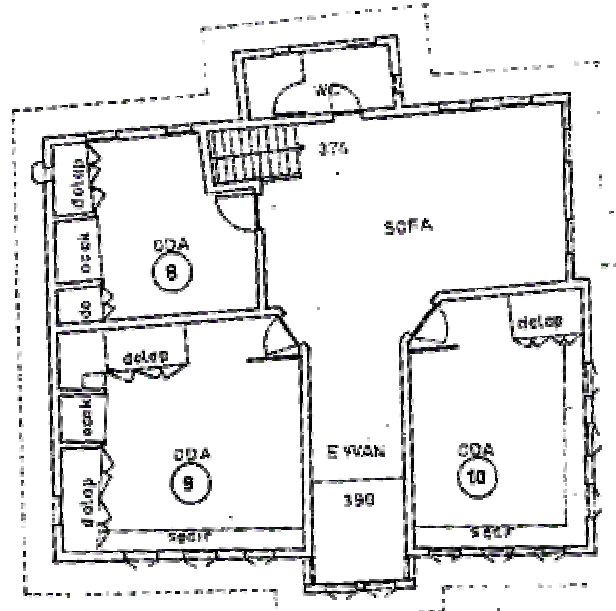
ÜST KAT PLANI
