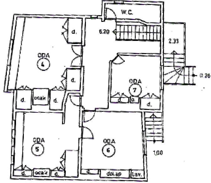
ÜST KAT PLANI
