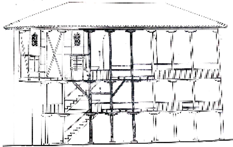
Şekil3.4: Üç katlı bir Türk Evi'ne ait bir kesit. (Eldem, 1972).
