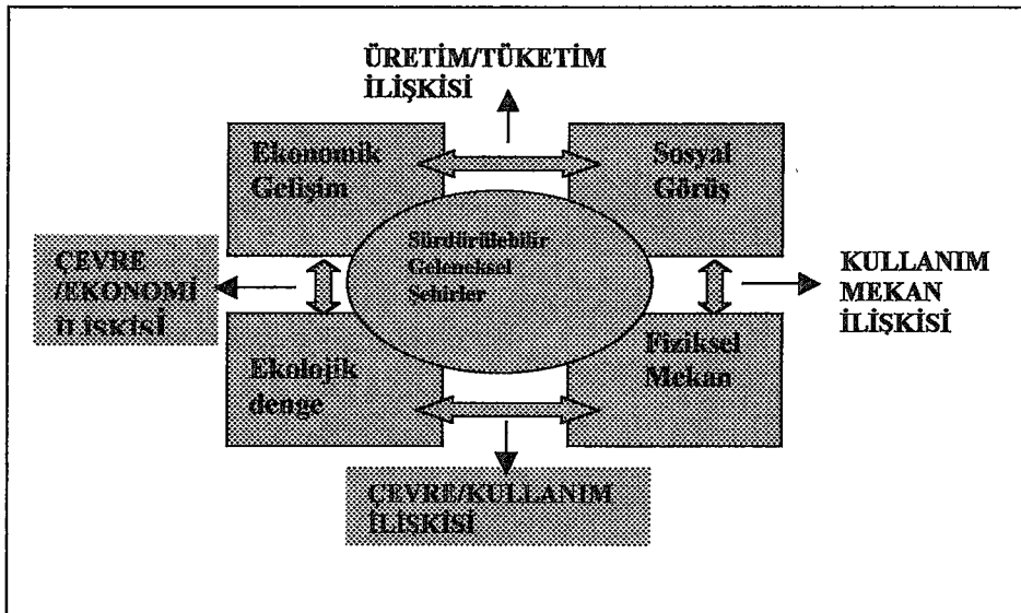
Şekil 2.16 Şehirsel Tasarım kuramında kullanılabilecek bir sürdürülebilirlik modeli (H.Uğur.)
