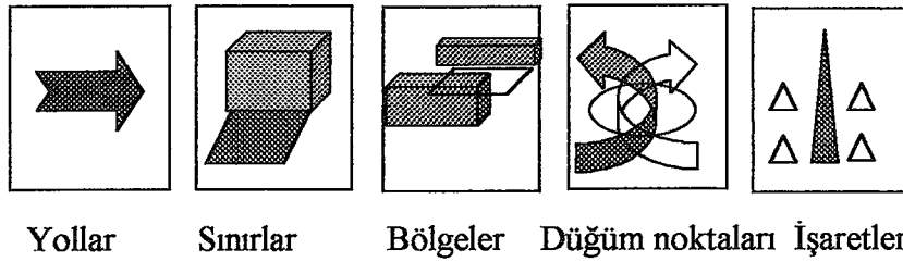
Şekil 2.8 Şehirselle mekan ölçeğinde doku öğeleri (Lynch, 1960)
