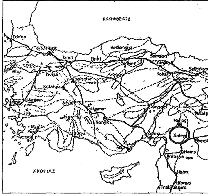
Şekil 3.17 Gaziantep ve Osmanlı ilk dönemi ticaret yolları
