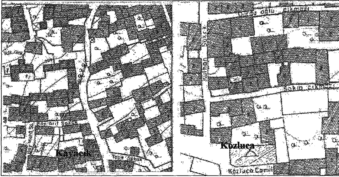
Şekil 3.24 Farklı kültürlere ait (Kayacık-Ermeni, Kozluca-Müslüman) iki mahallenin morfolojik yapısı.
