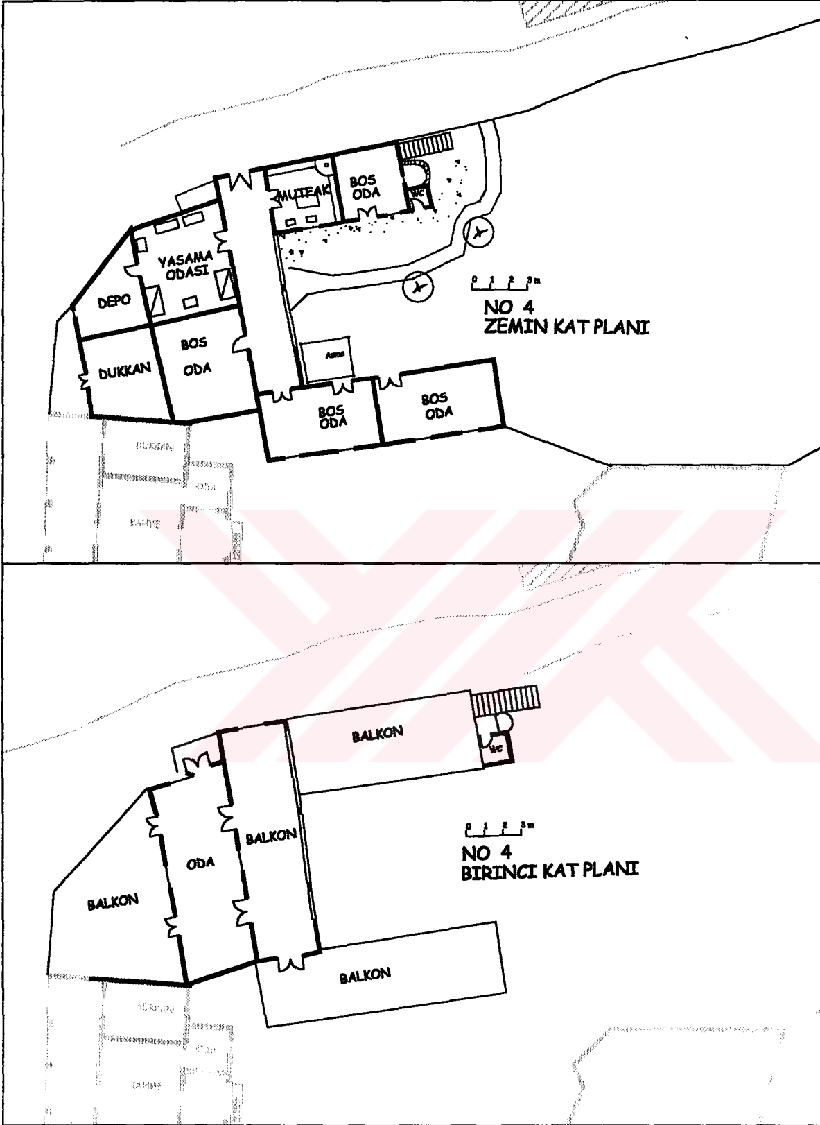
Şekil 5.14. No 4 Konutu Planı.
