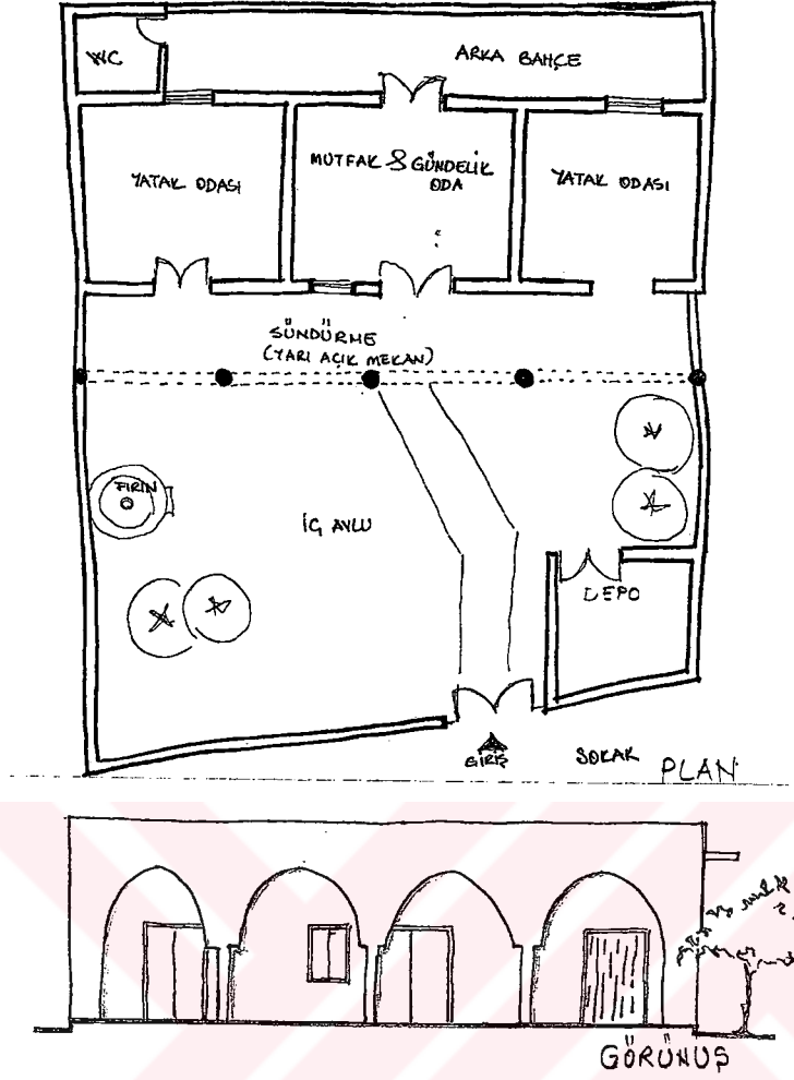
Şekil 4.5. Önde yarı açık mekanı bulunan konut örneği (Tozan, A., 1998).
